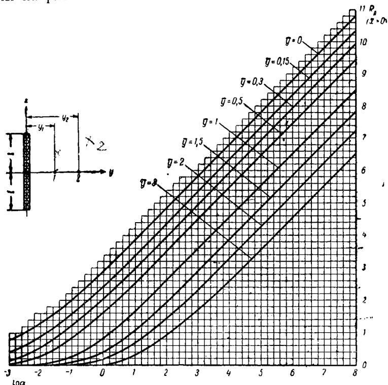
Рис. 2. График функции R_{л|x=0}(\alpha; \bar{y})
