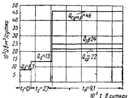
Рис. 22. График режима эксплуатации водозаборов к примеру № 4
