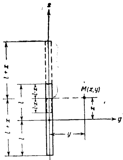
Рис. 4. Схема к расчету R_{л|\bar{x}, \bar{y}} в любой точке пласта с координатами x, y
