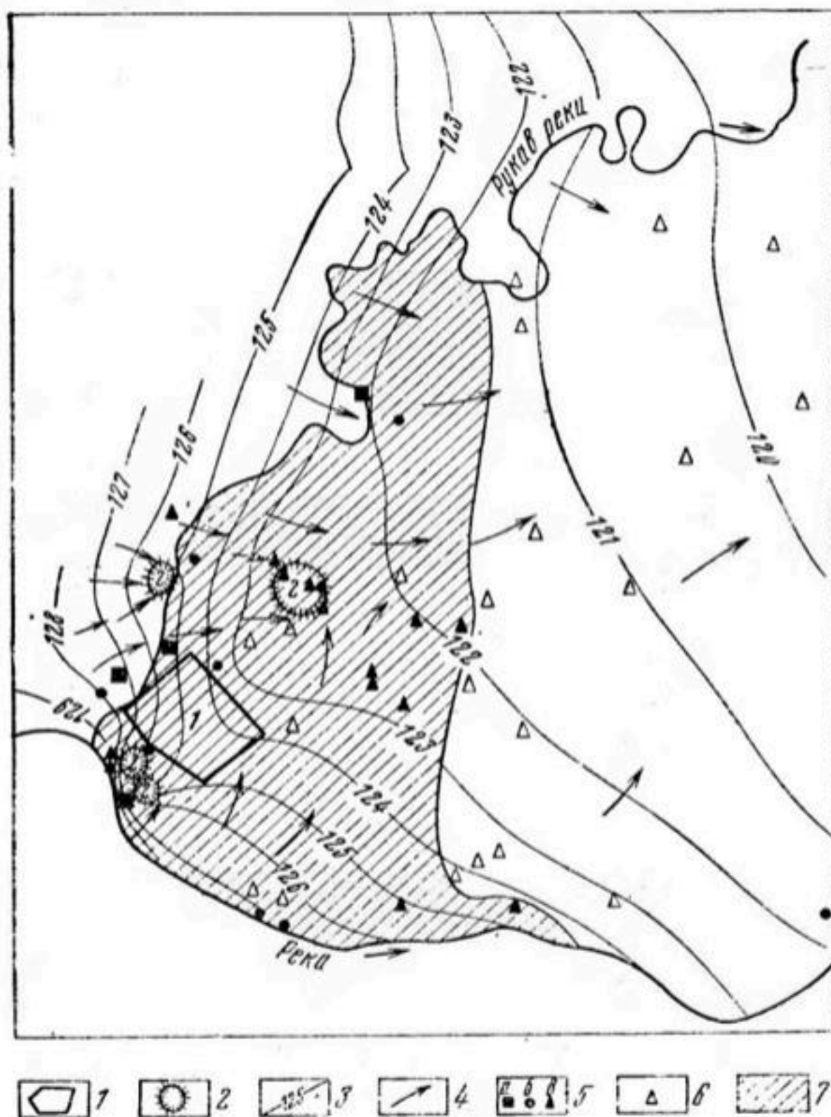
Рис. 76. Загрязнение подземных вод нефтепродуктами:
