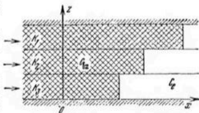
Рис. 6. Концентрационные языки загрязненных вод в слоистом пласте:
