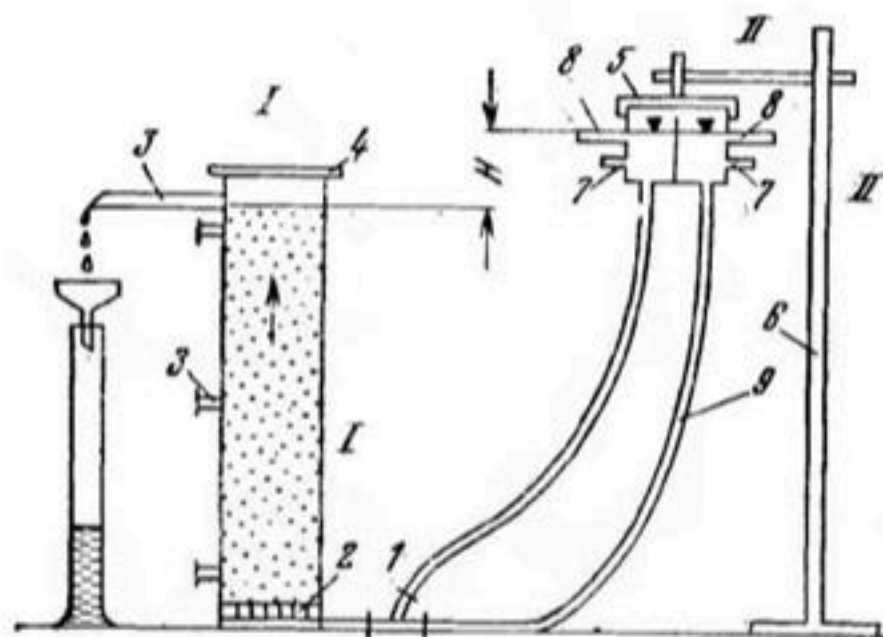
Рис. 64. Схема лабораторной установки для изучения фильтрационной дисперсии:
