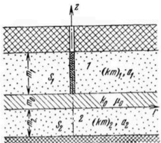
Рис. 28. Схема трехслойного пласта: 1, 2 — номера слоев
