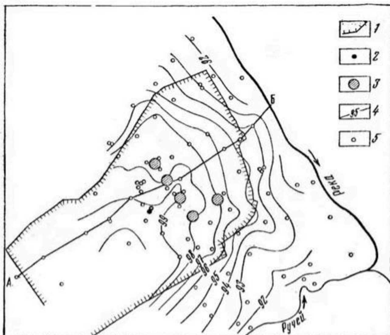
Рис. 71. Схематическая карта гидронизогипс в районе сажевого завода:
