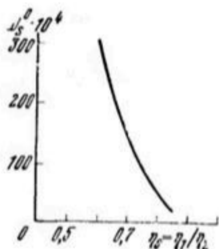
Рис. 4. Зависимость D_s^0 от \eta_0 = \eta_1/\eta_2 (по [66])
