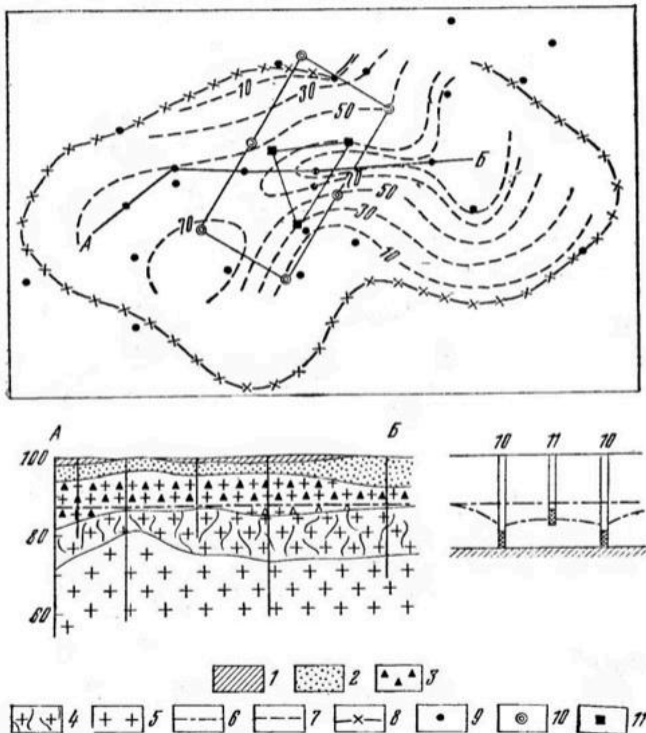
Рис. 74. Загрязнение трещинно-пластовых вод нефтепродуктами:
