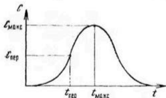
Рис. 68. График C(t) в наблюдательной скважине при запуске индикаторного «намета»
