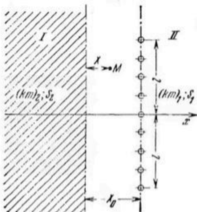
Рис. 25. Схема к расчету линейного ряда скважин в неоднородном пласте с прямой границей раздела: I, II — зоны с различной водопроницаемостью и пьезопроводностью
