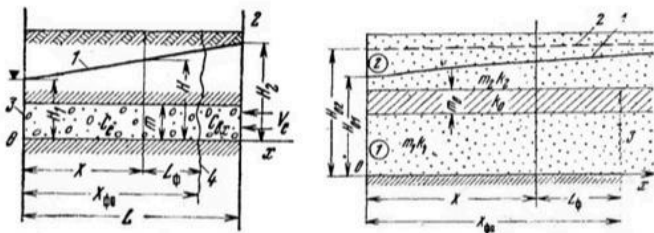
Рис. 44. Схема к расчету фронта загрязнений в одномерном потоке подземных вод (пласт, изолированный водоупорными кровлей и подошвой):
