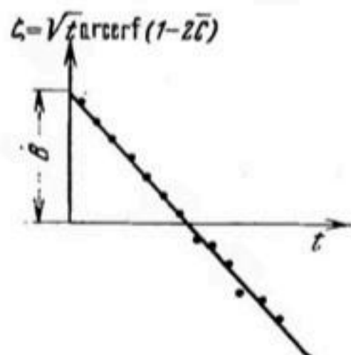
Рис. 65. График зависимости \xi(t)
