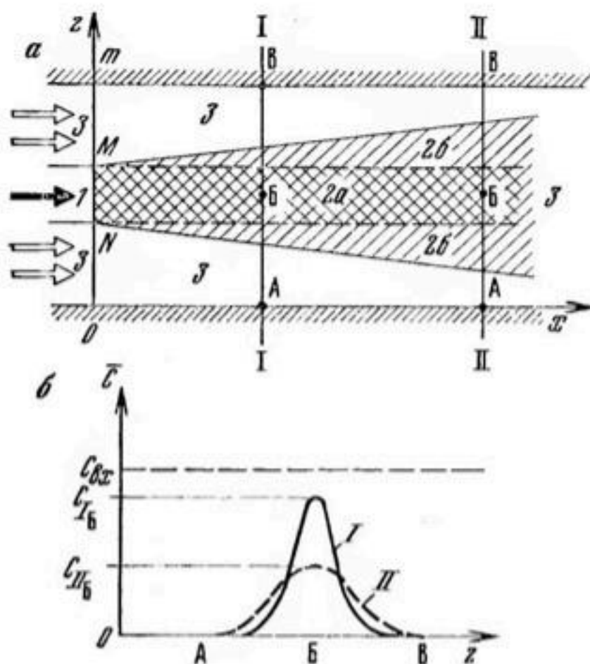
Рис. 3. Поперечная и продольная микродисперсия: a — схема пласта; b — график C(z) . I — загрязненные воды; 2a — зона продольной микродисперсии; 2b — зона поперечной микродисперсии; 3 — чистые воды; I, II — сечения пласта
