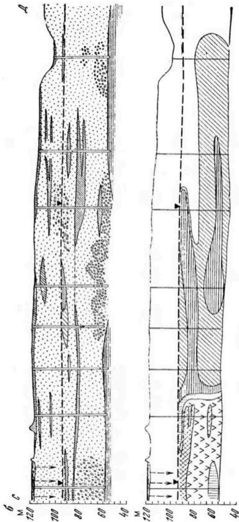
Рис. 81. Гидрогеологические и гидрохимические разрезы по линиям А-В (а) и СД (б).
