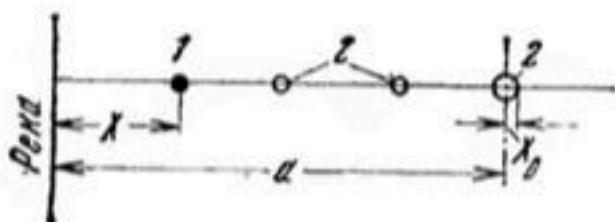
Рис. 69. Схема расположения скважин при запуске индикатора и наблюдательную скважину при откачке вблизи реки:
