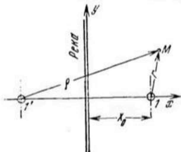
Рис. 16. Схема к расчету скважины у совершенной реки:
