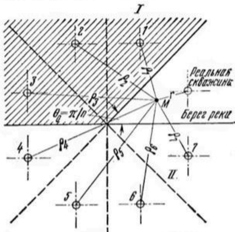
Рис. 20. Скважина в неоднородном пласте с прямолинейной границей раздела, не параллельной урезу реки.
