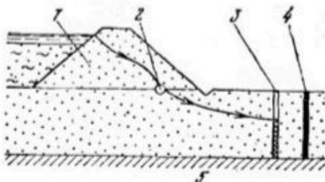
Рис. 54. Перехватывающий дренаж в нижнем бьефе шламохранилища:
