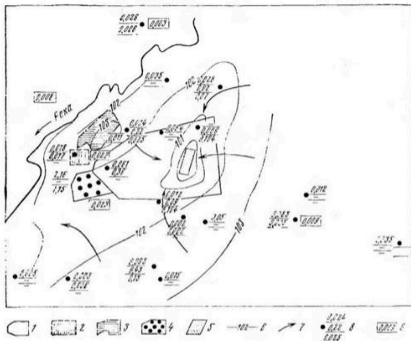
Рис. 77. Загрязнение подземных вод в районе металлургического завода:
