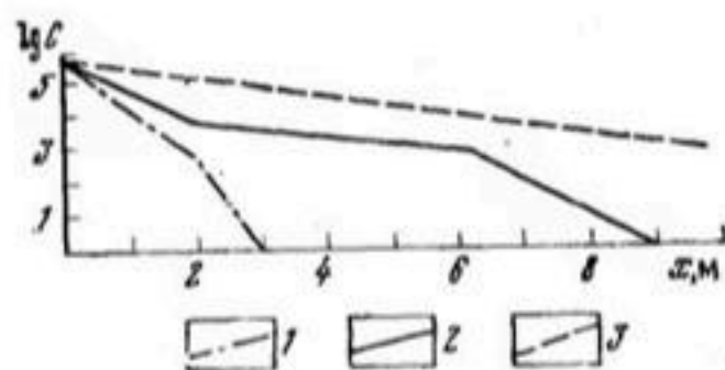
Рис. 12. Дальность распространения микроорганизмов за 60 суток при фильтрации в песках бактериально загрязненной воды со скоростью 1,5 м/сут. (Эффективный диаметр частиц песка 0,2 \text{ мм} < d_{эф} < 0,5 \text{ мм} ): C — количество микробных тел в 1 л воды; x — путь фильтрации; 1 — споры антракноса; 2 — кишечная палочка; 3 — энтерококк
