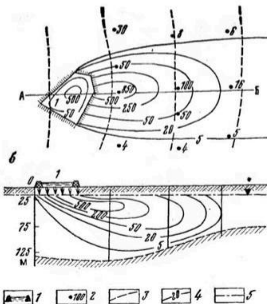
Рис. 37. Схема распространения загрязнения в подземных водах (по В. А. Грабовникову) a — план; б — разрез по линии А—Б: 1 — хвостохранилище, 2 — скважина и содержание микрокомпонента в мкг/л; 3 — гидроизогонсы; 4 — изолинии содержания микрокомпонента в мкг/л; 5 — уровень подземных вод
