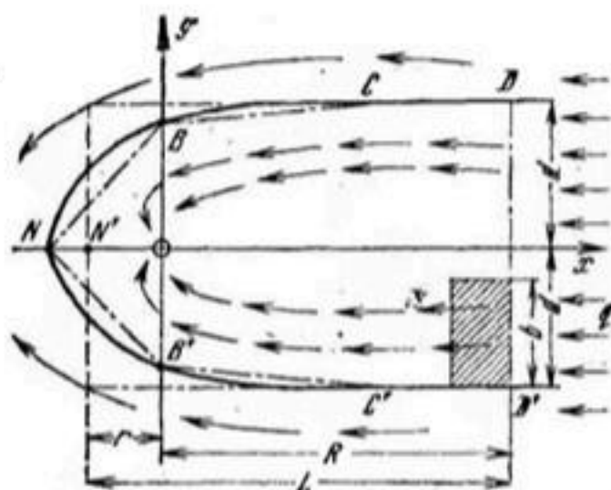
Рис. 56. Схема области захвата водозабора
