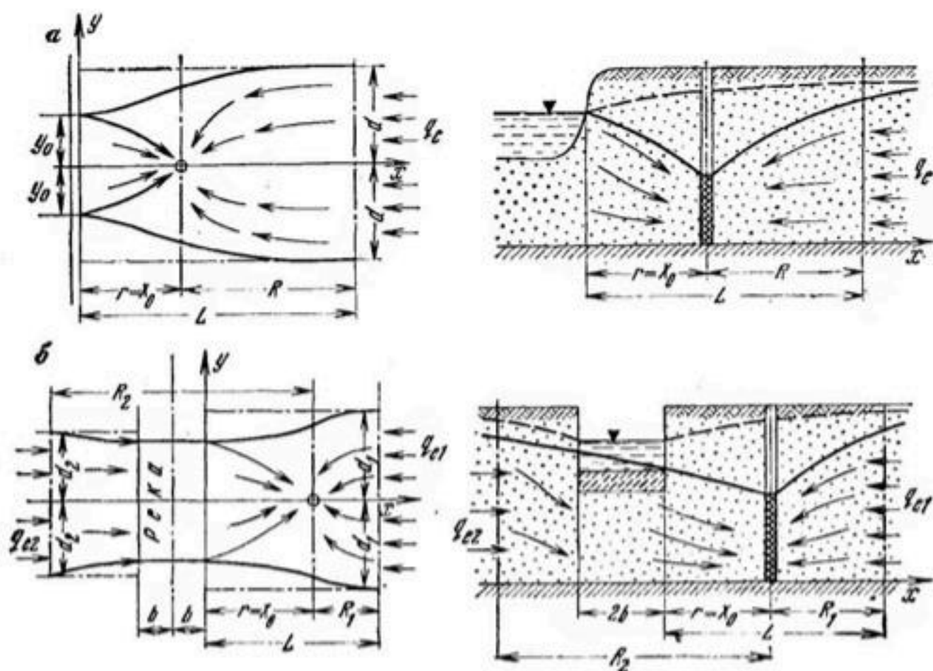
Рис. 59. Схемы фильтрации к береговому водозабору:
