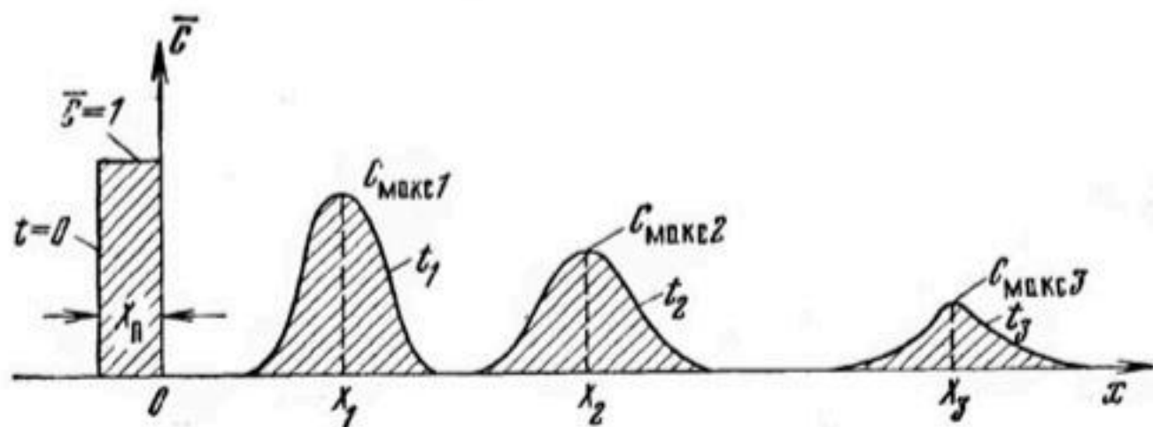
Рис. 33. Изменение концентрации вещества при «пакетном» запуске:
