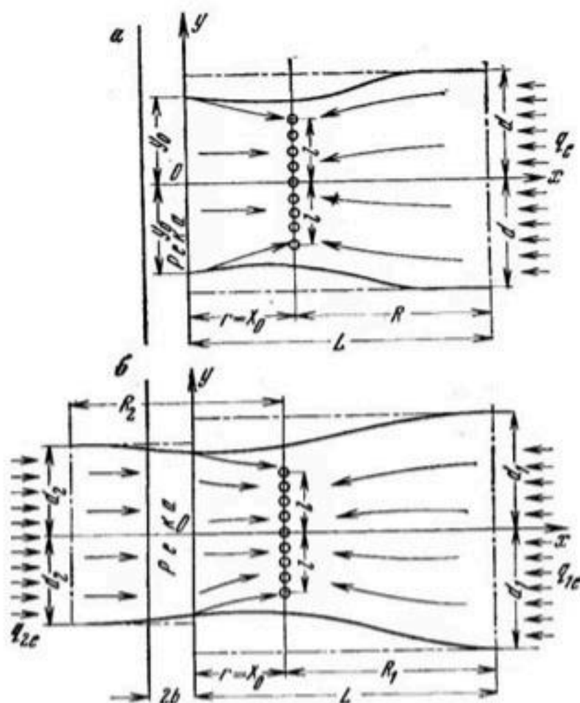
Рис. 61. Схемы фильтрации к линейному водозабору:
