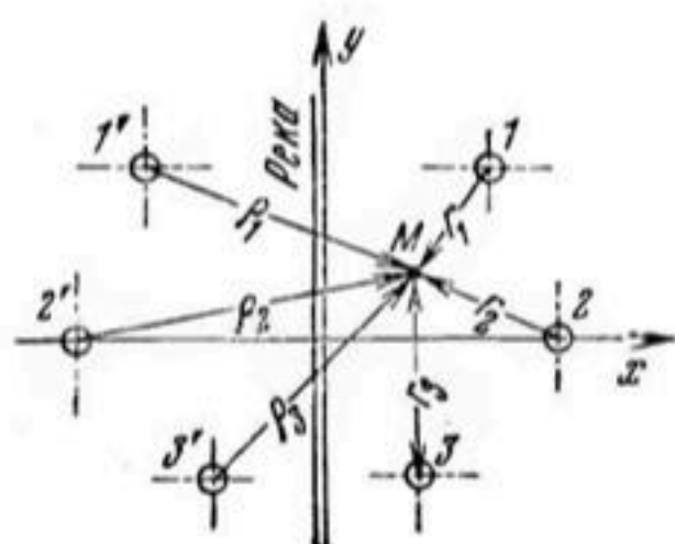
Рис. 17. Система взаимодействующих скважин у совершенной реки:
