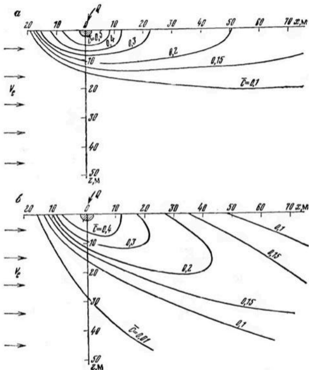
Рис. 35. Ареал распространения загрязнений в подземных водах в районе хранилища при \frac{Q}{2l} = 5 \text{ м}^3/\text{сут.} , Kl_e = 0,05 \text{ м/сут.} , D_x^* = D_y^* = 0,1 \text{ м}^2/\text{сут.}
