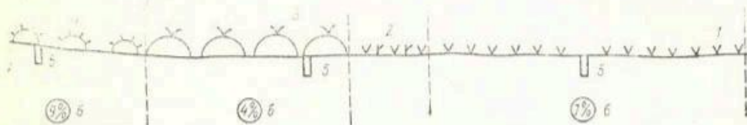
Рис. 5. Обобщенный геоботанический профиль в области контакта авандельты и обсохшей поверхности моря.
