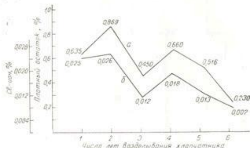
Рис. 2. Засоление почвы опытного участка в слое 0—50 см по плотному остатку (а) и хлор-иону (б) в зависимости от продолжительности возделывания хлопчатника.
