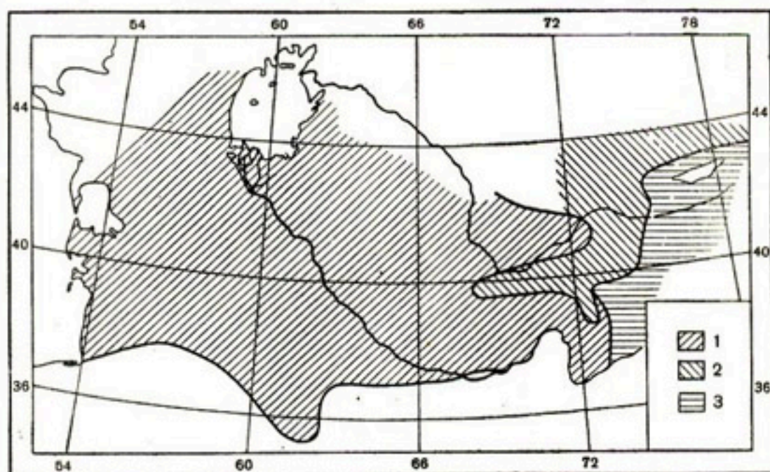
Рис. 75. Распределение различных типов годового хода осадков.
