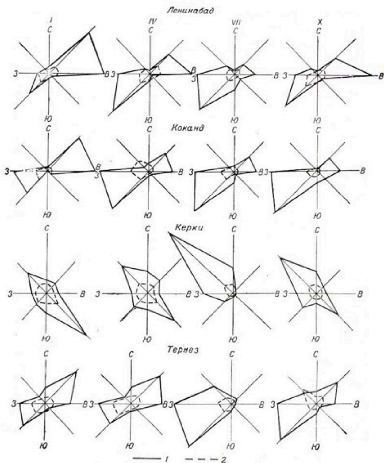
Рис. 39. Направление и скорость ветра. 1 — направление ( ^{\circ}/_{\text{в}} ), 2 — скорость (м/сек.).
