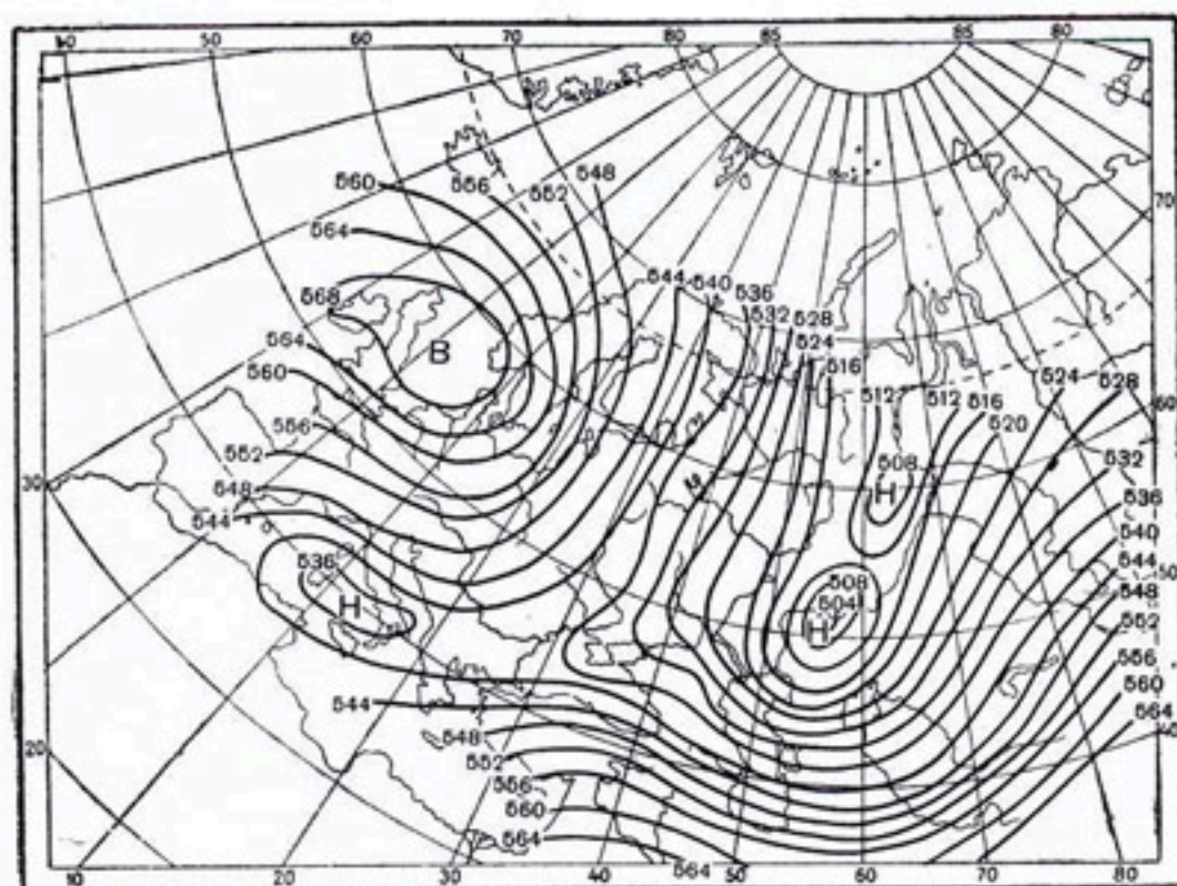
Рис. 18. Карта АТ 500 . 18 час. 20/І 1950 г.
