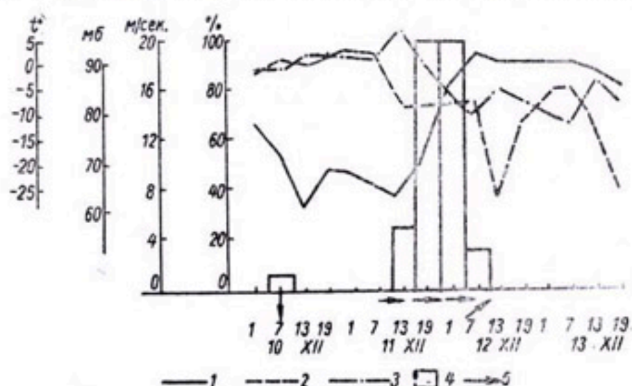
Рис. 44. Ход метеорологических элементов в Коканде. 10—13/XII 1952 г.
