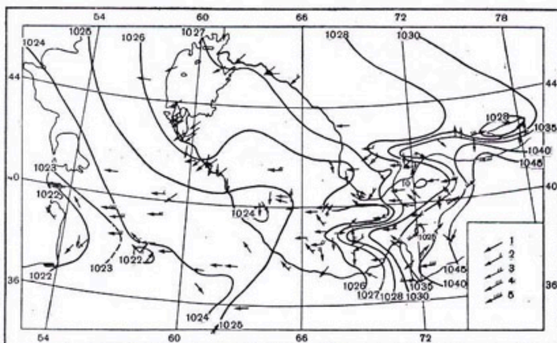
Рис. 29 Давление воздуха на уровне моря и преобладающие направления ветра. Январь. 1 — менее 30%, 2 — 30—40, 3 — 40—50, 4 — 50—60, 5 — более 60%.
