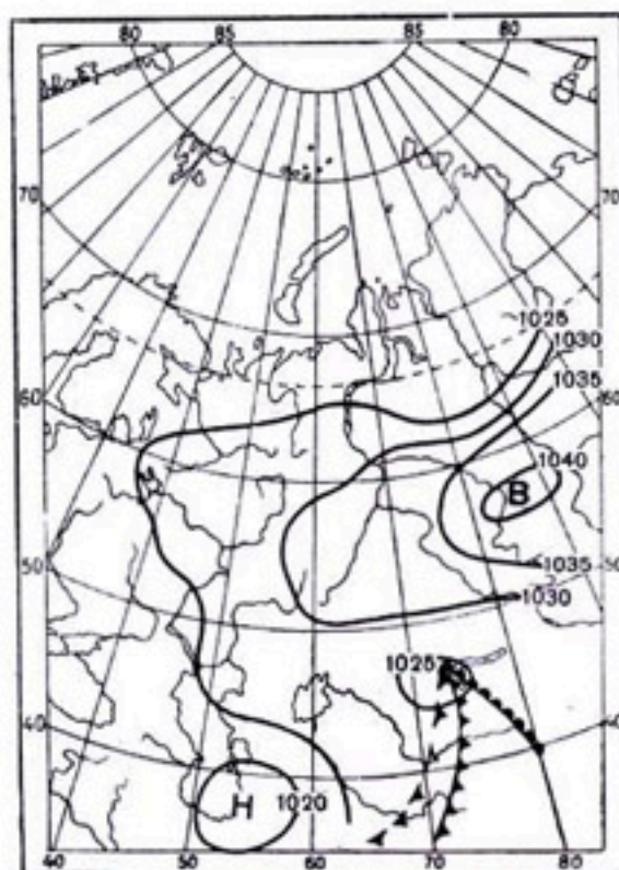
Рис. 86. Карта погоды. 07 час. 15/XII 1939 г.
