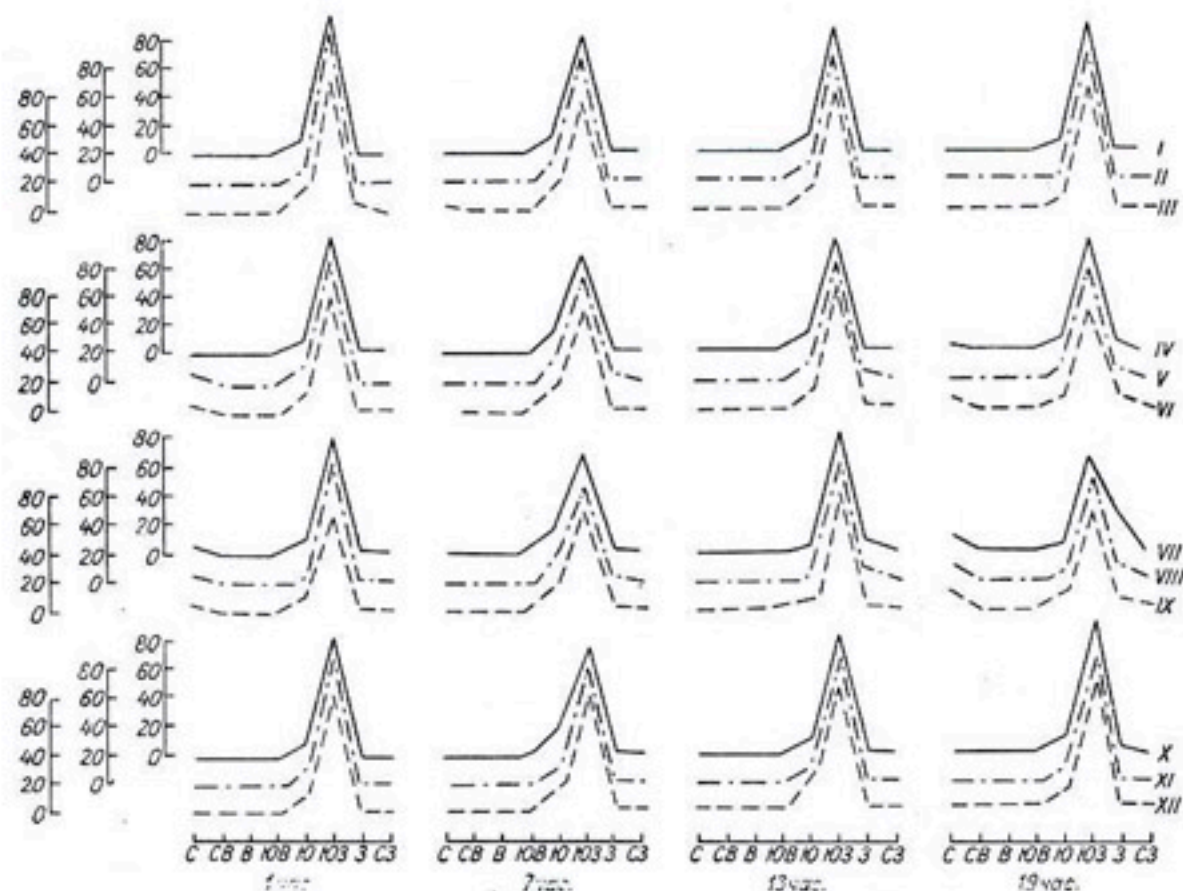
Рис. 50. Годовой и суточный ход ветра (%). Ледник Федченко.
