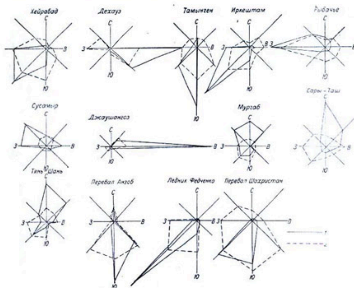
Рис. 45. Розы ветров в горной и высокогорной областях. Январь. 1 — направление (°/h), 2 — скорость (м/сек.).
