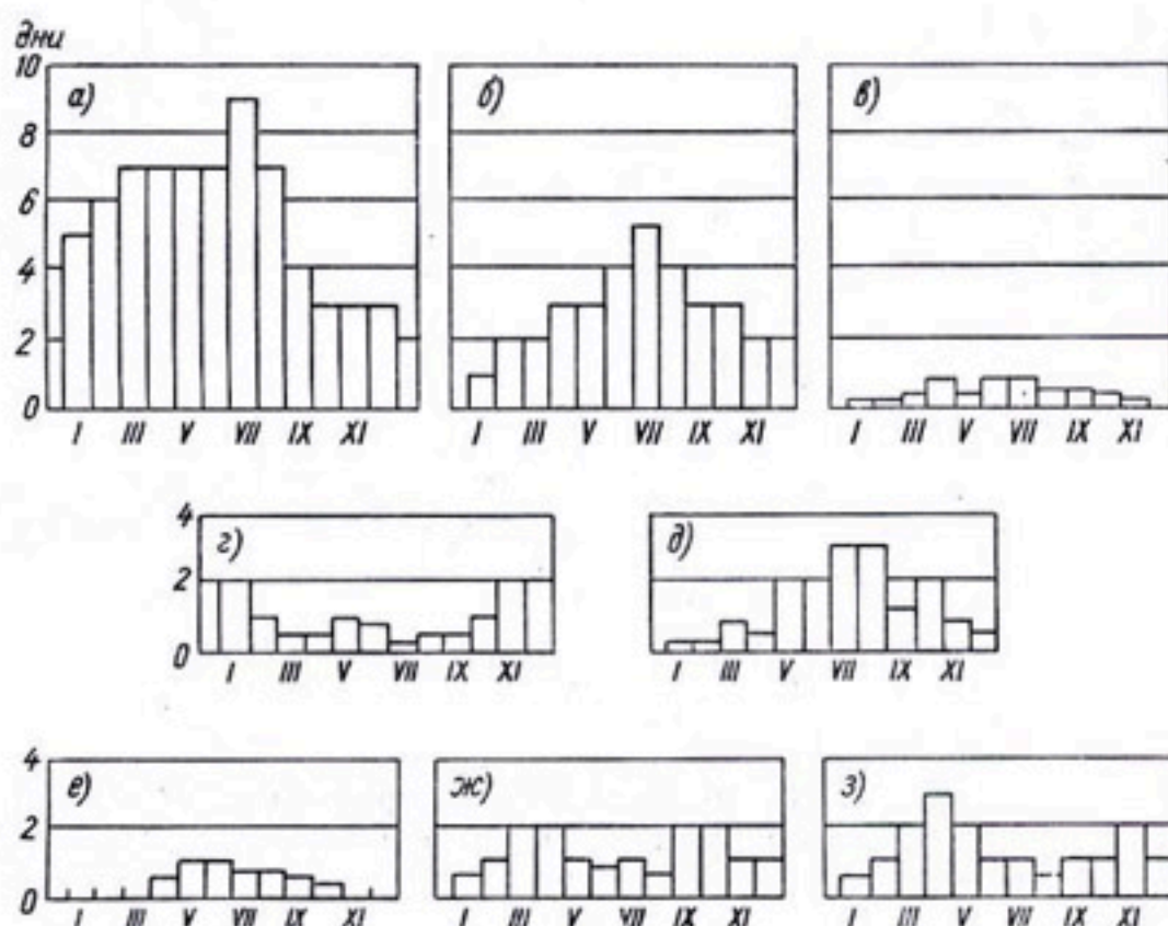
Рис. 92. Годовой ход числа дней с пыльными бурями. Равнины: а — Репетек, б — Тамды, в — Куйград; предгорья: з — Кушка, д — Карши; горы: е — Нарын, ж — Рыбачье, з — Мургаб.
