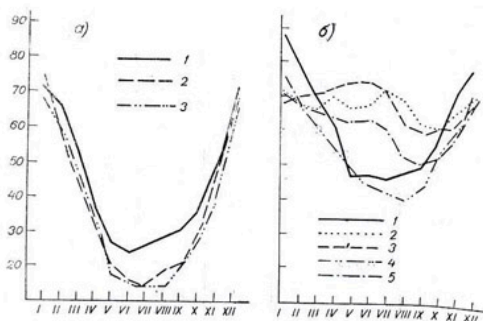
Рис. 68. Годовой ход относительной влажности в 13 час. а) 1 — Хива, 2 — Тамды (овasis), 3 — Зеагли (пустыня); б) прибрежная полоса: 1 — Муйнак, 2 — Гасан-Кули, 3 — Мыс Тарта, 4 — Красноводск, 5 — Челекен.
