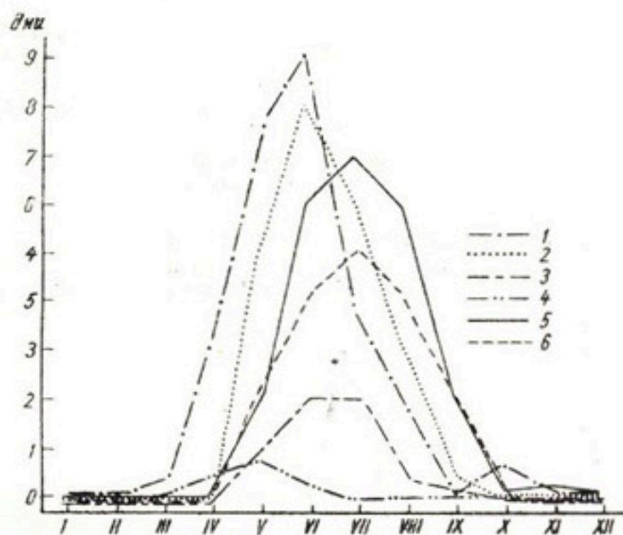
Рис. 90. Годовой ход числа дней с грозой. 1 — Перевал Анзоб, 2 — Сары-Таш, 3 — Мургаб, 4 — Ледник Федченко, 5 — Тянь-Шаньская обсерватория, 6 — Акшийрак.
