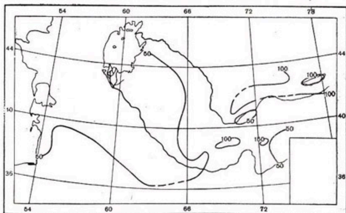
Рис. 77. Среднее годовое число дней с осадками \geq 0,1 мм.
