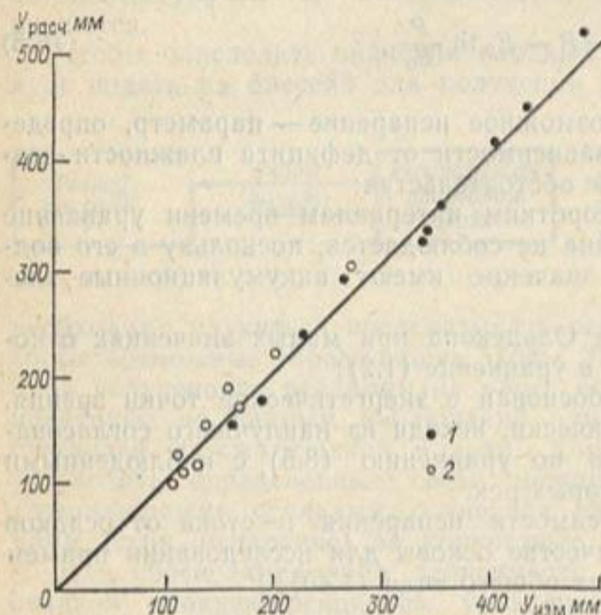
Рис. 15. Связь измеренных и рассчитанных значений стока.
