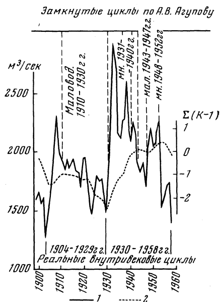
Рис. 2. Сопоставление реальных полных внутривековых циклов стока р. Ангары у с. Пашки с замкнутыми циклами по А. В. Агупову
