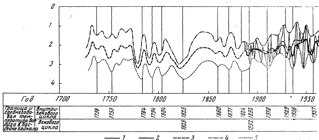
Рис. 31. Многолетние колебания температуры воздуха в бассейне оз. Байкал 1 — годовые значения; 2 — индекс \Sigma t/m по данным наблюдений; 3 — то же рассчитанный 4 — кривая максимальной температуры малых циклов; 5 — то же минимальной температуры
