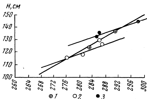
Рис. 28. График зависимости между средними цикловыми значениями уровней оз. Байкал и продолжительностью свободного состояния р. Ангары
