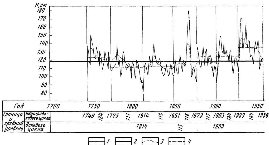
Рис. 23. Многолетние колебания уровня оз. Байкал у ст. Байкал
