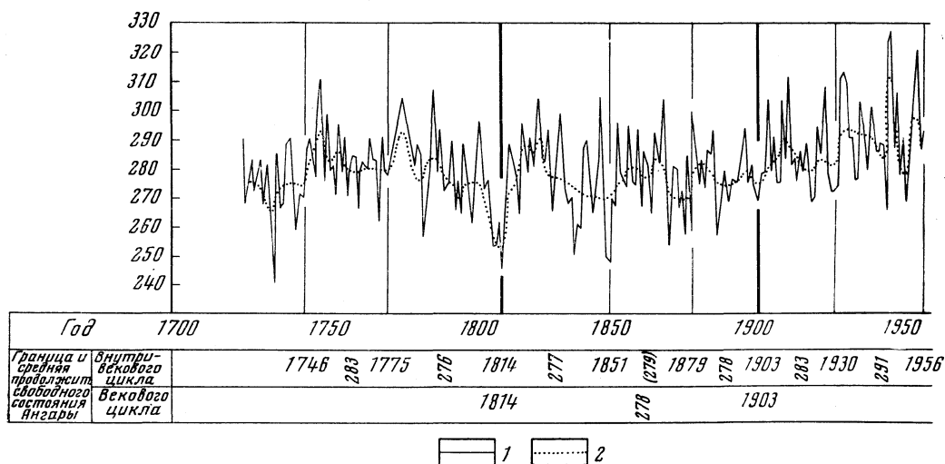
Рис. 24. Многолетние колебания продолжительности свободного состояния р. Ангары у г. Иркутска
