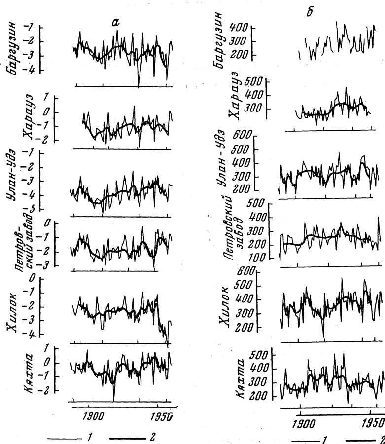
Рис. 12. Многолетние колебания и изменения температуры воздуха (а) и атмосферных осадков (б) в бассейне оз. Байкал
