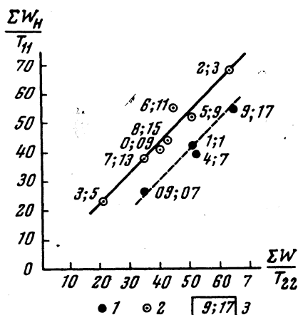
Рис. 10. Зависимость между \Sigma W/T_{22} и \Sigma W_n/T_{11}
