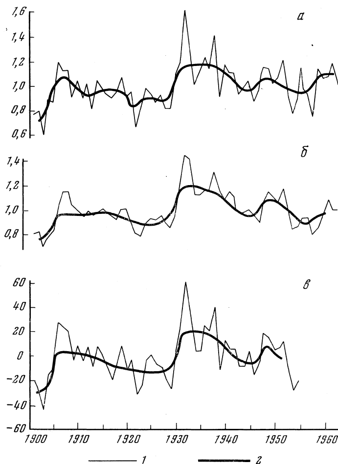
Рис. 15. Многолетние колебания прихода (а), расхода (б) воды в оз. Байкал и взаимосвязь их с уровнем воды на 1 января (в) 1 — годовые значения; 2 — индексы \Sigma X_M/n
