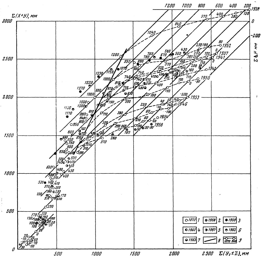
Рис. 21. Графики связи между суммарными месячными значениями прихода, расхода и приращения уровня воды оз. Байкал
