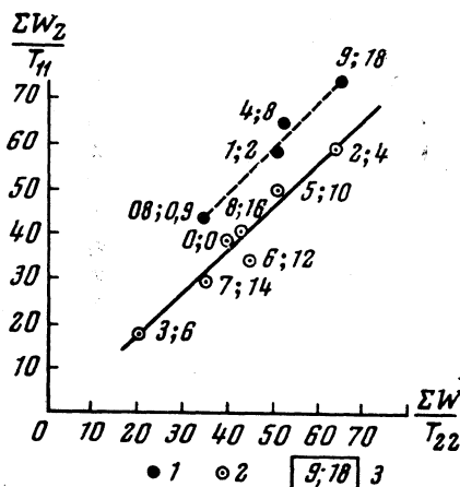
Рис. 11. Зависимость между \Sigma W/T_{22} и \Sigma W_r/T_{11}
