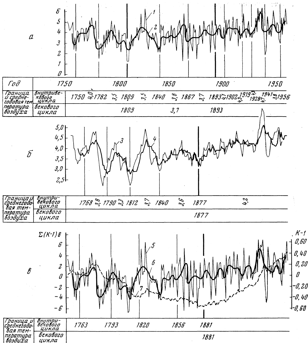
Рис. 3. Сопоставление многолетнего хода индекса \Sigma t_m/n среднегодовой температуры воздуха по Ленинграду (а) с хронологическим графиком осредненных по скользящим n -летним (б) и разностной интегральной кривой (в) за период 1743—1962 гг.
