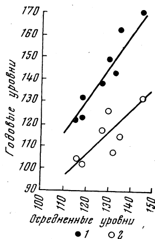
Рис. 29. График зависимости между максимально-минимальными годовыми и средними цикловыми значениями уровней (индекс \Sigma H_{\text{м}}/n ) оз. Байкал
