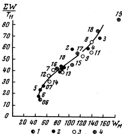
Рис. 7. Зависимость между \Sigma W/T_{11} и W_M
