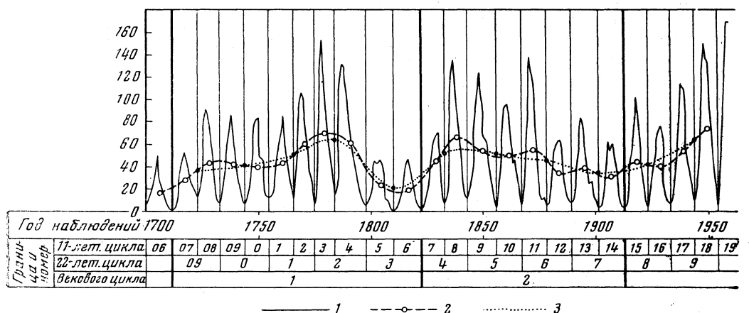
Рис. 5. Многолетние колебания солнечной активности
