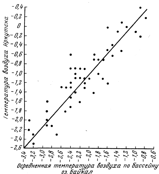
Рис. 26. График связи между годовыми значениями температуры воздуха по метеорологической станции Иркутск и осредненными по 6-ти станциям в бассейне оз. Байкал температурами
