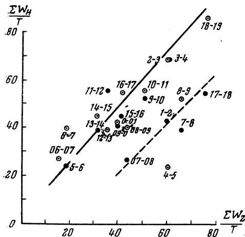
Рис. 6. Зависимость между \Sigma W_n / T_{11} и \Sigma W_r / T_{11}
