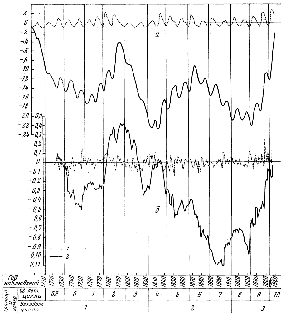
Рис. 25. Многолетние колебания солнечной активности (а) и продолжительности свободного состояния реки Ангары у г. Иркутска (б)
