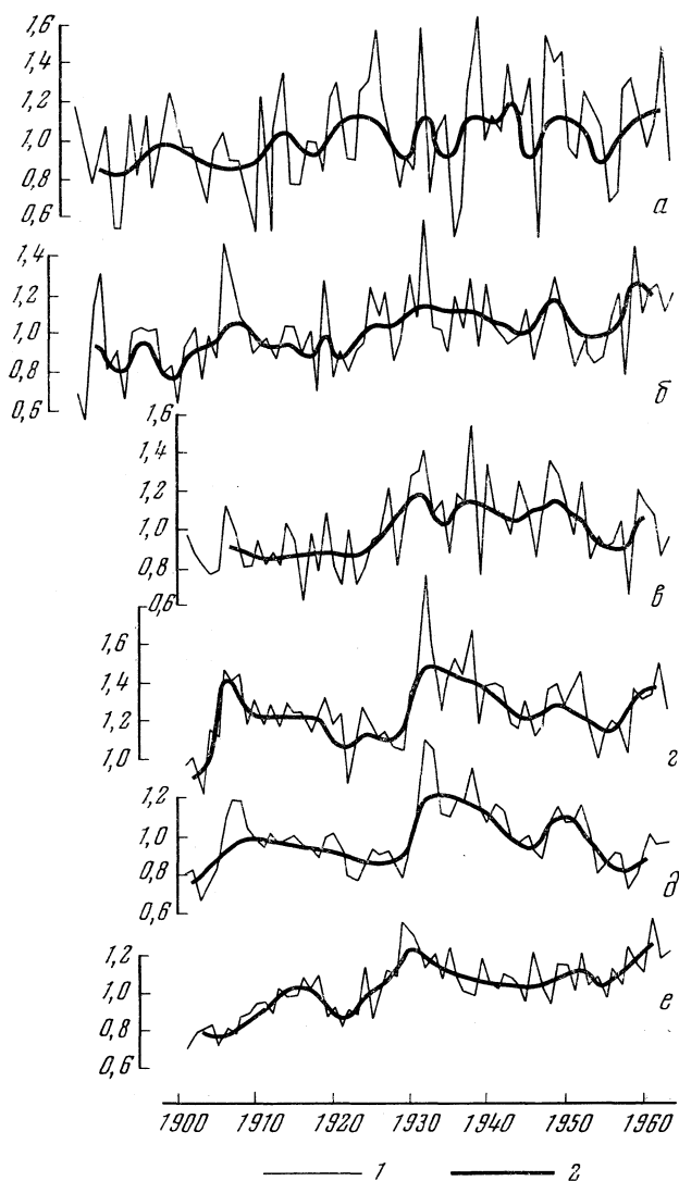
Рис. 14. Многолетние колебания элементов водного баланса оз. Байкал и связь их с определяющими элементами 1 — годовые значения: температуры (а) и осадков в бассейне (б), осадков на поверхности озера (в), притока (г), стока (д) и испарения (е); 2 — соответственно индексы \sum X_M/n
