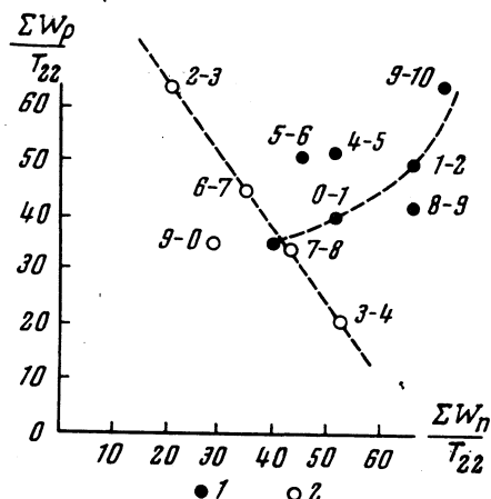
Рис. 9. Зависимость между \Sigma W_p/T_{22} и \Sigma W_n/T_{22}
