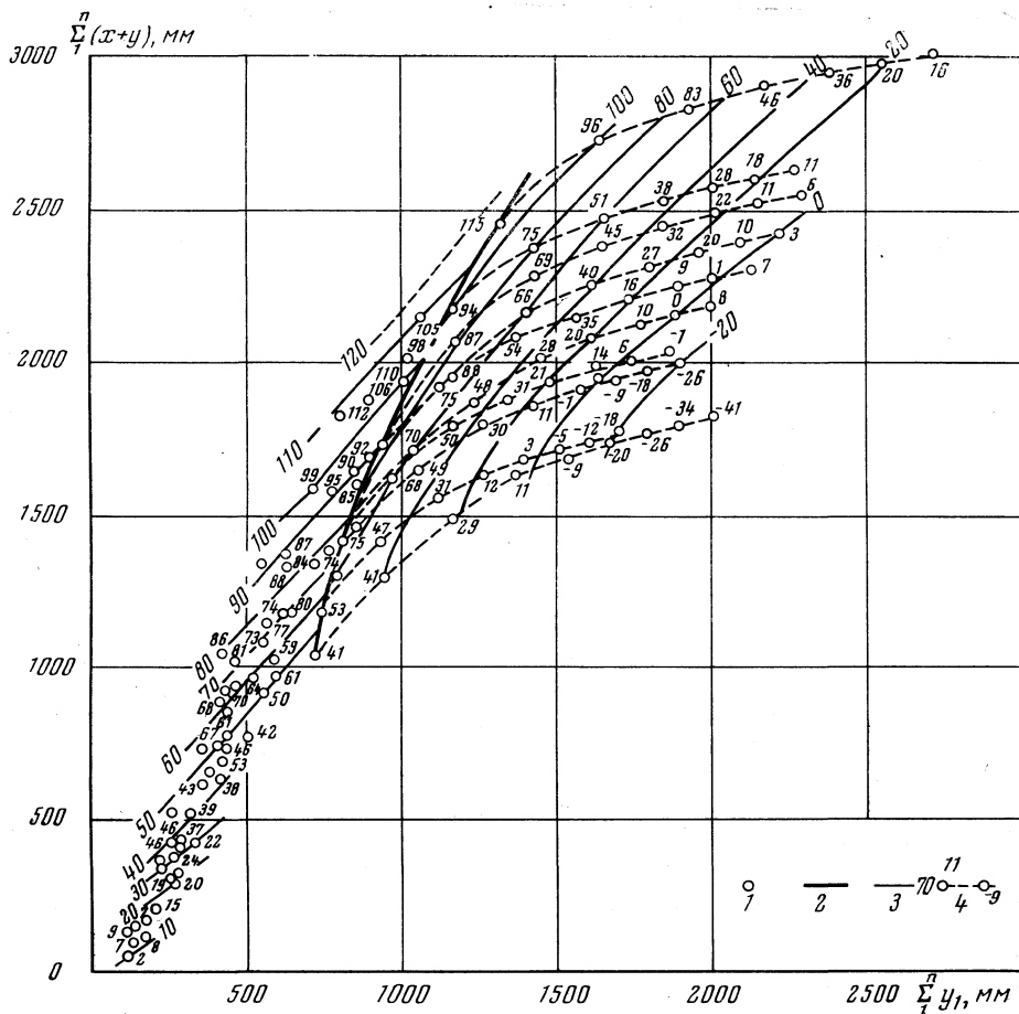
Рис. 22. Зависимость суммарного приращения уровня воды в озере за последующий n + 1 -й месяц (см) и суммарного прихода воды в озере от суммарного расхода воды из него за предыдущий n -й месяц (мм)
