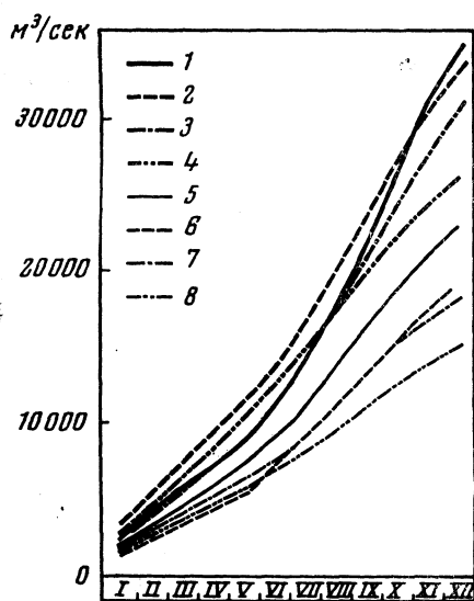
Рис. 20. Интегральные кривые стока из оз. Байкал
