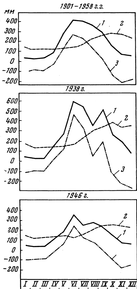
Рис. 18. Годовой ход прихода-расхода и приращения уровня воды в оз. Байкал за период 1901—1958 гг.
