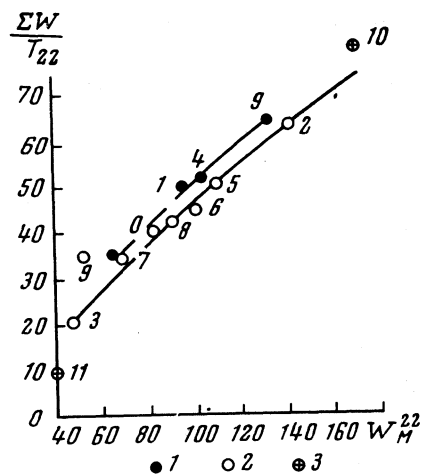
Рис. 8. Зависимость между \Sigma W/T_{22} и W_M^{22}
