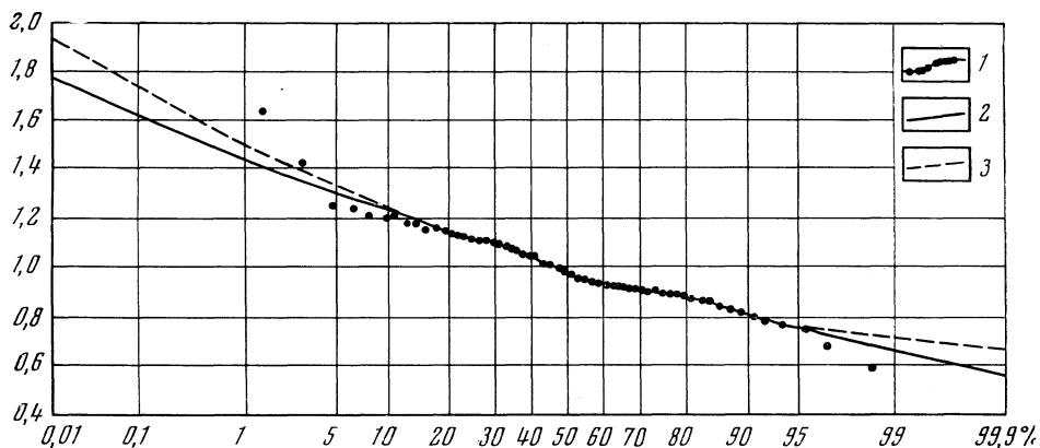
Рис. 17. Кривые обеспеченности годового прихода воды в оз. Байкал 1 — эмпирические точки, вычисленные по формуле P\% = m/(n + 1) \cdot 100 ; 2 — C_s = 2C_v ; 3 — C_s = 5C_v
