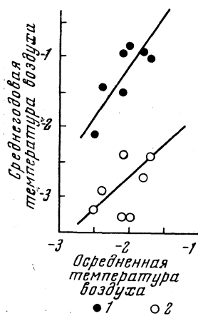
Рис. 30. График зависимости между максимально-минимальными годовыми и средними цикловыми значениями температуры воздуха (индекс \Sigma t_{\text{м}}/n ) в бассейне Байкала
