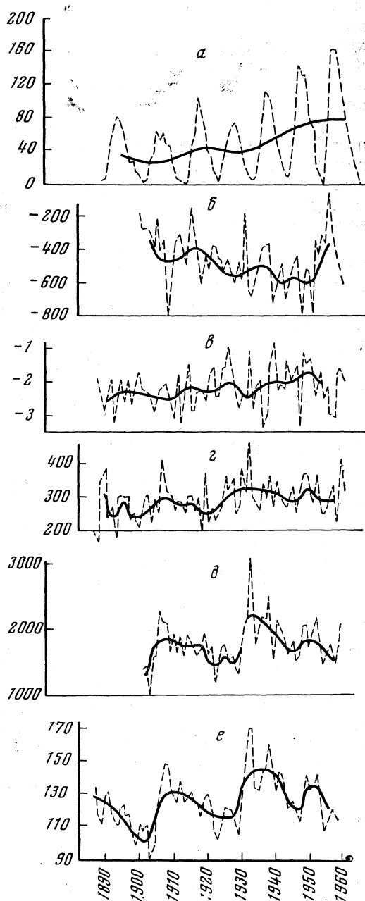
Рис. 13. Взаимодействие годового хода солнечной активности (числа Вольфа) (а), циркуляция воздуха (б), температура воздуха (в) и атмосферных осадков (г) в бассейне Байкала, притока воды в оз. Байкал (д) и колебаний уровней в нем (е). 1 — годовые значения; 2 — индекс \Sigma X_{M/n}
