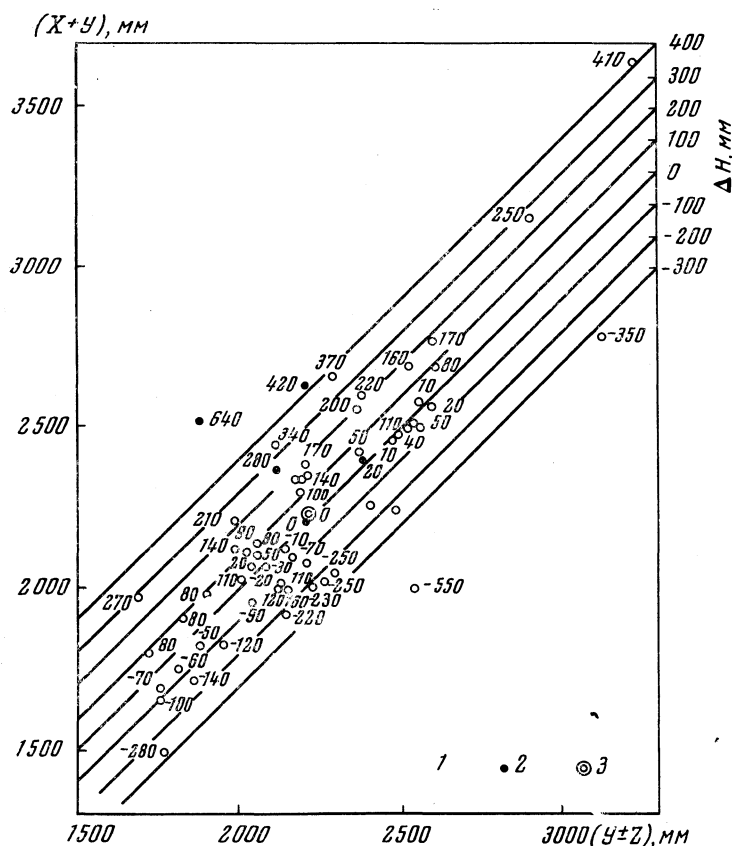
Рис. 16. Графики связи между годовыми значениями прихода, расхода и приращения уровня воды оз. Байкал
