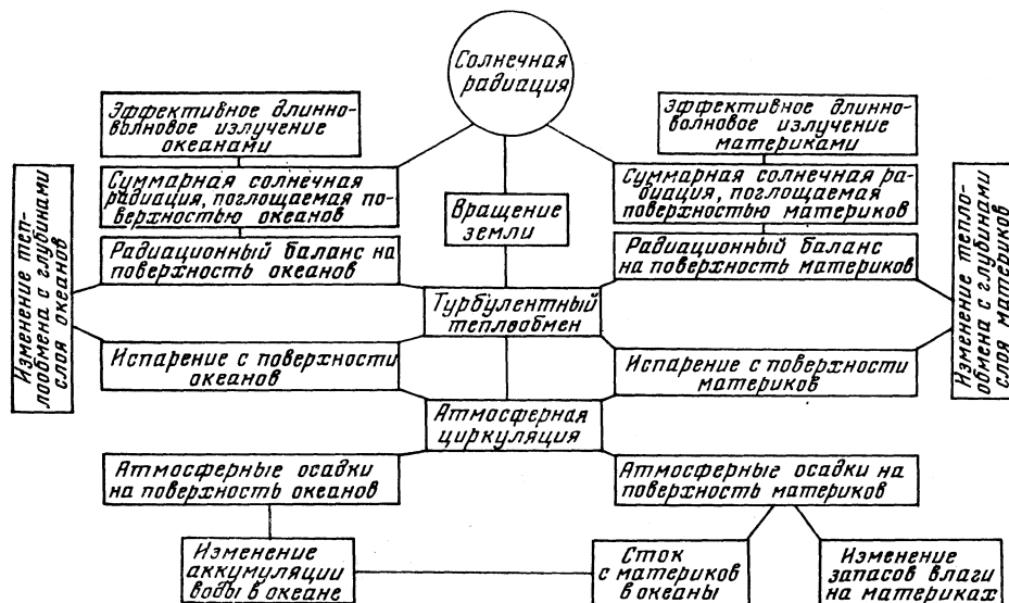
Рис. 1. Принципиальная схема формирования циклических колебаний и изменений компонентов теплового и водного баланса Земли
