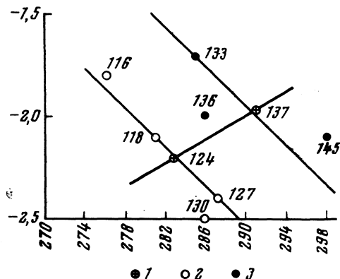
Рис. 27. График зависимости между средними значениями температуры воздуха в бассейне оз. Байкал, продолжительности свободного состояния р. Ангары и уровней оз. Байкал
