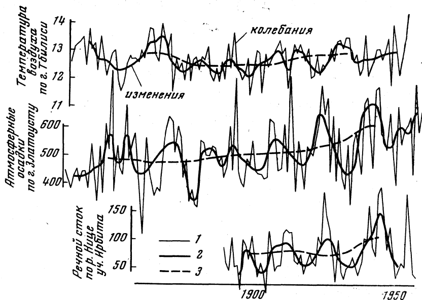
Рис. 4. Схема динамики колебаний и изменений некоторых основных гидрометеорологических факторов
