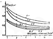
Рис. 37. Изменение предельной прочности песчаной корки на продавливание в зависимости от площади штампика I — при температуре воздуха 36 (1), 39 (2) и 42° (3). Корки получены путем опрыскивания песчаной поверхности отработанным маслом с добавкой битума (I) и керосина (II).
