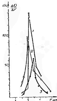
Рис. 7. Кривые распределения частиц по радиусам 2%-ной суспензии глины Котурдепе (1), Барсакельмес (2), Вышки (3).
