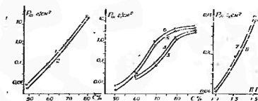
Рис. 9. Изменение предельного напряжения сдвига барсакельмесской (1) и аннаууской (2) глин; котурделипского (3) и аннаууского (4) песков; смеси котурделипского песка с барсакельмесской глиной при 1:1 (5) и аннаууского песка с аннаууской глиной при 1:1 (6) от концентрации твердой фазы и 60%-ной суспензии смеси котурделипского песка с барсакельмесской (7) и аннаууской глинной (8) от соотношения песка и глины.
