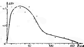
Рис. 42 Изменение влажности ( \Delta W = W_s - W_1 ) на опытных с К-9 ( W_s , %) и контрольном ( W_1 , %) участках в зависимости от глубины ( h , см) разреза.
