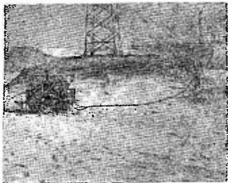
Рис. 33. Использование установки ЛСД-2М для закрепления оснований снос линий электропередачи
