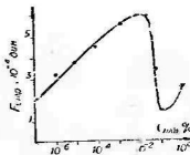
Рис. 23. Зависимость силы прилипания сферических частиц к подложке в растворах электролитов.
