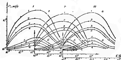
Рис. 21. Изотермы адсорбции полиэлектролитов К-9(1), К-6(2), Сунак-2(3), ВРП-1(4) глинами (а) и песками (б) из Котурдесе (I), Барсакельмесс (II) и Айнау (III).
