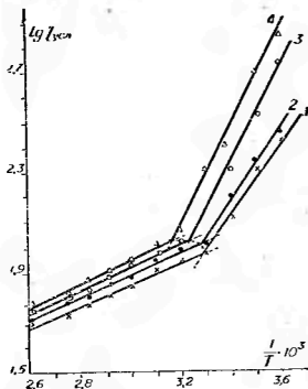
Рис. 10 Зависимость \lg \eta_{всх} - 1/T обработанного масла (1) и 100:1 (2), 100:5 (3), 100:10 (4)-ной смеси масло-битум.
