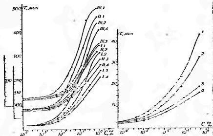
Рис. 30 Зависимость размокания каторпенской (II), барсакельмесской (II), выщелоченной (III) глины (А) и аназаского песка (Б) от концентрации растворов К-9 (1), К-6 (2), Сунак-3 (3), ВРП-1 (4).
