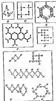
Рис. 3. Предполагаемые типы структур воды: а — тетраэдрическая, n=4 ; б — \mu=72 (Боалдер Р. В., Касснер Дж. А. Ципе Дж. Г.); в — кольцевая тетрамер, m=4 , \mu=72 (Белла Дж. Д., Осборн А. К., Липиникотт Е. Р., Бэйдли А. Р.); г — гексагональная, m=6 , \mu=108 (Липиникотт Е. Р., Штромберг Р. Р., Грант В. Т., Кессом Т. А.); д — разветвленная полимерная цепь (те же, что и в в); е — ассоциация возбужденных молекул H_2O (Гуринов Ю. В.); ж — молекулярные агрегаты в жидкой воде (Адамс М.).
