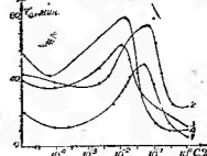
Рис. 27. Зависимость времени формирования осадка в суспензиях глины Котурдас (1), Барскальмес (2), Огдылы (3), Визки (4) от содержания в них полиэлектролита К-9.
