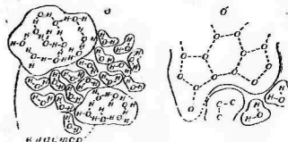
Рис. 5. Схематическое изображение Немети и Шерага модели чистой (а) и содержащей углерод (б) воды.
