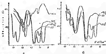
Рис. 17 ИК-спектры: а) — NaCl + D 2 O, Na 2 SO 4 + D 2 O, Na 3 PO 4 + D 2 O, K-4 + D 2 O, б) K-4 + D 2 O, NaCl, Na 2 SO 4 , Na 3 PO 4 .
