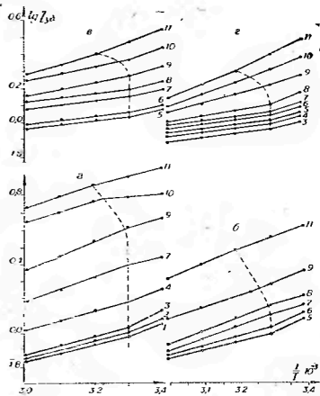
Рис. 14. Зависимость \lg \eta_{sp}/c — 1/T для растворов полиэлектролитов К-9 (а), К-6 (б), Сунак-2 (в), ВРП-1 (г), 1-9,7 \cdot 10^{-4} , 2-1,0 \cdot 10^{-3} , 3-3,9 \cdot 10^{-3} , 4-7,5 \cdot 10^{-3} , 5-1,5 \cdot 10^{-2} , 6-3 \cdot 10^{-2} , 7-6,2 \cdot 10^{-2} , 8-1,2 \cdot 10^{-1} , 9-2,5 \cdot 10^{-1} , 10-5,0 \cdot 10^{-1} , 11-1,0 \cdot 10^{-1} .
