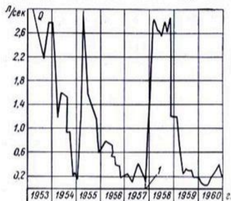
Рис. 8-15. График дебита скважины. 1 — момент смены фильтра.
