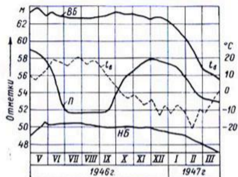
Рис. 8-14. Кривые изменения уровней бьефов ВБ и НБ, воды в пьезометре П и температуры воздуха t_a .
