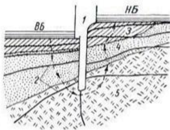
Рис. 3-18. Схема плановой фильтрации в неоднородном пласте. 1 — плотина; 2 — гидроизогипсы; 3, 4, 5 — зоны различной водопроницаемости; БВ — верхний бьеф; НБ — нижний бьеф.
