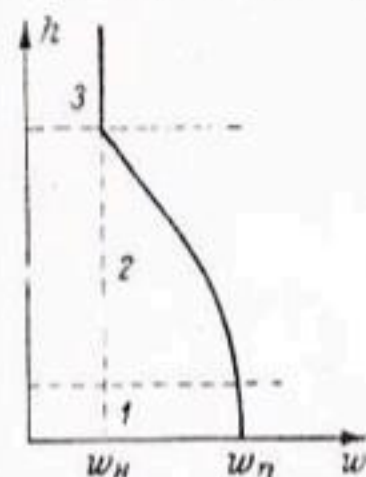
Рис. 2-3. Распределение влагосодержания по высоте пласта.
