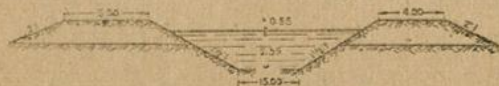
тип. сеч. от ПК N 0+0 до ПК N 13+60
