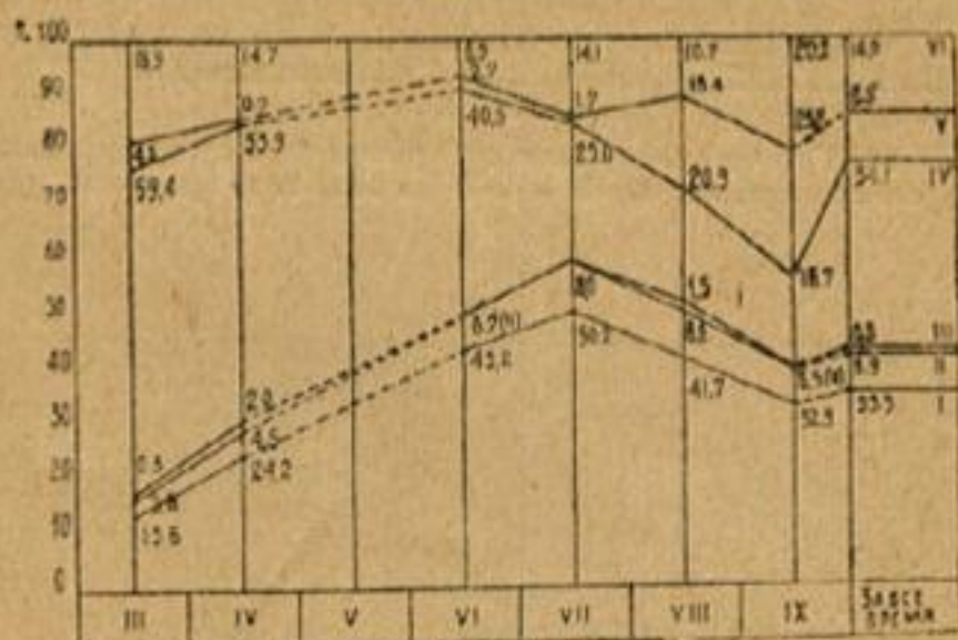
Черт. 59. График баланса суммарного рабочего времени по экскаватору № 214 Монинган за все время работы по группам: I—чистое рабочее время; II—простои, связанные с производством работ (нормальная передвинка, холостой ход) III—оргпростои (планировка и расчистка, отсутствие горючего, воды, освещения) IV—простои, связанные с конструкцией машины (ремонт, набор воды и топлива, смазка, промывка и проч.); V—прочие простои; VI—дни отдыха
