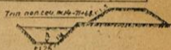
Черт. 71. Сокращенный поперечный профиль Галацкого Водосборного канала
