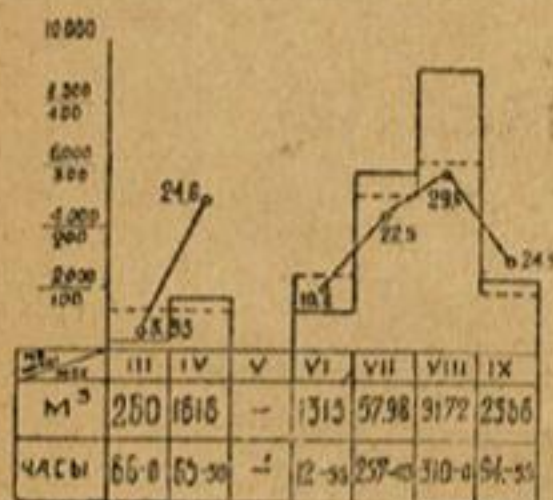
Черт. 58. График объемов произведенных работ, числа часов чистого рабочего времени и производительности 1 часа последнего по месяцам за все время работы экскаватора № 214 Монинган
