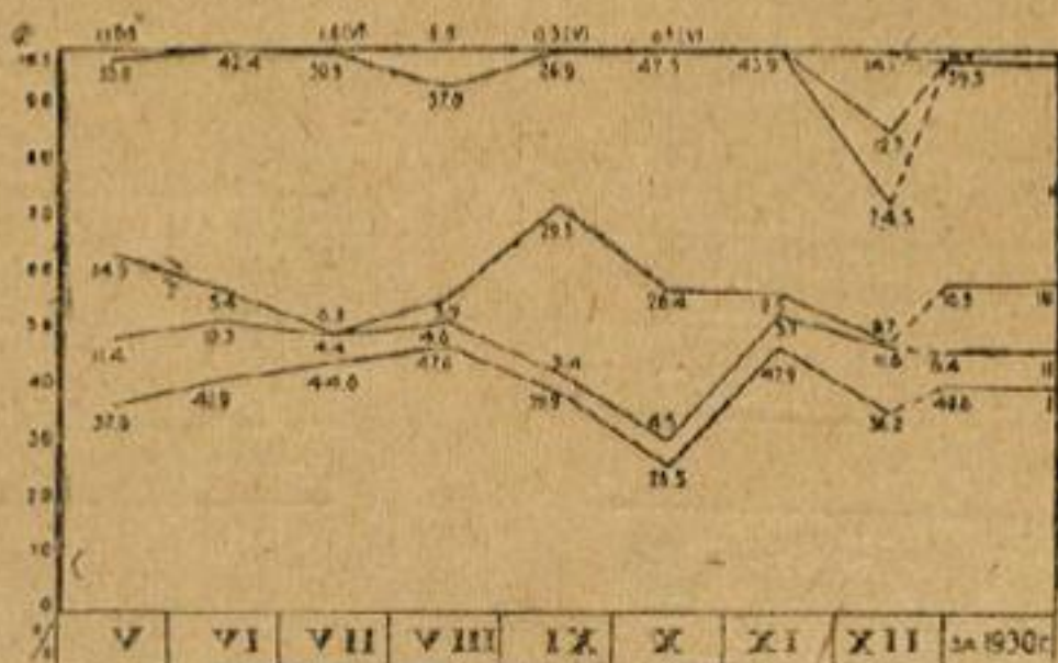
Черт. 73. График баланса суммарного рабочего времени по экскаватору кл. 7 М 851 по месяцам в 1930 г. и за все время работы по группам: I—чистое рабочее время; II—простой, связанные с производством работ (нормальная передвигка, холостой ход); III—оргпростои (планировка и расчистка, отсутствие горючего, воды, освещения); IV—простой, связанные с конструкцией машины (ремонт, набор воды и топлива, смазка, промывка котла и проч.) V—прочие простои; VI—дни отдыха
