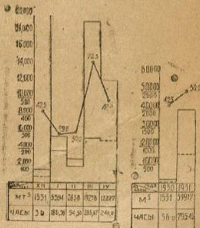
Черт. 85 и 86. Графики объема произведенных работ, числа часов чистого рабочего време- ни и производительности 1 ча- са последнего по месяцам 1980 31 года и по годам экскава- тора Остии
