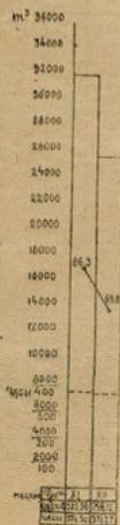
Черт. 17. График месячной выработки, чистого рабочего времени и часовой производительности экскаватора Бьюсабурга в класс 50-В № 9736 за 1978 год
