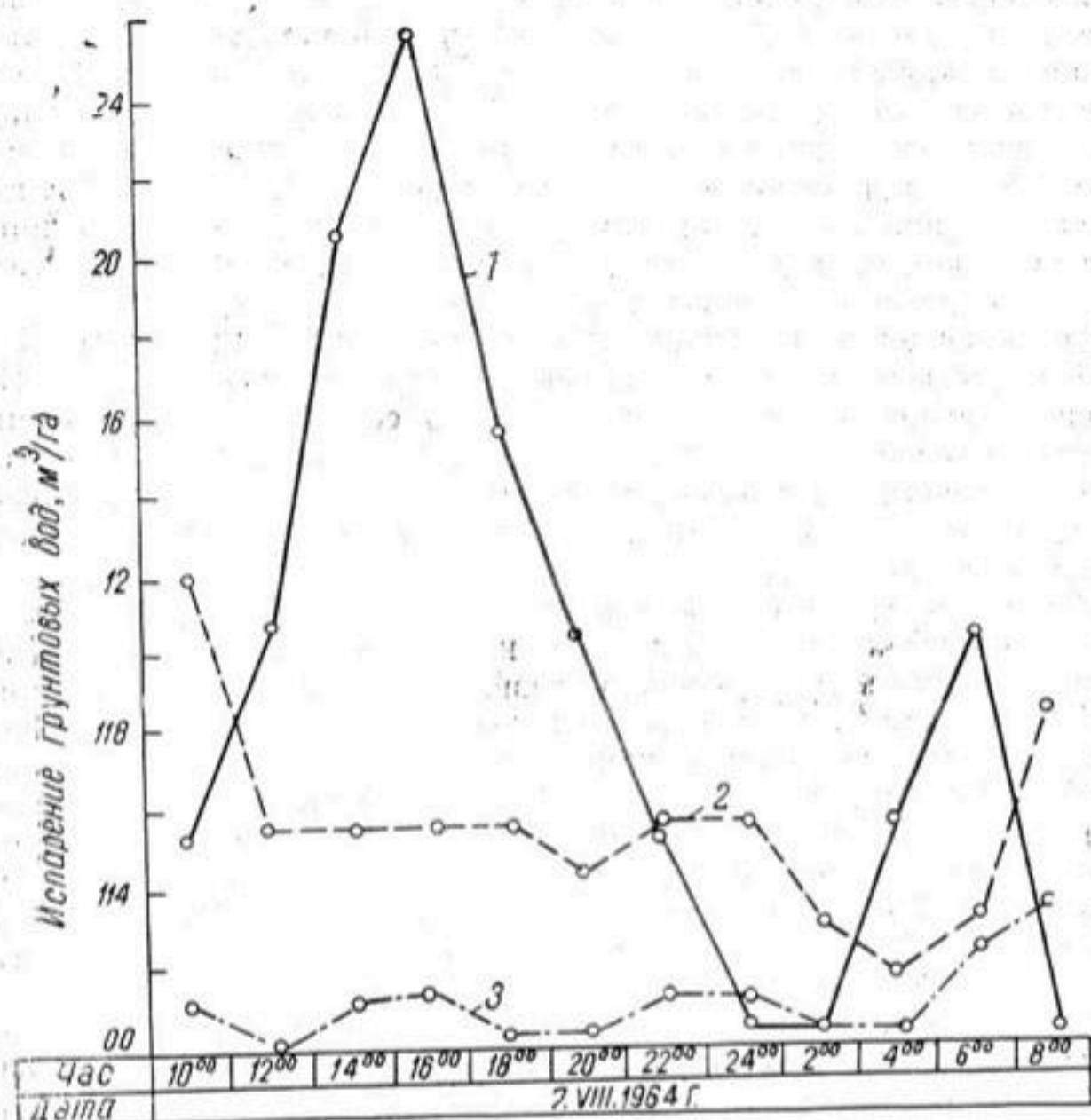
Рис. 4. Суточный ход испарения грунтовых вод хлопчатником с глубины 1,0 м (1), 1,5 (2), 2,0 м (3) от поверхности земли, площадь лизиметра 0,36 м 2 , размер сторон 0,6×0,6 м.
