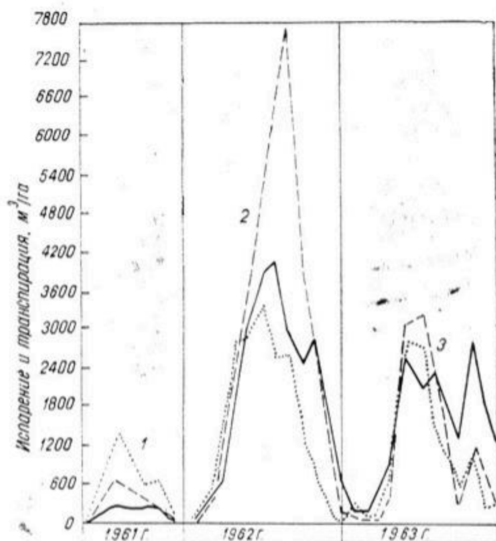
Рис. 5. График испарения и транспирации грунтовых вод люцерной первого (1961), второго (1962) и третьего (1963) годов посева при глубинах уровня воды в лизиметре 1,0 м (1), 1,5 (2), 2,0 (3) от поверхности.
