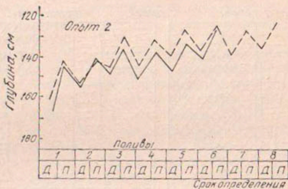
рис. 3. Динамика уровня грунтовых вод (хлопковое поле).
