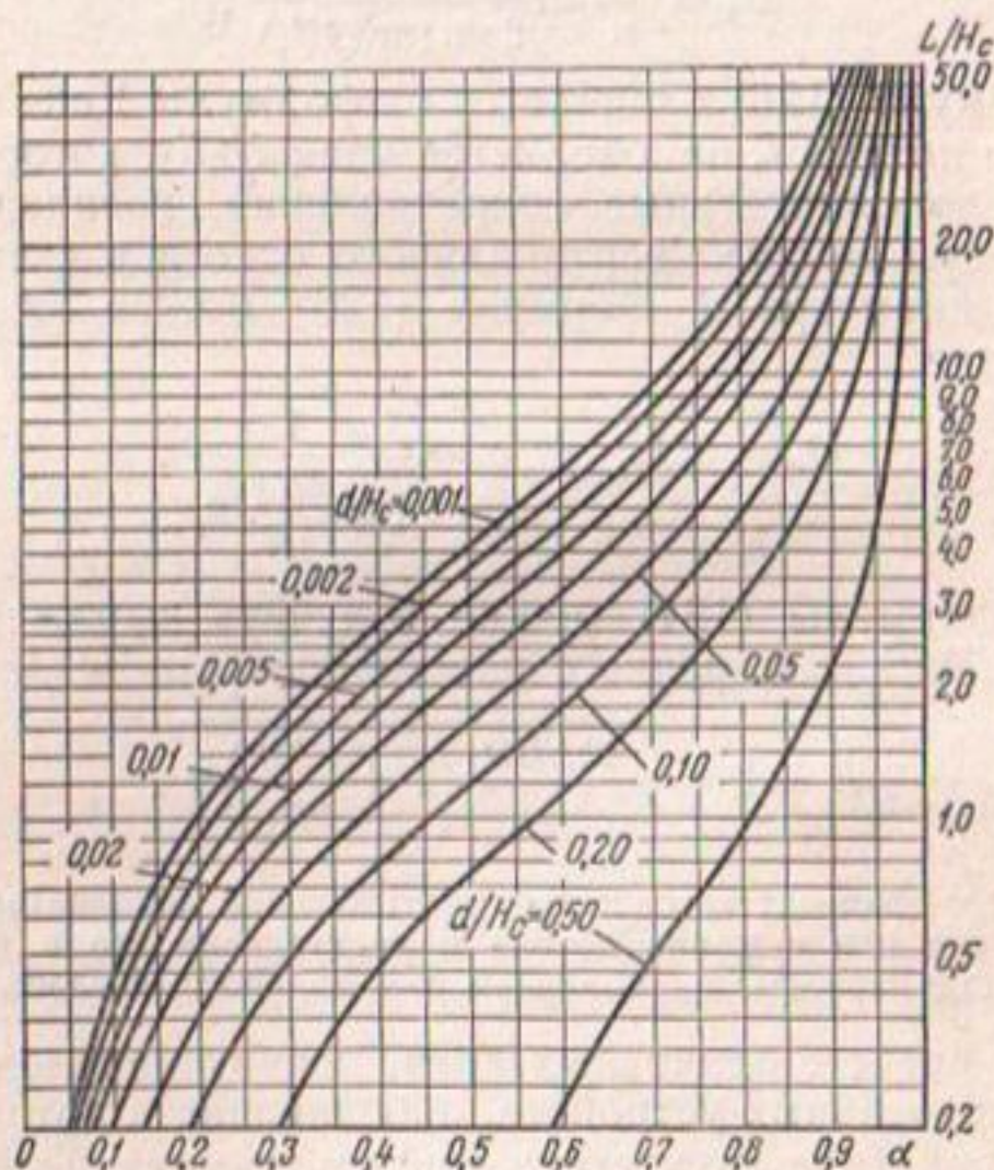
Рис. 23. График для определения коэффициента висячности дренажа \alpha :
