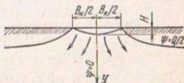
Рис. 48. Схема к расчету фильтрации из одиночного канала.
