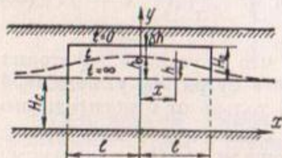
Рис. 17. Схема растекания бугра грунтовых вод.
