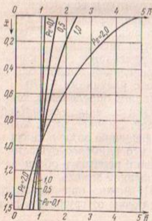
Рис. 4. Влияние параметра Пекле на распределение солей при \bar{V} = 1,5, \bar{n}_2 = 0,2 .
