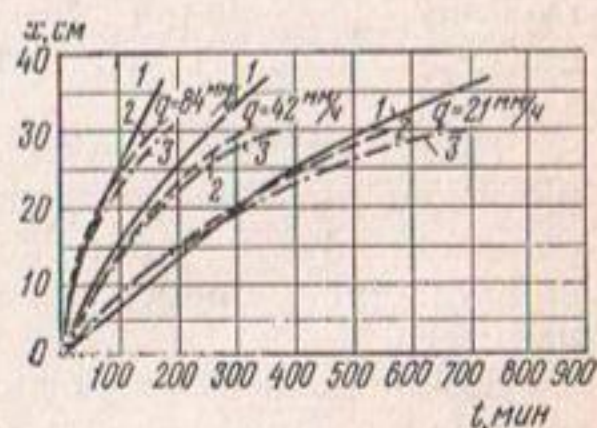
Рис. 14. Сравнение теоретических и экспериментальных данных по рассолению почвогрунтов при глубоком водоупоре:
