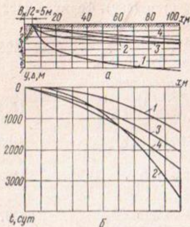
Рис. 49. Поверхность грунтовых вод (а) и динамика продвижения фронта опреснения (б) при фильтрации из одноканала и различных условиях оттока.
