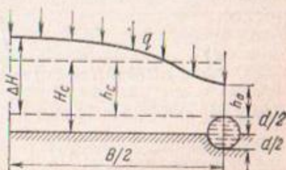
Рис. 24. Схема к расчету горизонтального дренажа при наличии инфильтрации (залегание дрен на водоупоре).
