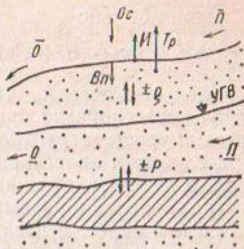
Рис. 1. Схема составляющих водного баланса:
