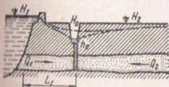
Рис. 43. Схема к расчету берегового дренажа.
