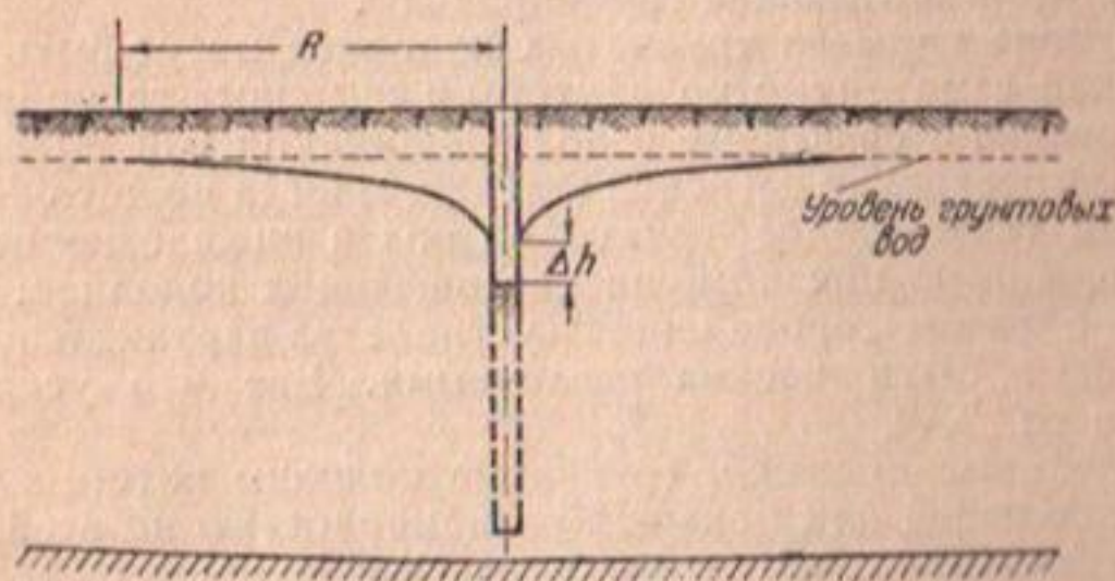
Фиг. 706. Схема понижющего действия трубчатого колодца
