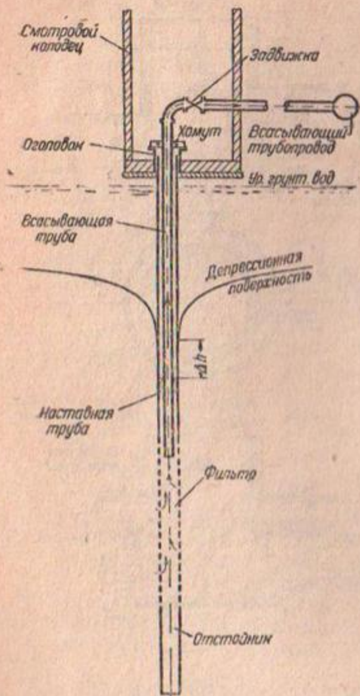
Фиг. 70а. Общая схема трубчатого колодца
