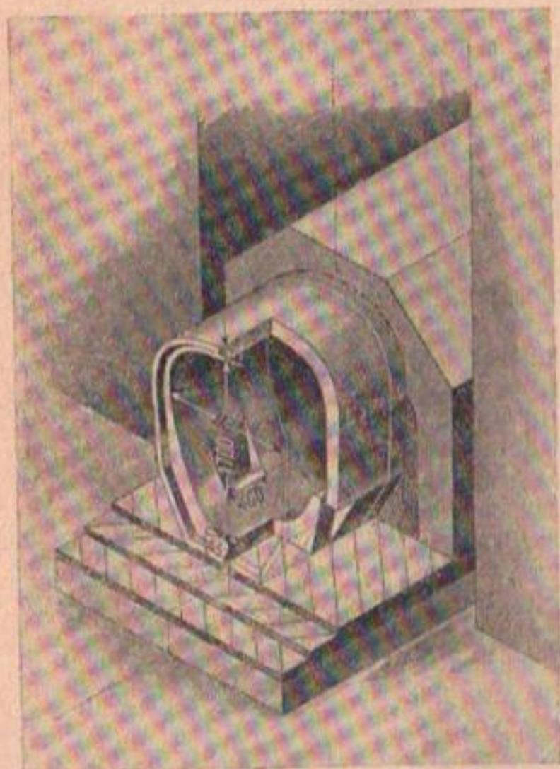
Фиг. 95. Горизонтальная дрена с колокольчатыми фильтрами
