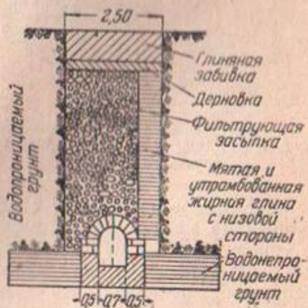
Фиг. 38. Дренажная галерея с экраном
