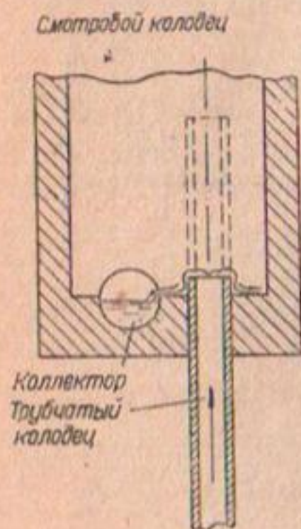
Фиг. 87. Схема присоединения трубчатого колодца к коллектору
