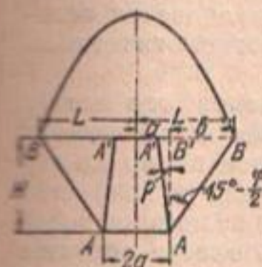
Фиг. 60 Схема определения безопасных расстояний дренажных штолен от зданий при туннельном способе работ
