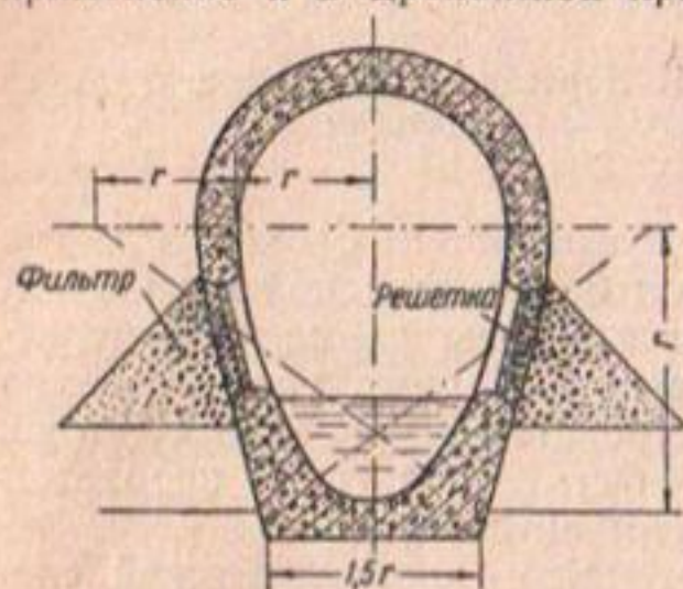
Фиг. 28. Бетонные дренажные трубы овальной формы
