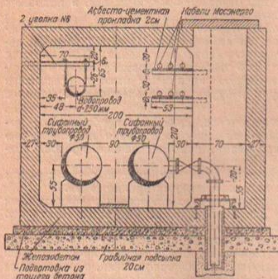
Фиг. 89а. Поперечный разрез по галлее берегового дренажа
