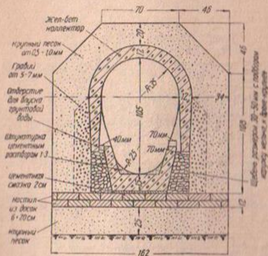
Фиг. 101. Конструкция горизонтальной дрены в местах расположения дренажных отверстий
