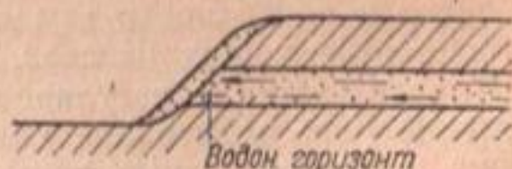
Фиг. 3. Выход грунтового потока в склоне
