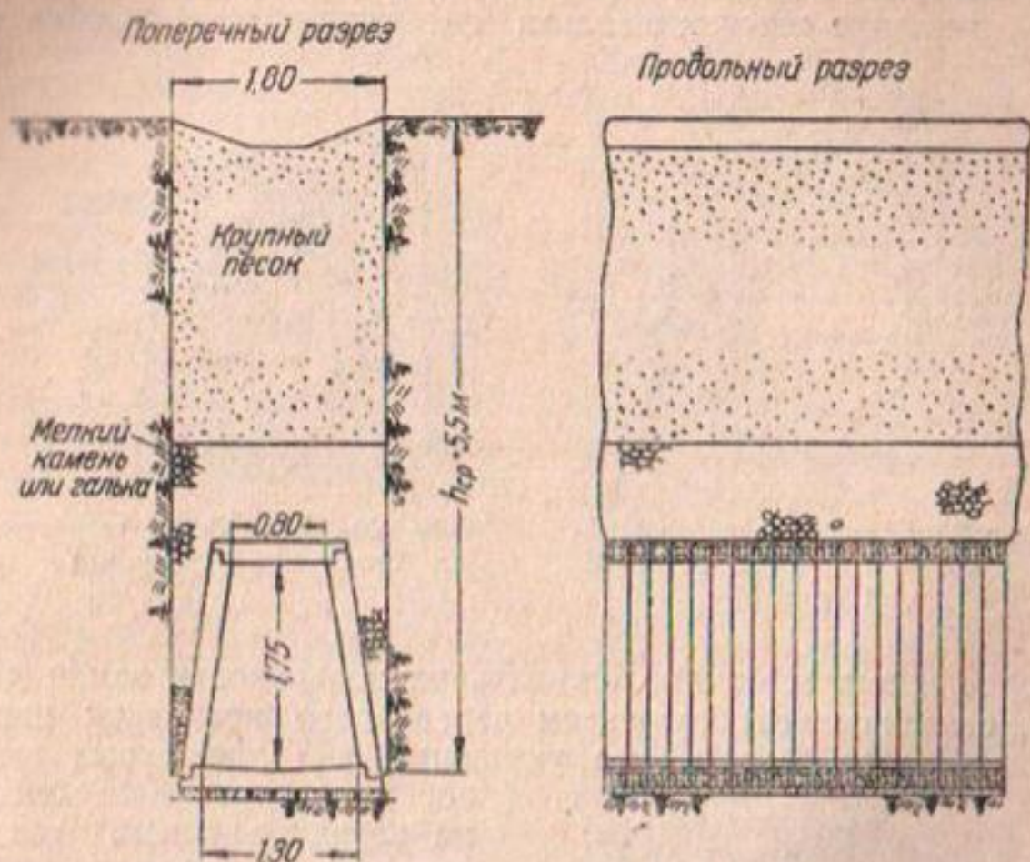
Фиг. 37. Деревянная дренажная галерея
