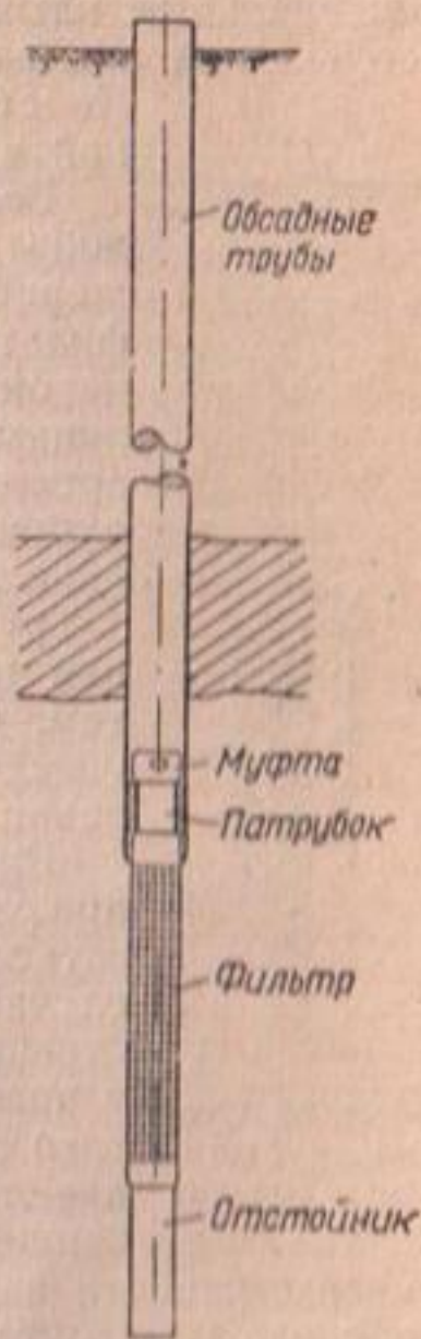
Фиг. 75. Схема трубчатого колодца
