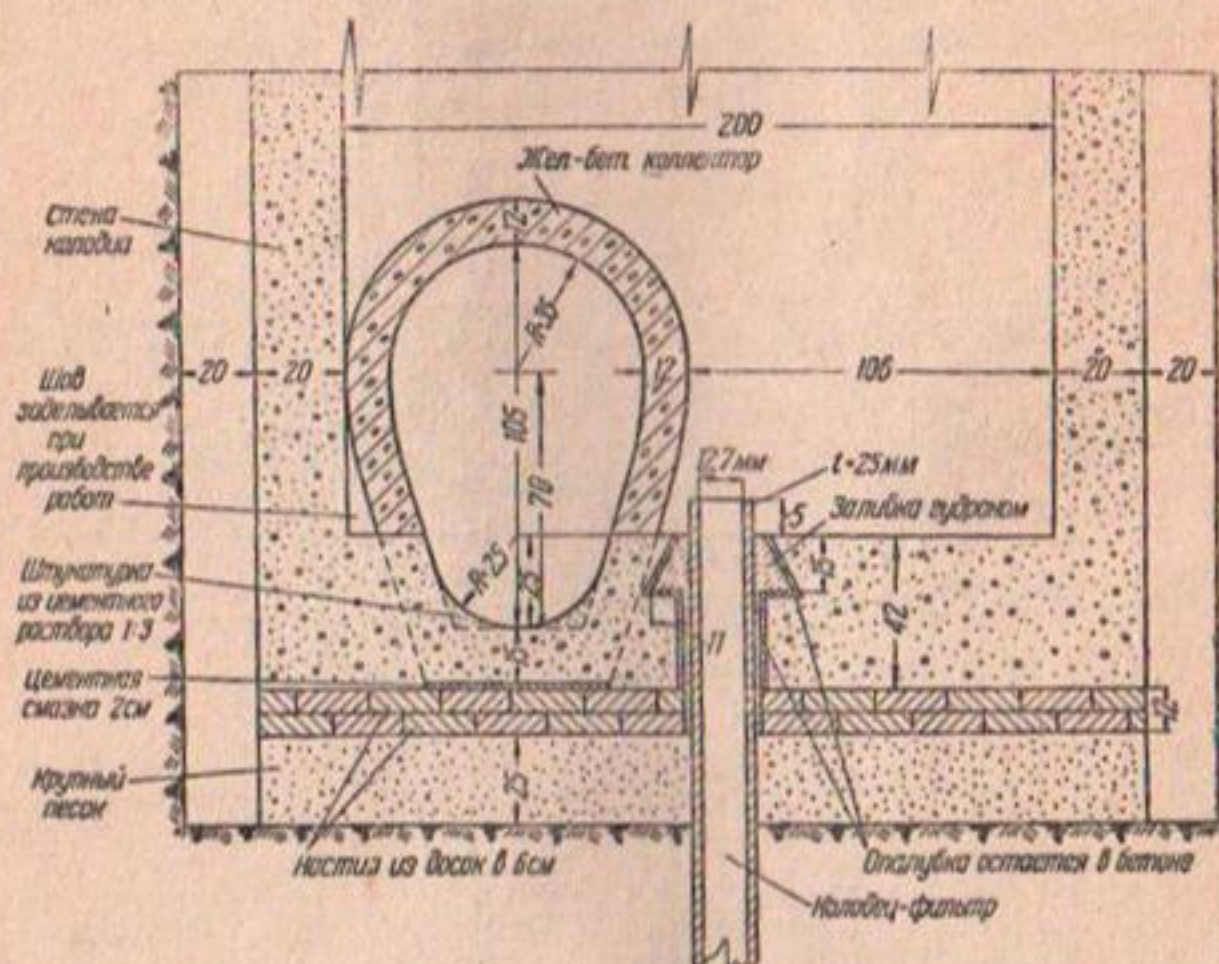
Фиг. 105. Сопряжение вертикальных колодцев с горизонтальной дренай. Деталь.
