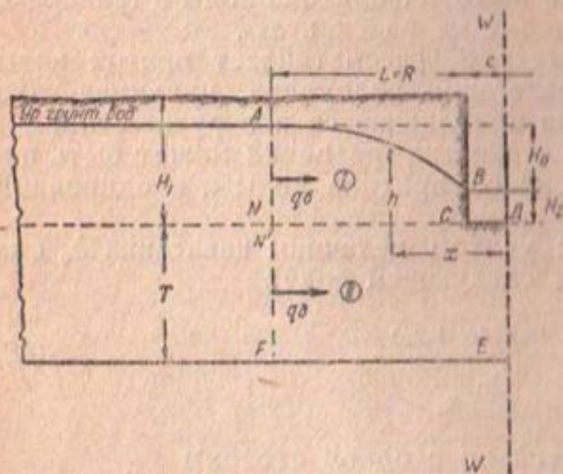
Фиг. 49. Схема притока воды к горизонтальной дрене по Чугаеву
