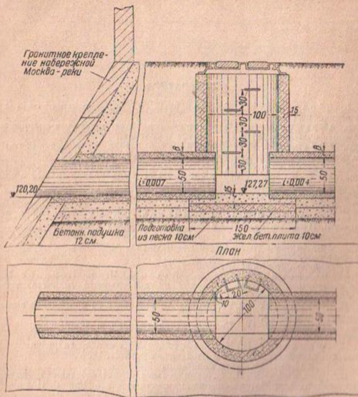
Фиг. 106. Выпуск дренажных вод через стенки набережной
