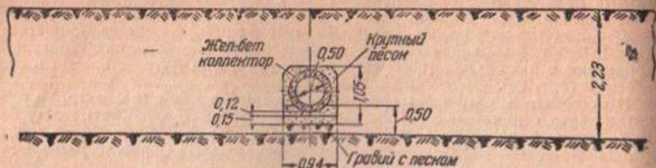
Фиг. 102. Конструкция горизонтальной дрены в пределах сбросной части
