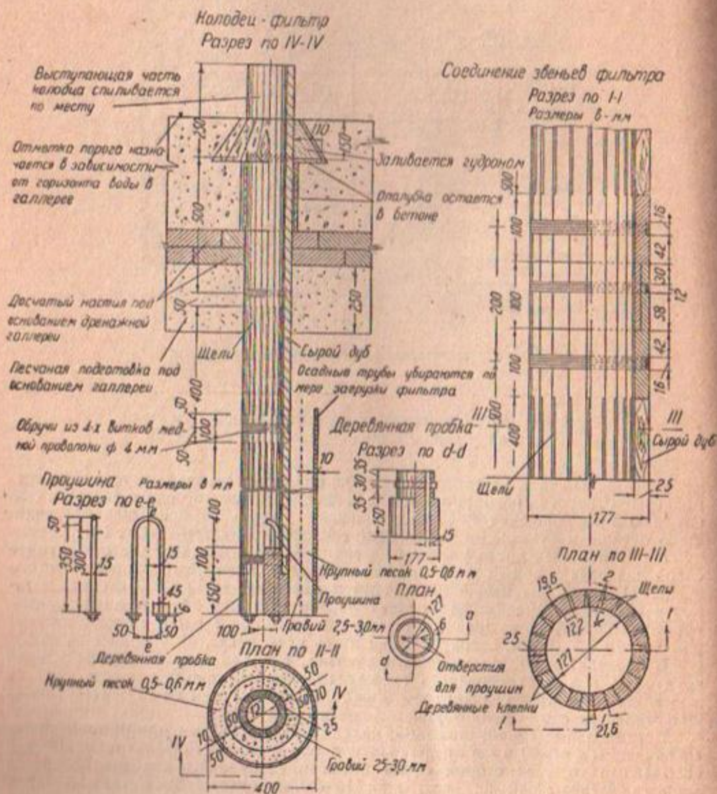
Фиг. 103. Конструкция самонизливающих колодцев
