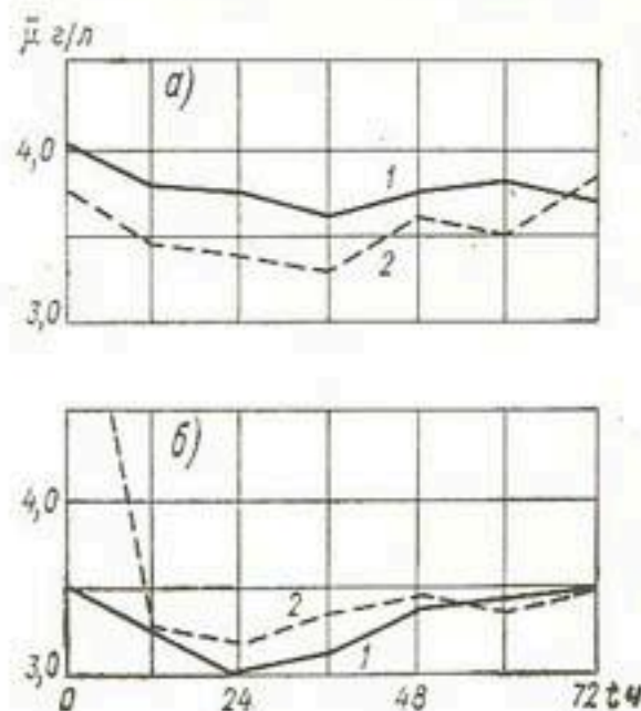
Рис. 25. Достижение предельного режима в опытном полевом канале в Ташаузе в результате заиления (а) и размыва (б).
