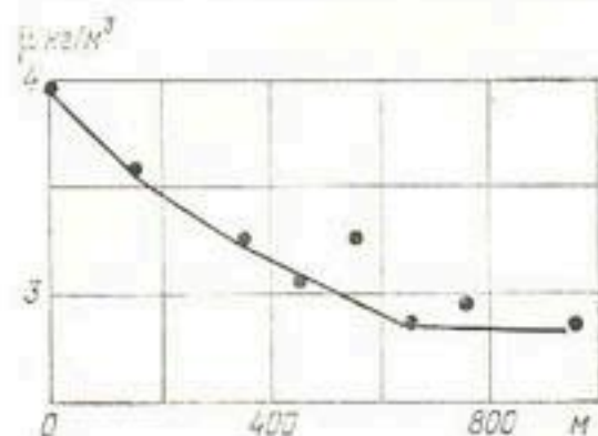
Рис. 58. Динамика заиления в отстойнике Кипчак—Бозсу.
