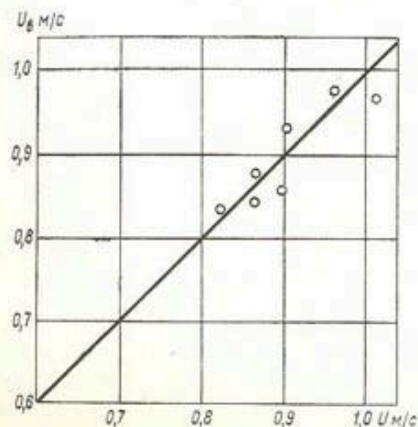
Рис. 32. Опытные и расчетные скорости течения в лотке по опытам Г. А. Тер-Абрамянца.
