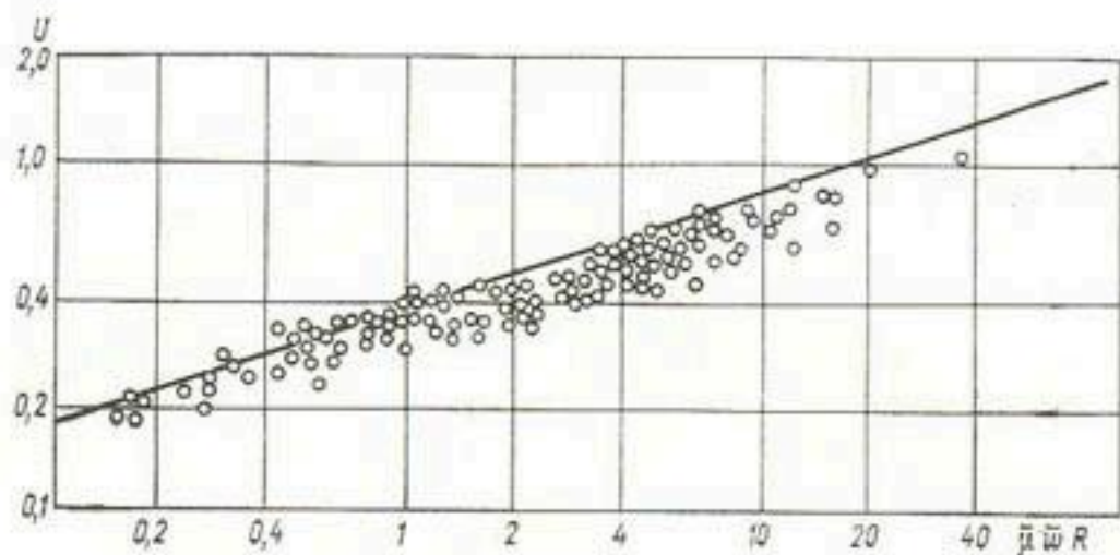
Рис. 27. Заиляющие режимы. Сводный график.
