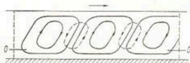
Рис. 5. Схема крупномасштабных пульсаций в отсеке потока.
