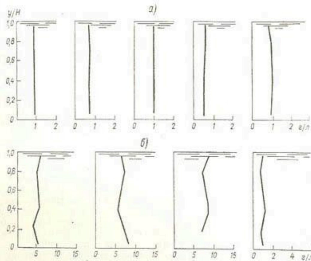
Рис. 44. Распределение взвешенных наносов по глубине. а — мельче 0,01 мм (Амударья), б — мельче 0,05 мм (Вахш).
