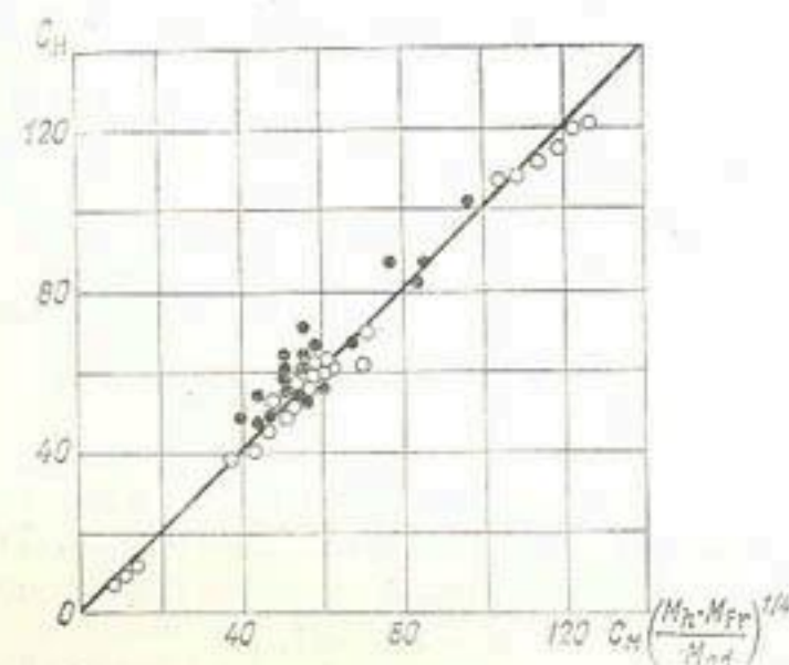
Рис. 61. Коэффициент Шези по данным натурных и модельных наблюдений.
