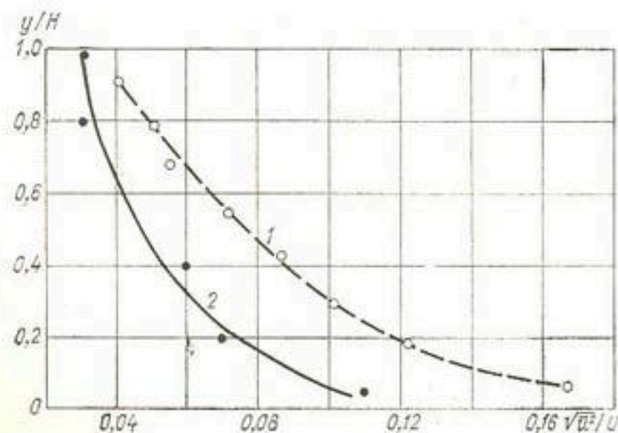
Рис. 37. Изменение отношения дисперсии продольной пульсации к местной осредненной скорости. 1 — в лотке [111], 2 — в реке [48].
