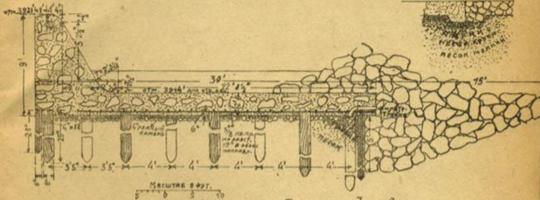
ЧЕРТ. № 15 ПЛОТИНА Ласвику
