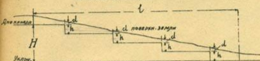
Профиль канала когда необходимы перепады.
