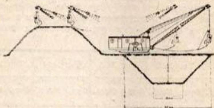
Черт. 33. Схема поперечного передвижения к оси канала ходящего экскаватора.
