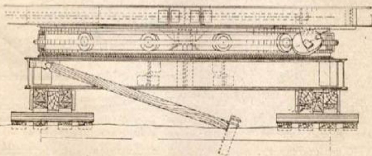
Черт. 29. Разрез хода на катках экскаватора "Бьюсайрус", класс 14, Управление работ в Голодной степи.
