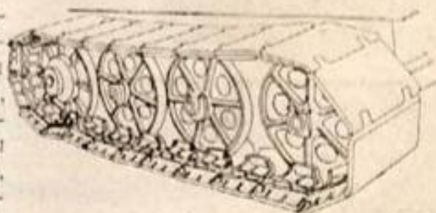
Черт. 27. Гусеничный ход экскаваторов „Бьюсайрус“.
