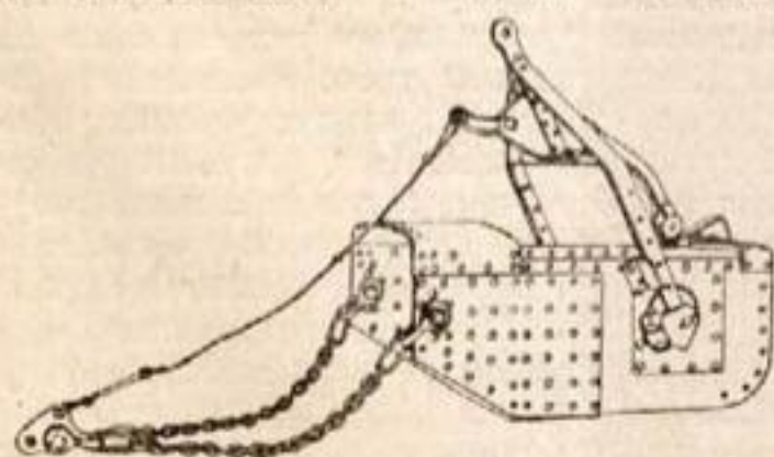
Черт. 21. Ковш системы „Monighan“ со стальным козырьком для легких грунтов.
