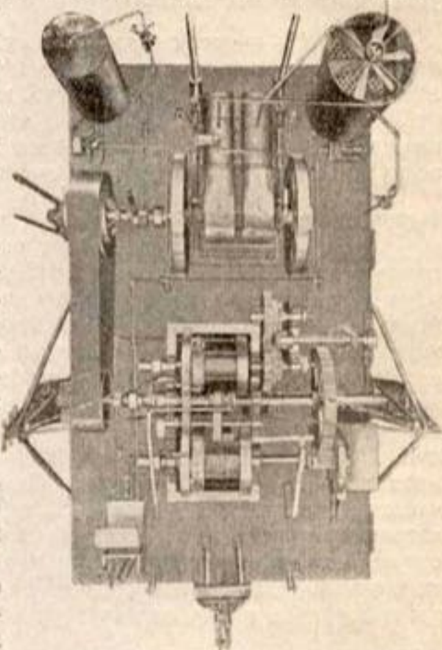
Фот. 17. Расположение механизмов экскаватора внутреннего сгорания системы „Monaghan“.
