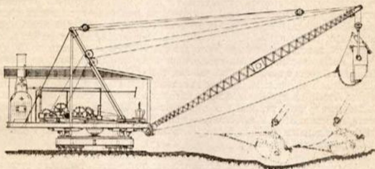
Черт. 28. Фасад парового экскаватора на катках.
