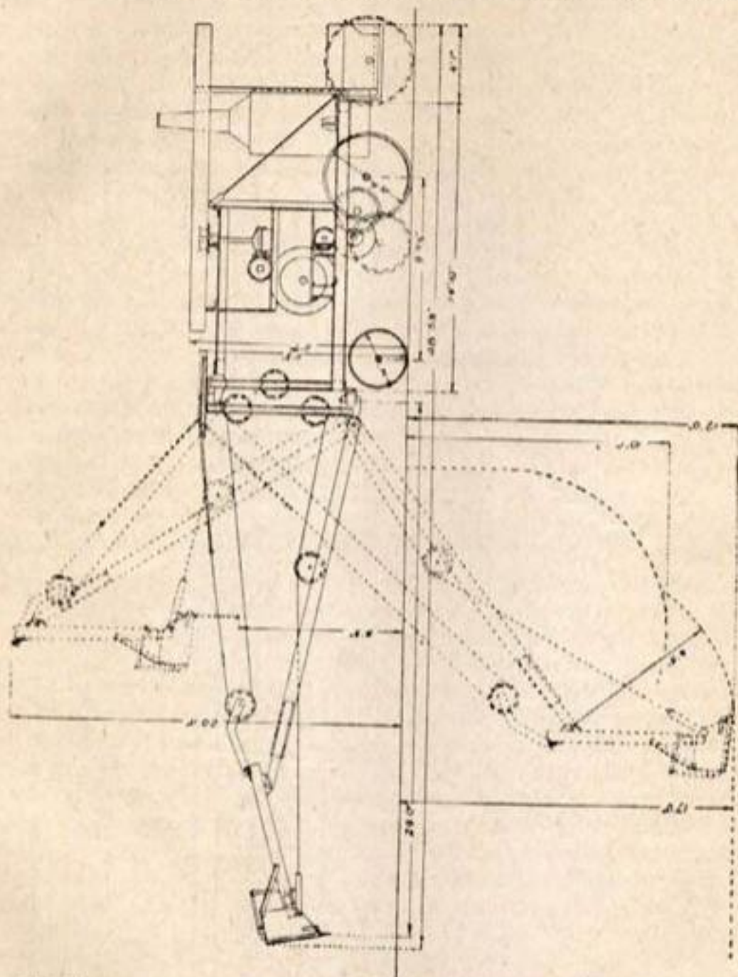
Черт. 37. Схема экскаватора системы „Кистон“ с рычажным приспособлением для выемки узких траншей.
