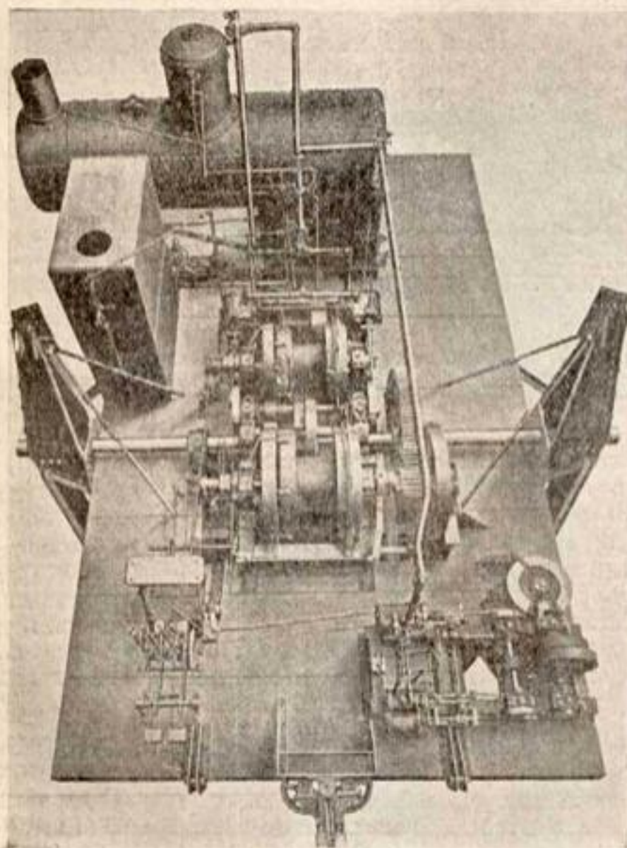
Рис. 13. Общее расположение механизмов парового экскаватора системы Монигли.
