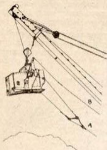
Черт. 22. Ковш системы „Iverson“ с отдельными троссами: тяговым для набора грунта и для опрокидывания.
