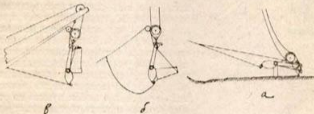
Черт. 24. Ковш системы „Dunbar“ быстрого наполнения с дверцей против высыпания грунта. а) Наполнение черпака, б) под'ем наполненного черпака, в) опорожнение черпака.
