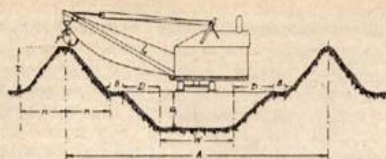
Черт. 34. Схема предельных размеров канала разрабатываемого различного типа скреперными экскаваторами.
