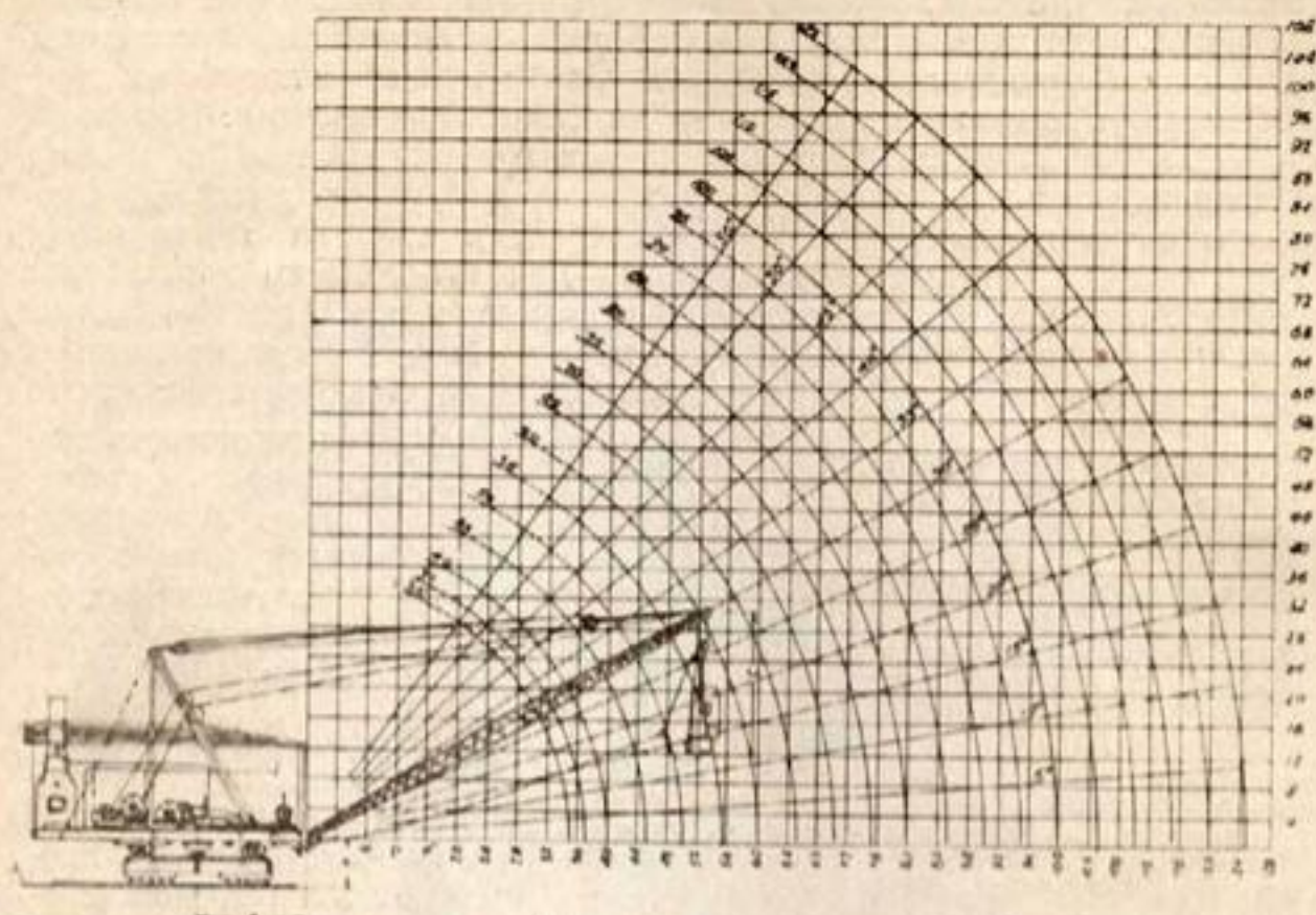
Черт. 26. Диаграмма для определения радиуса действия и предельной высоты кавальера для экскаваторов системы „Monaghan“, для различных типов снарядов и различных углов наклона стрелы.
