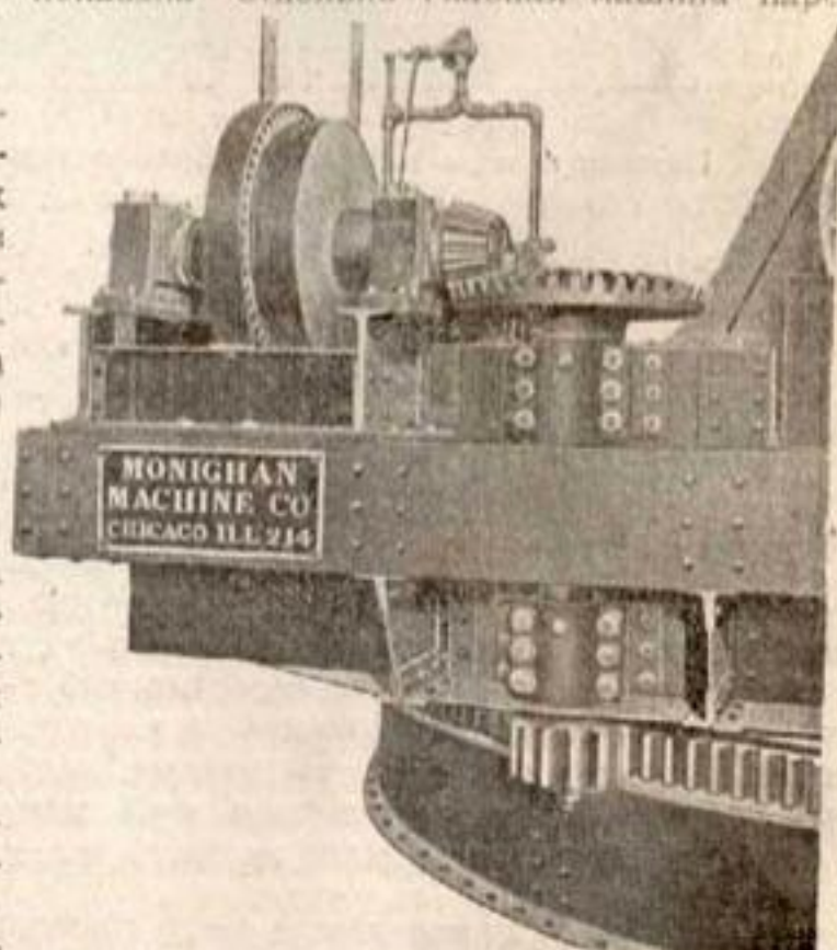
Рис. 15. Поворотный механизм экскаватора системы „Monighan“. Наверху вверху видна вращающаяся машина, показанная отдельно на рис. № 16.
