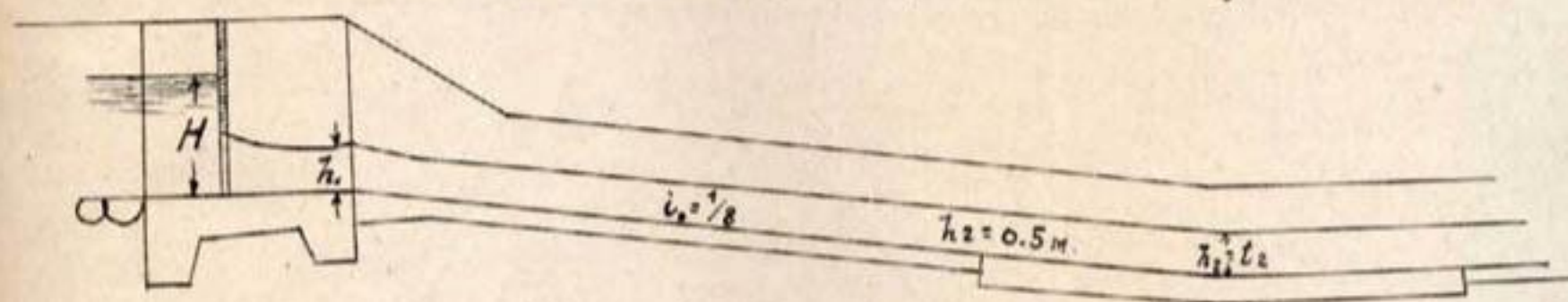
ЧЕРТ. 1. БЫСТРОТОК ПОСТОЯННОГО СЕЧЕНИЯ
