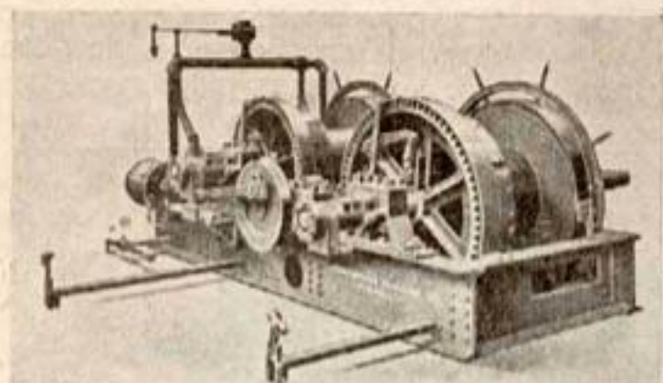
Рис. 14. Главная машина парового экскаватора системы „Monighan“.
