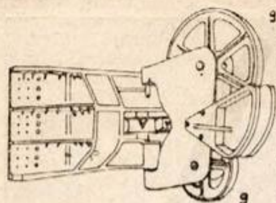
Черт. 25. Универсальные направляющие устройства для тягового тросса.
