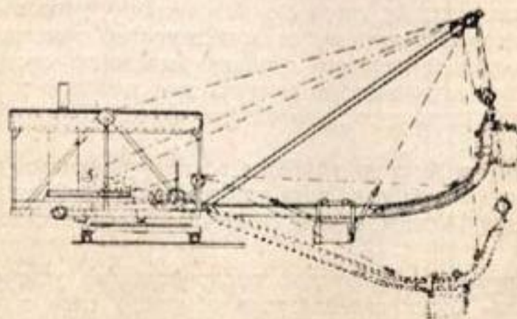
Черт. 35. Схема экскаватора Джекобса с жестким направлением ковша.
