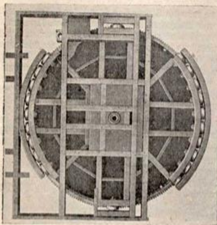
Рис. 18. Поворотные части и роликовые тележки экскаватора системы „Monighan“.
