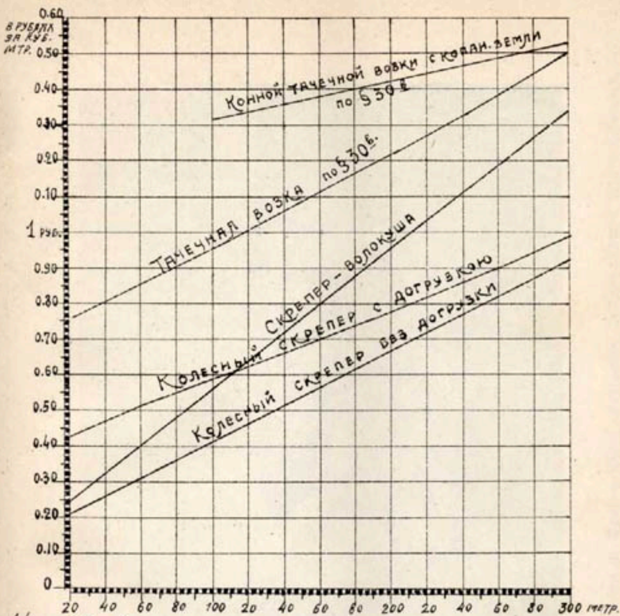
Черт. 18. Диаграмма расценок земляных работ скреперами с распахиванием грунта и для копаний по § 30 а Урочн. Полот. для различных дальностей возки.
