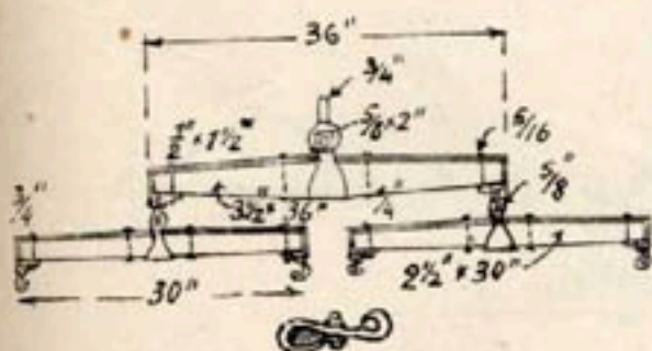
Черт. 17. Упражные приспособления скреперов Фресно.
