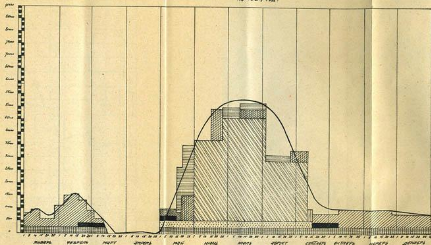
ГРАФИК РАСХОДА ВОДЫ В ГОЛОВЕ МАГИСТРАЛЬНОГО КАНАЛА Благодно-Ступской оросительной системы согласно заявкам водопользователей на 1924 год.
