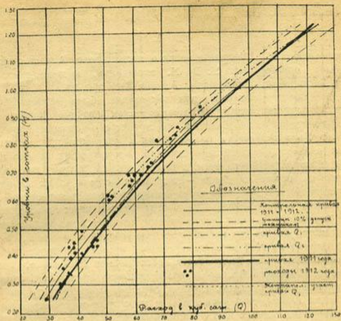
Черт 2. Река Или. Ст. Илийская
