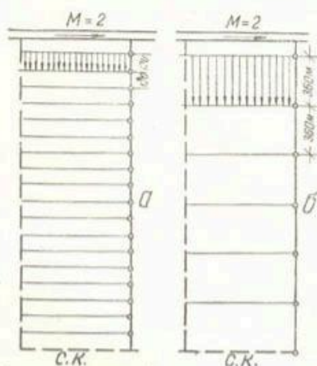
Рис. 3. Схема нарезки временных оросителей на полевых участках. а—спроектированные оросители, б—оросители, работавшие в 1961 г.
