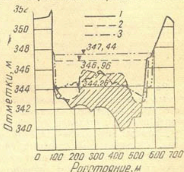
Рис. 6. Совмещенный поперечный профиль Кайраккумского водохранилища по створу 8: 1 — 1955; 2 — 1958; 3 — 1960 г.
