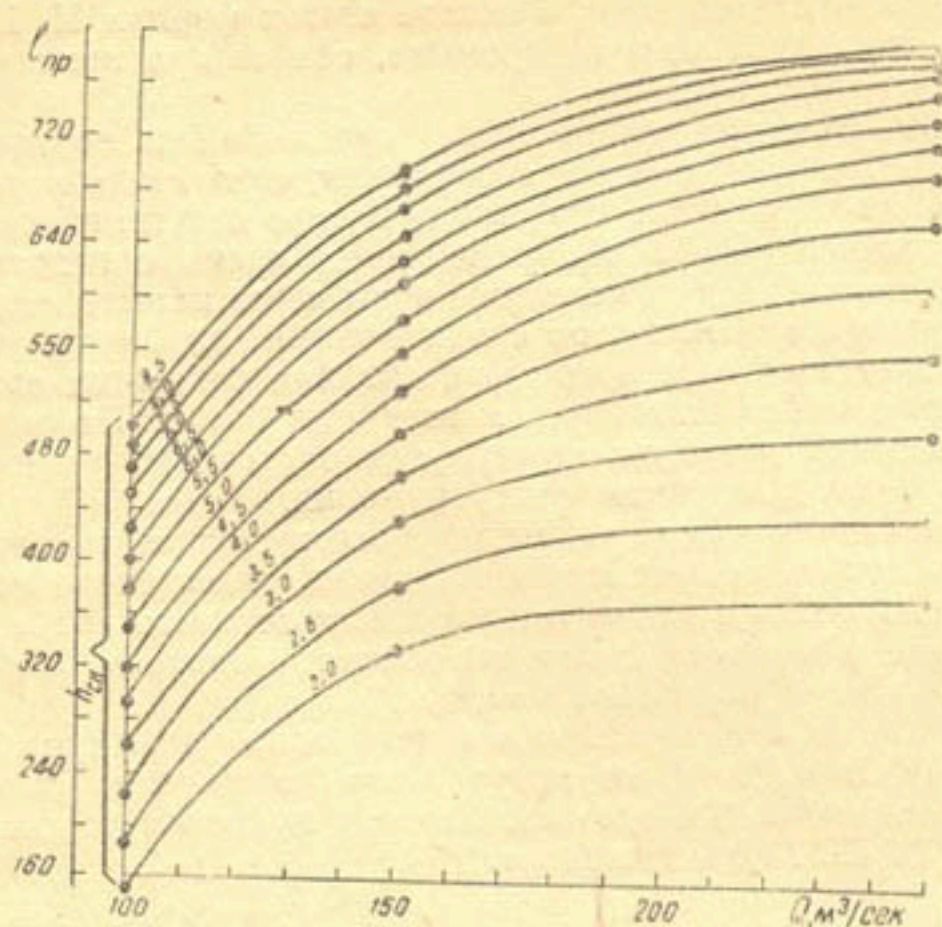
Рис. 4. График зависимости l_{\text{пр}} = f(Q_p, h_{\text{ст}}) .
