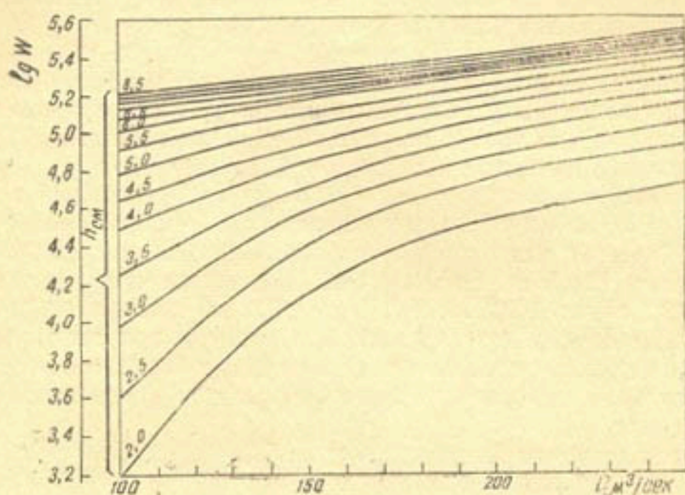
Рис. 3. График зависимости \lg W = f(Q_p, h_{сн}) .
