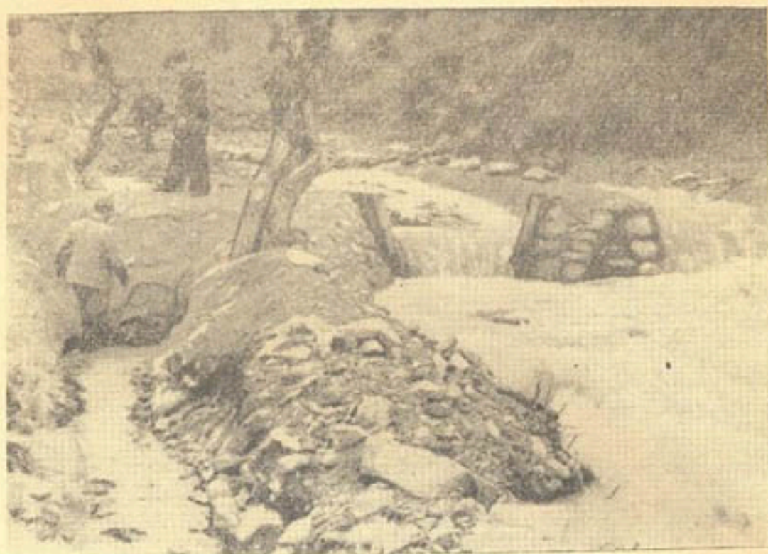
Рис. 4. Вид с нижнего бьефа на бассейн по измерению воды и наносов.
