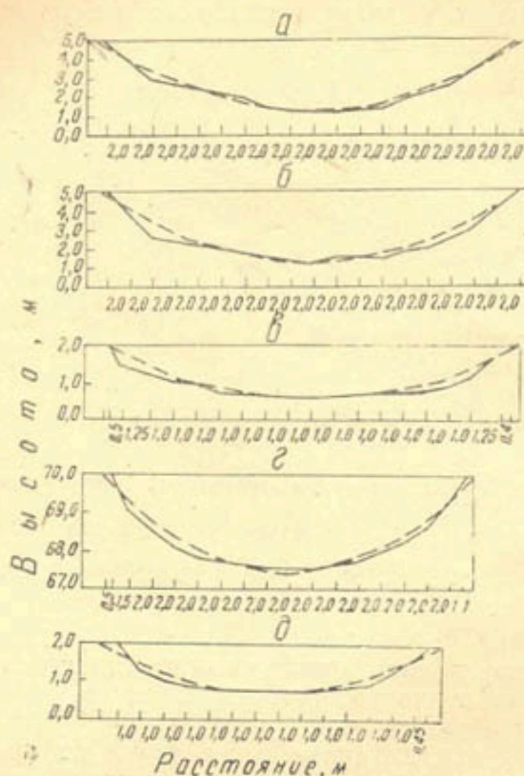
Рис. 2. Сопоставление натуральных поперечников с теоретическими на каналах:
