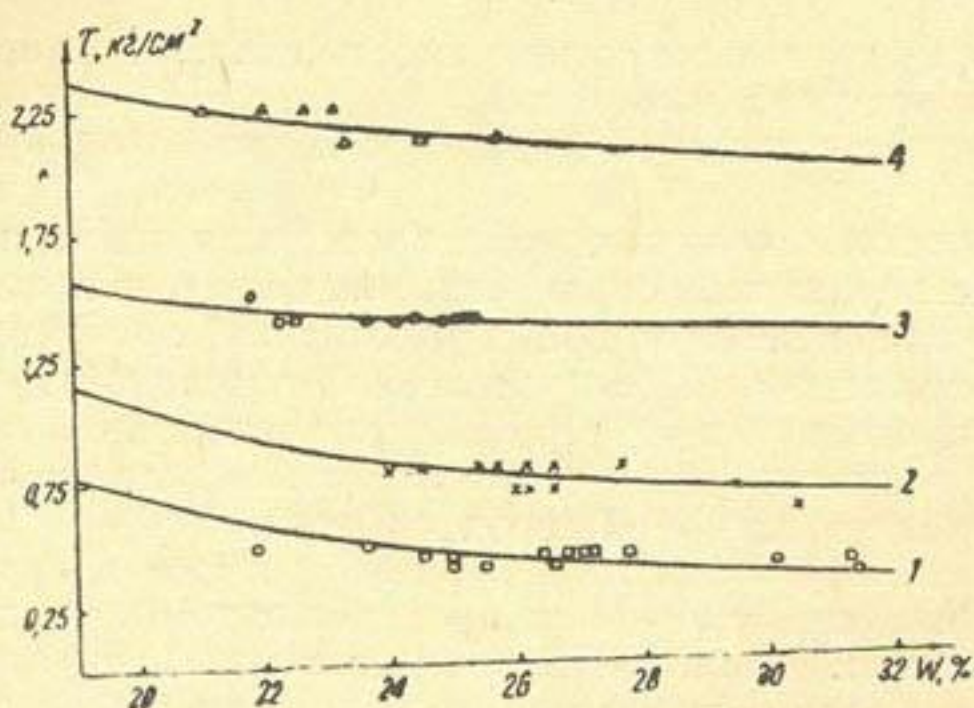
Рис. 1. График зависимости сопротивления грунтов сдвигу от влажности при различных нормальных давлениях. P равно:
