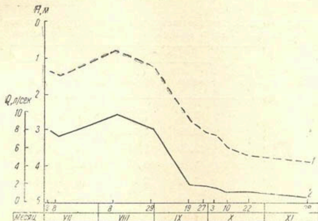
Рис. 4. Колебания уровня грунтовых вод и притока воды к дренаю 5-1-Д-53:
