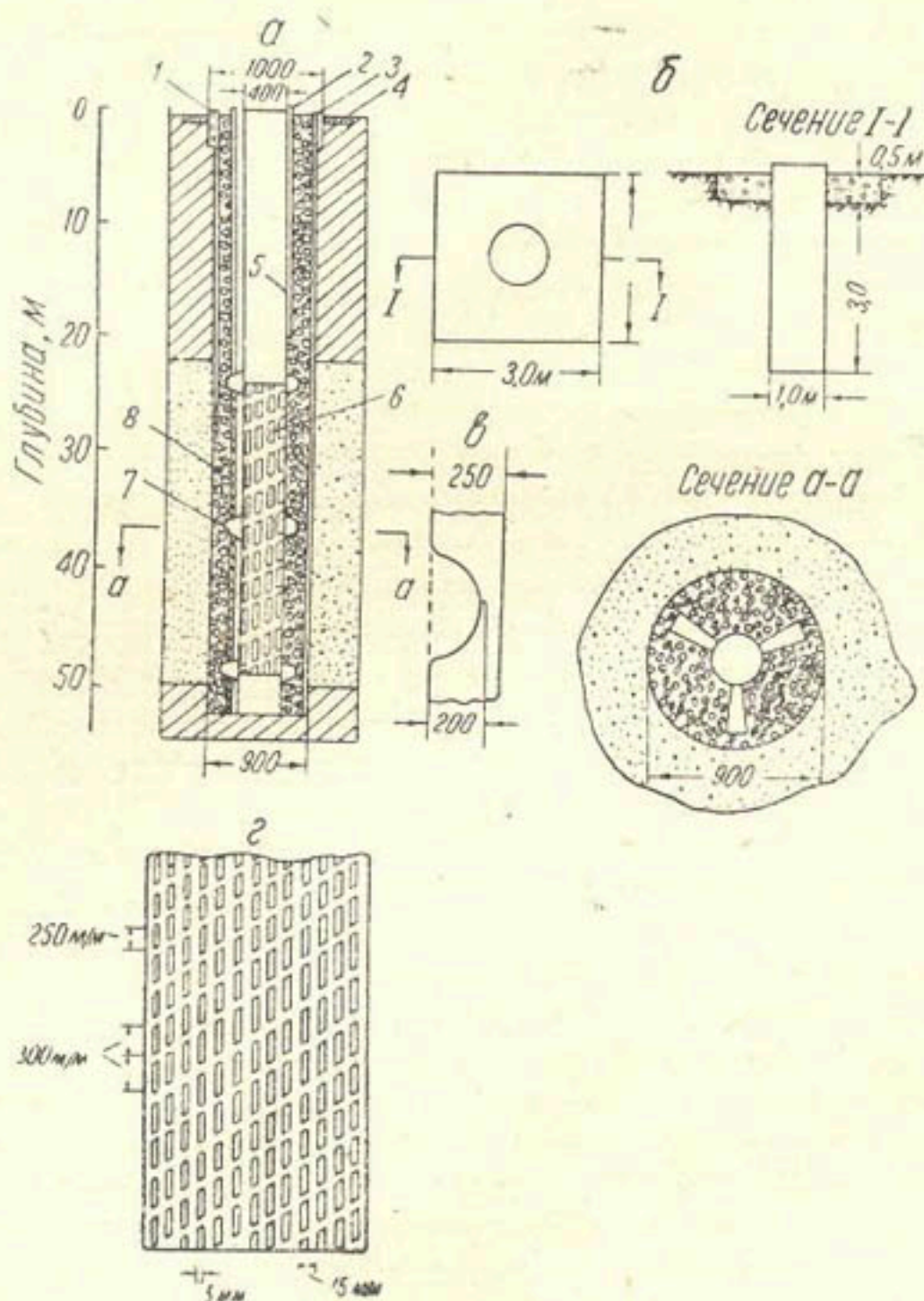
Рис. 1. Типовая конструкция скважины:
