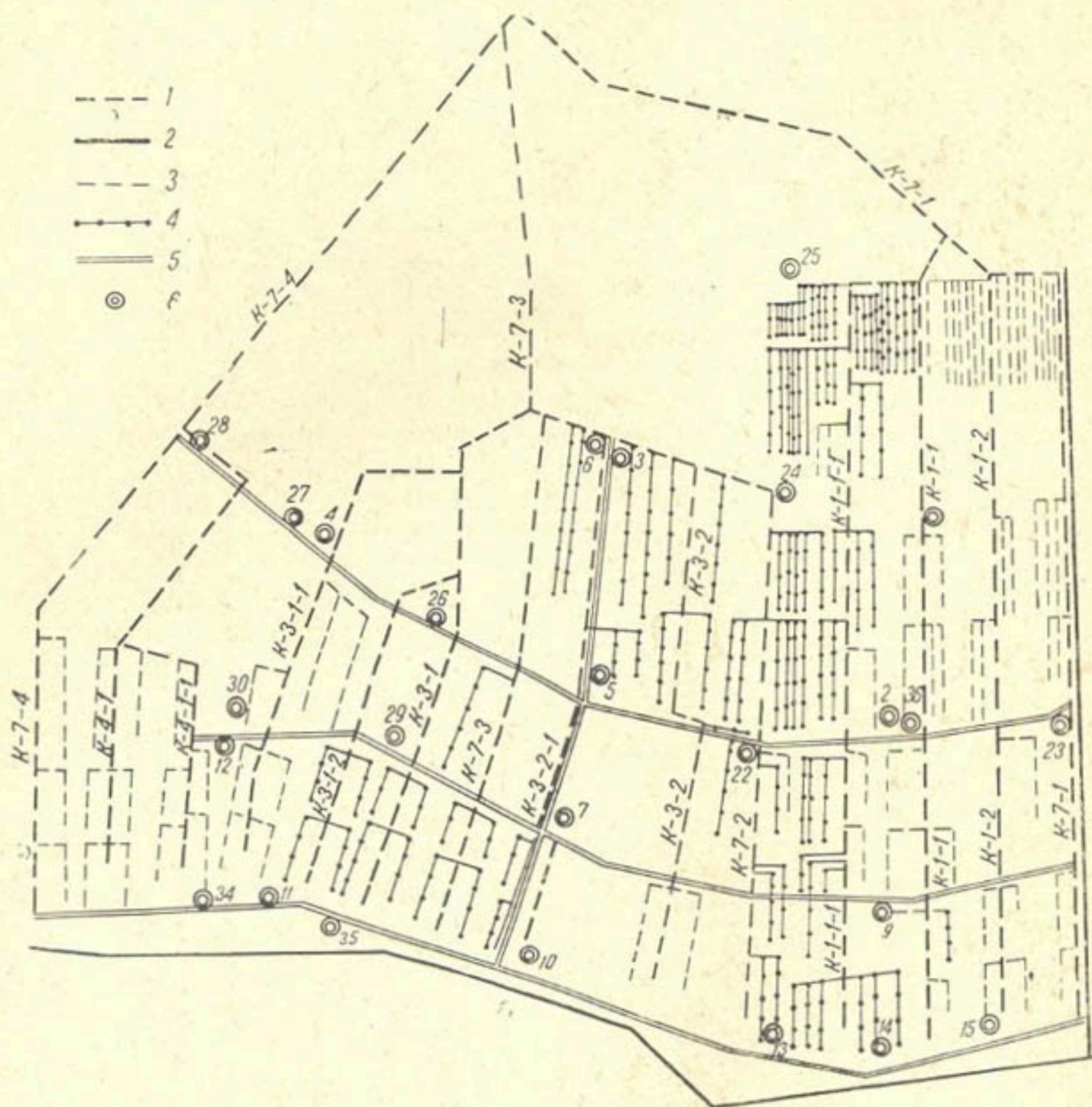
Рис. 1. Схема коллекторно-дренажной сети по совхозу № 5 на октябрь 1963 г.: 1 — открытые коллекторы; 2 — канал; 3 — открытые дрены; 4 — закрытые дрены; 5 — дороги; 6 — скважины.
