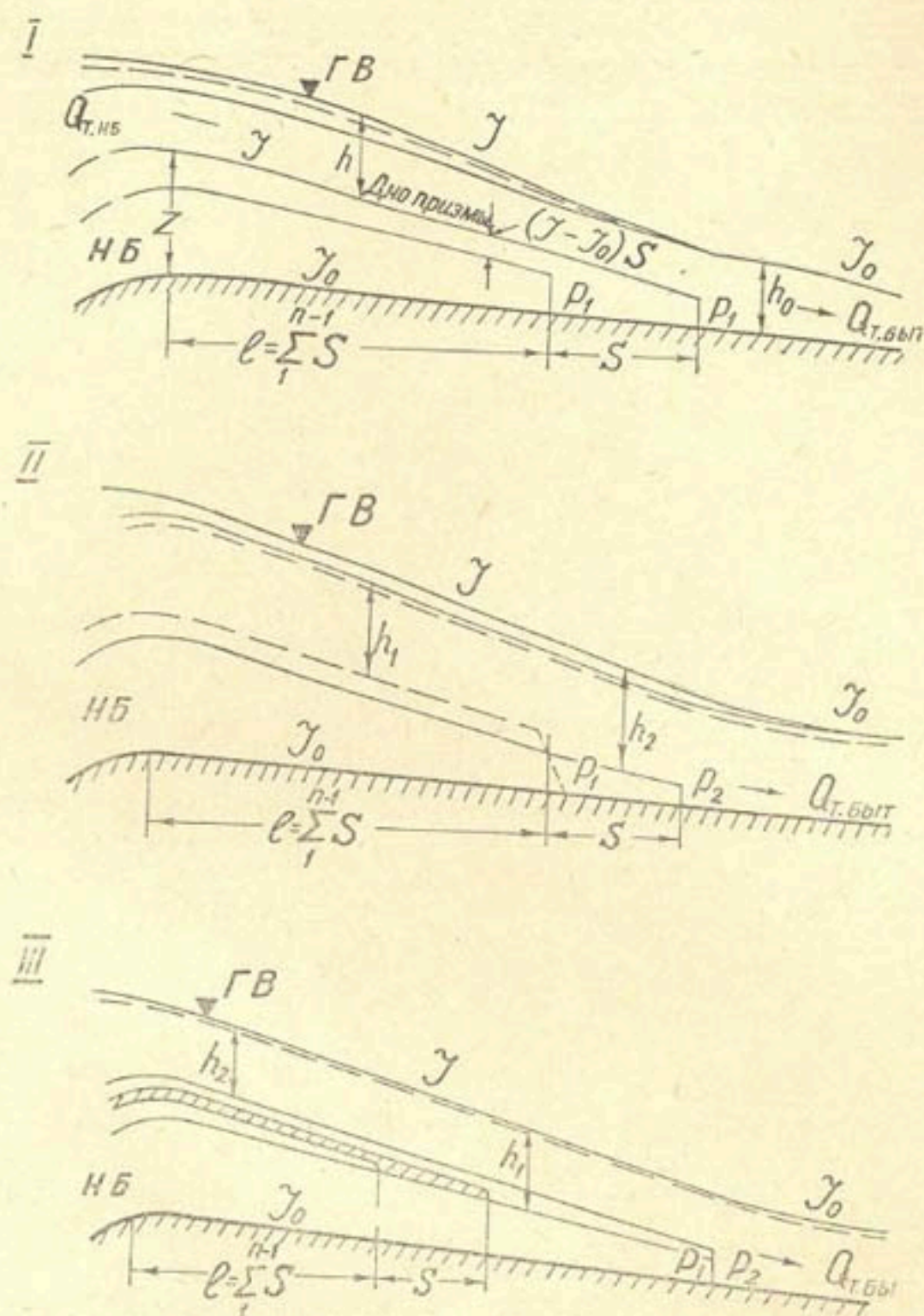
Рис. 3. Схемы занесения нижнего бьефа в зависимости от изменения расхода воды.
