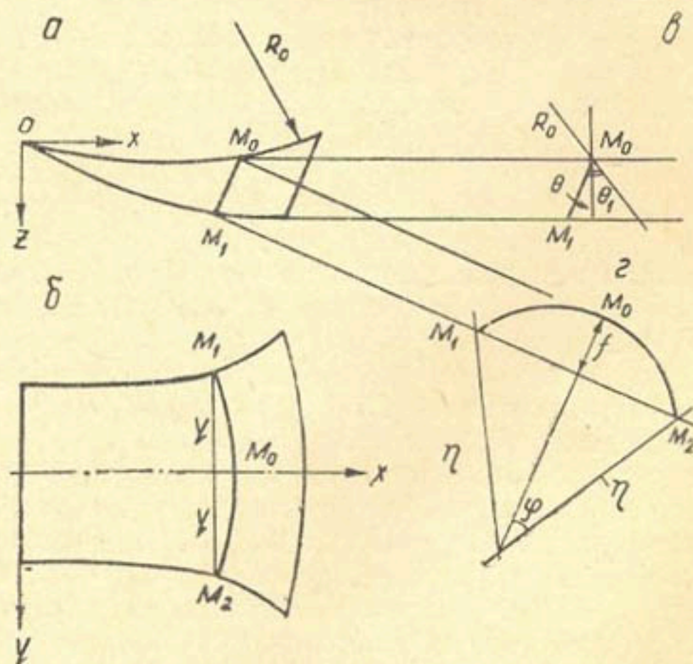
Рис. 2. План и разрезы рассеивающего трамплина.
