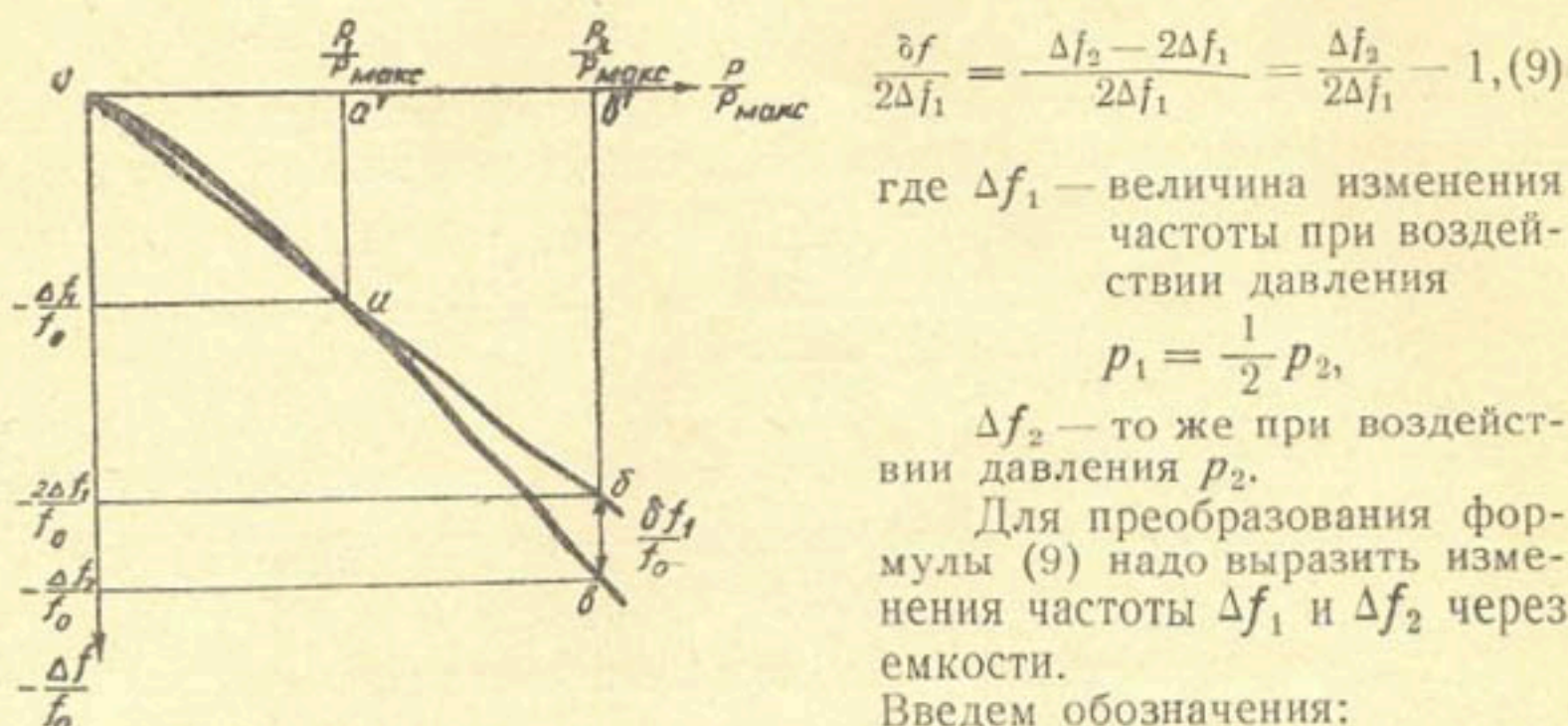
Рис. 2. Построения для определения погрешности измерения.
