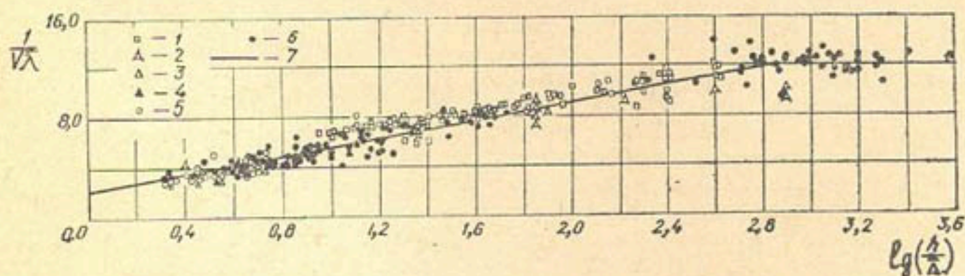
Рис. 4. График зависимости \frac{1}{\sqrt{\lambda}} = f\left(\frac{H}{\Delta}\right) .
