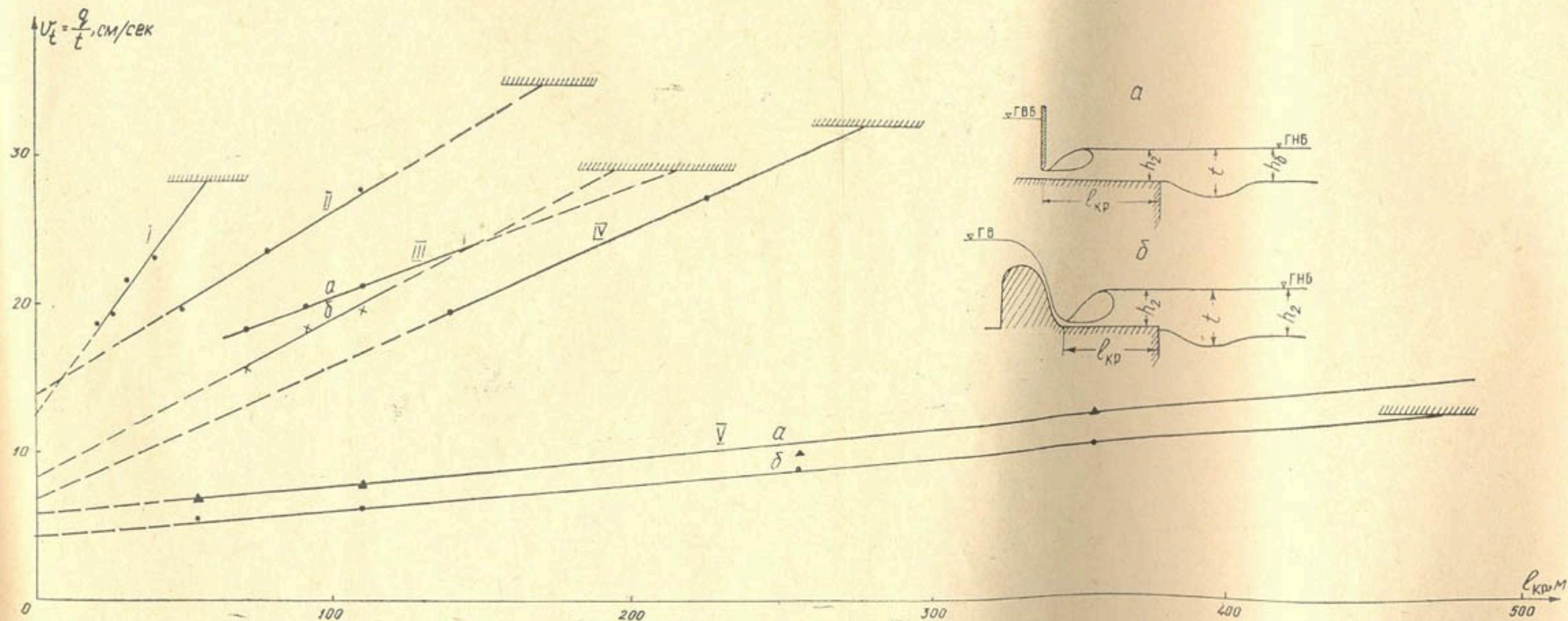
Рис. 2. График зависимости V_t от длины крепления.
