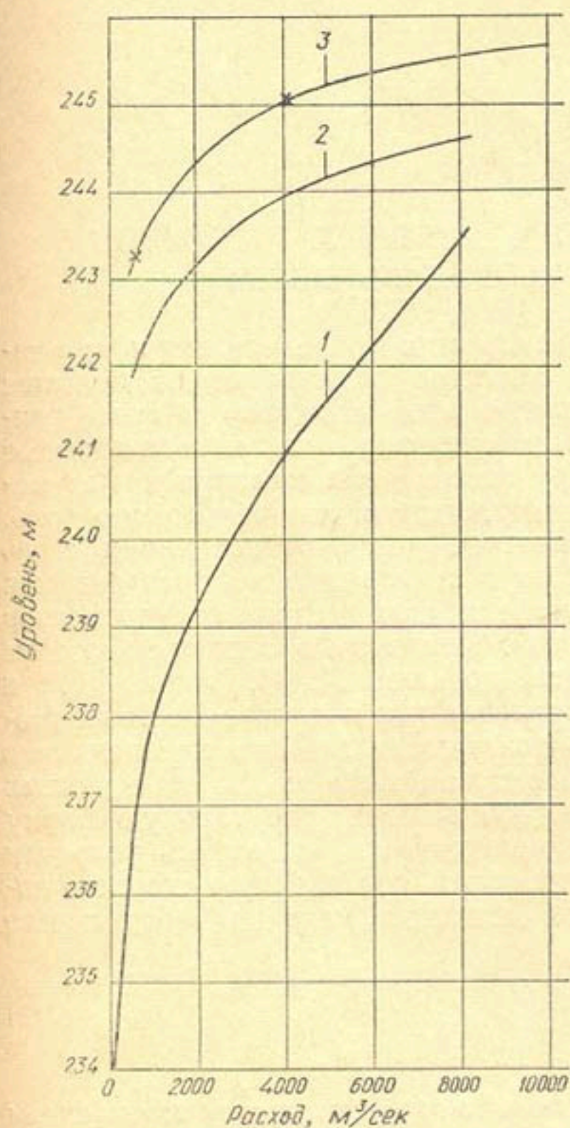
Рис. 5. Графики изменения уровня в бытовых условиях после общего размыва и занесения русла в нижнем бьефе в зависимости от расхода воды.
