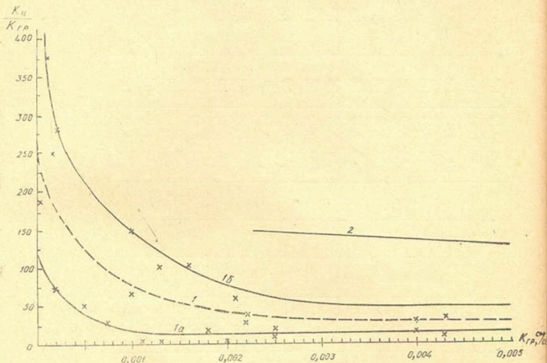
Рис. 2. График зависимости \frac{K_{\text{ц}}}{K_{\text{гр}}} = f(K_{\text{гр}}) для подбора фильтра из пористого бетона.
