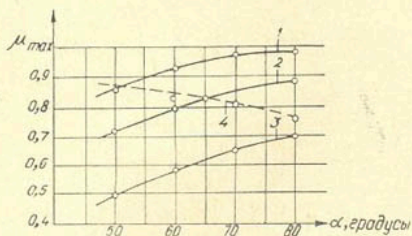
Рис. 4. График изменения максимальных коэффициентов расхода конусных затворов \mu_{\max} = \Phi = f\left(\alpha^\circ; \frac{A}{D}\right) для \alpha = 50, 60, 70 и 80^\circ .
