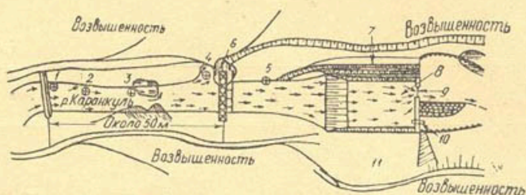
Рис. 1. Схема расположения опытного участка на реке Каранкуль.
