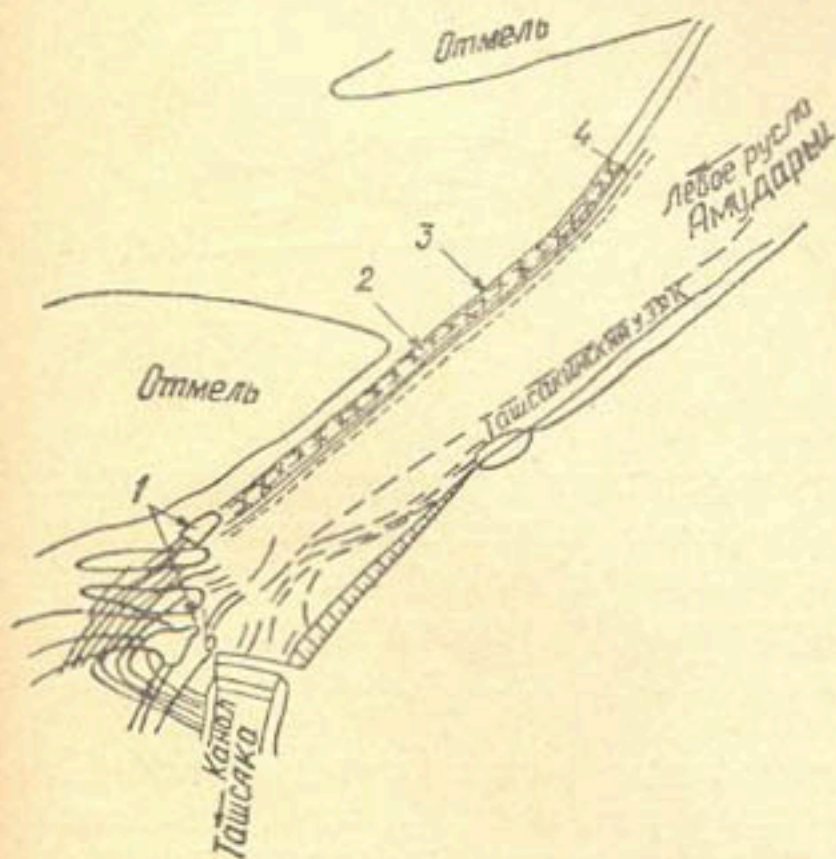
Рис. 2. План шпоры перед Ташсакинским головным сооружением (1948 г.).
