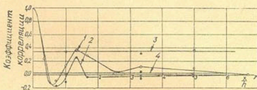
Рис. 2. График изменения коэффициента корреляции пульсационных составляющих скорости бурного потока с большой относительной шероховатостью.
