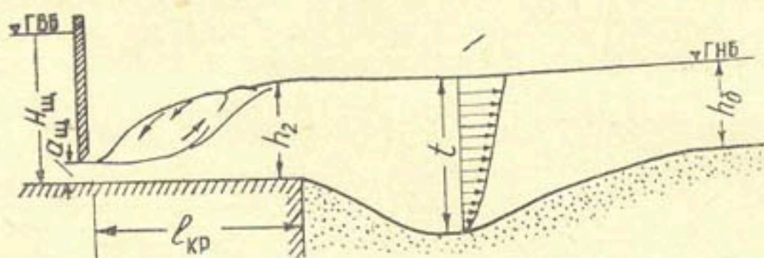
Рис. 1. Гидравлическая схема опыта.
