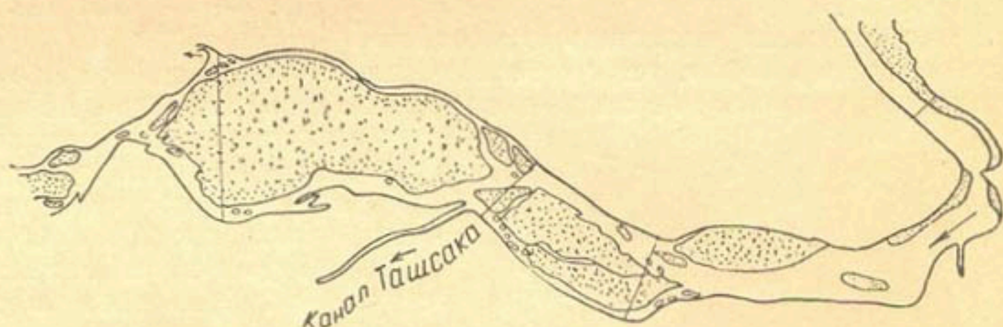
Рис. 4. План участка русла длиной в 35 км от Туямуюна до Октябрьсака (1957 г.).
