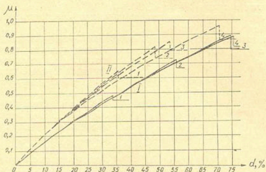
Рис. 2. График изменения коэффициентов расхода конусных затворов.
