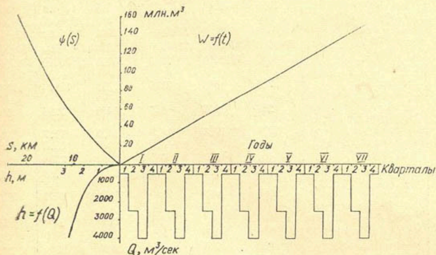
Рис. 4. Прямоугольная координатная система, включающая графики изменения стока наносов, глубины потока и длины призмы отложения в зависимости от гидрографа реки в нижнем бьефе (после водозабора).
