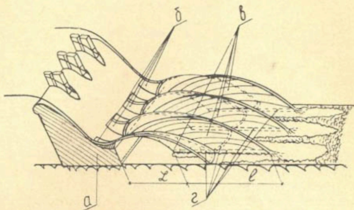
Рис. 1. Схема устройства группы рассеивающих носков на сливной поверхности плотины.
