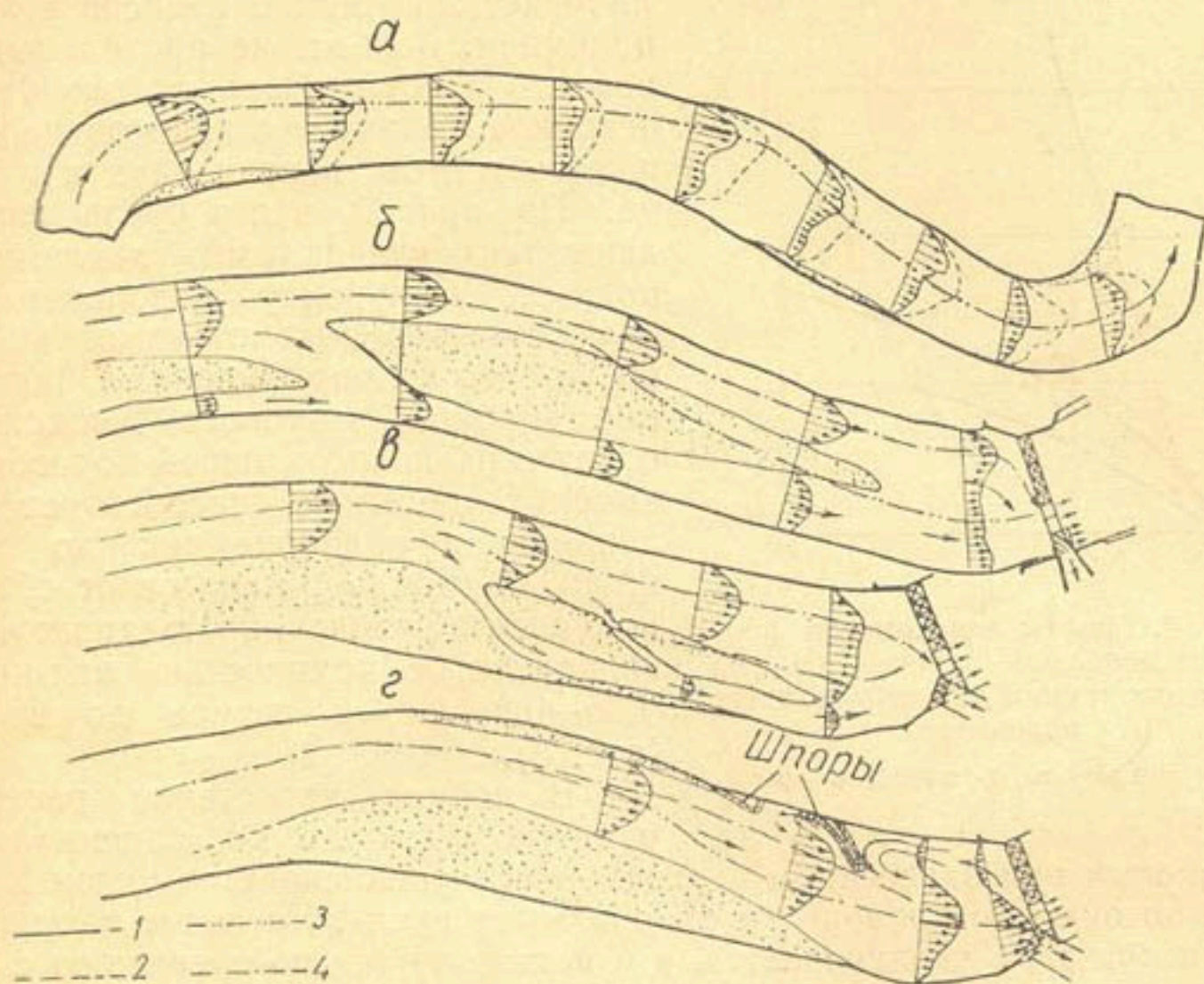
Рис. 2. Планы участка реки перед гидроузлом и эпюры скоростей.
