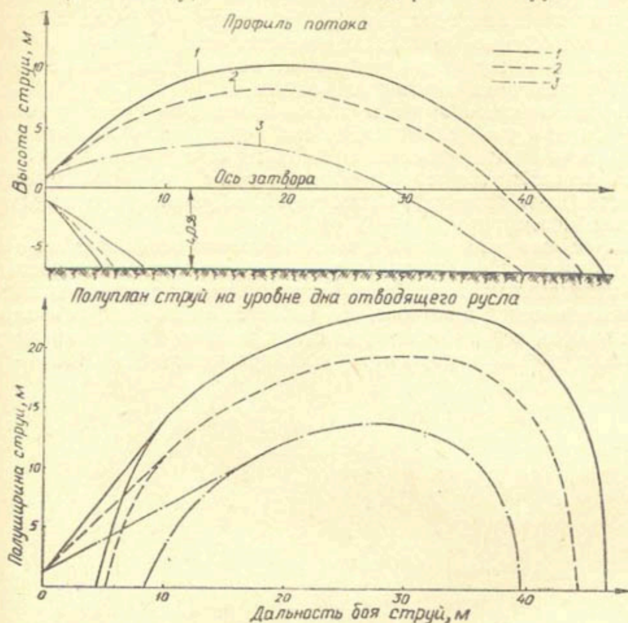
Рис. 5. Формы струй для конусных затворов разных конструкций в применении к параметрам водовыпуска Пачкамарского водохранилища ( \alpha=50\% , H_0=26,58 м, Q=28,2 м 3 /сек).
