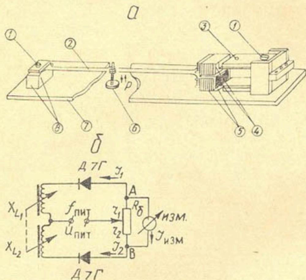
Рис. 5. Схемы индуктивного датчика давления.
