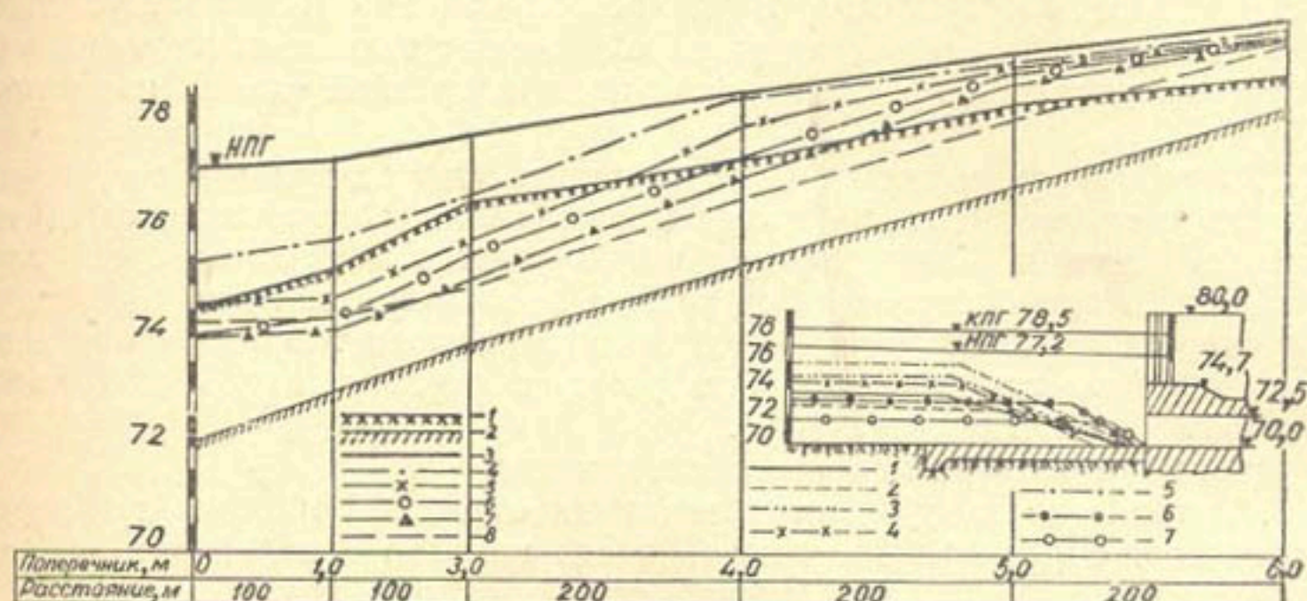
Рис. 4. Продольные профили верхнего бьефа во время промыва при Q = 400 м³/сек.
