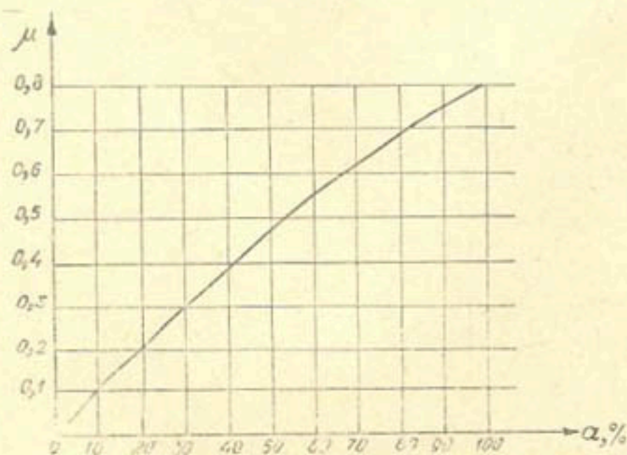
Рис. 6. График изменения коэффициентов расхода конусного затвора ( \mu = f(\alpha) для \alpha=70^\circ ) и безвакуумного очертания кромок неподвижного патрубка.
