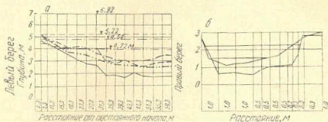
Рис. 3. Совмещенные поперечные профили рек.
