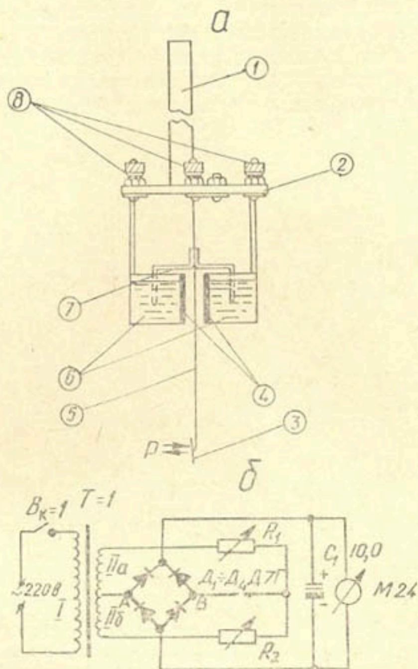
Рис. 6. Схемы датчика-индикатора границы противоположных токов потока.
