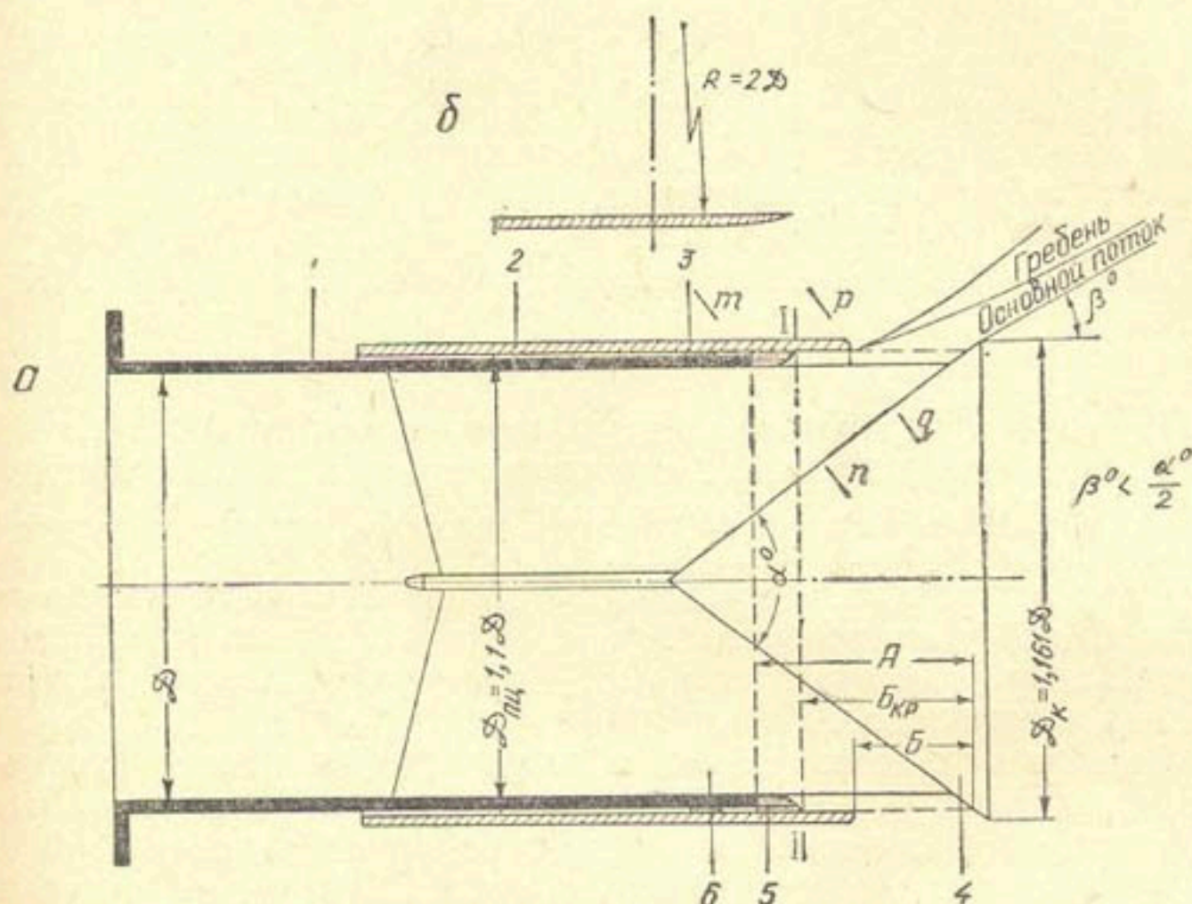
Рис. 1. Схема конусного затвора. a — выходная кромка неподвижного патрубка вакуумного очертания, b — безвакуумного.
