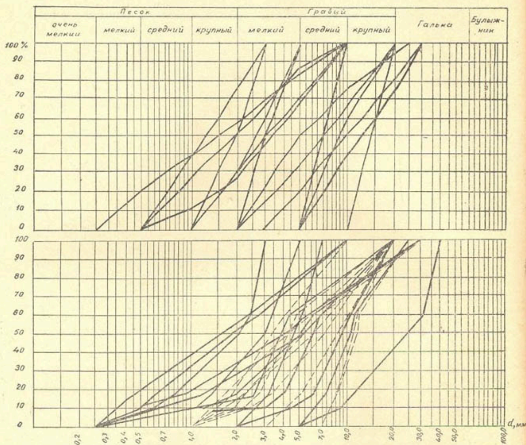
Рис. 4. Подбор состава заполнителей с учетом их формы.
