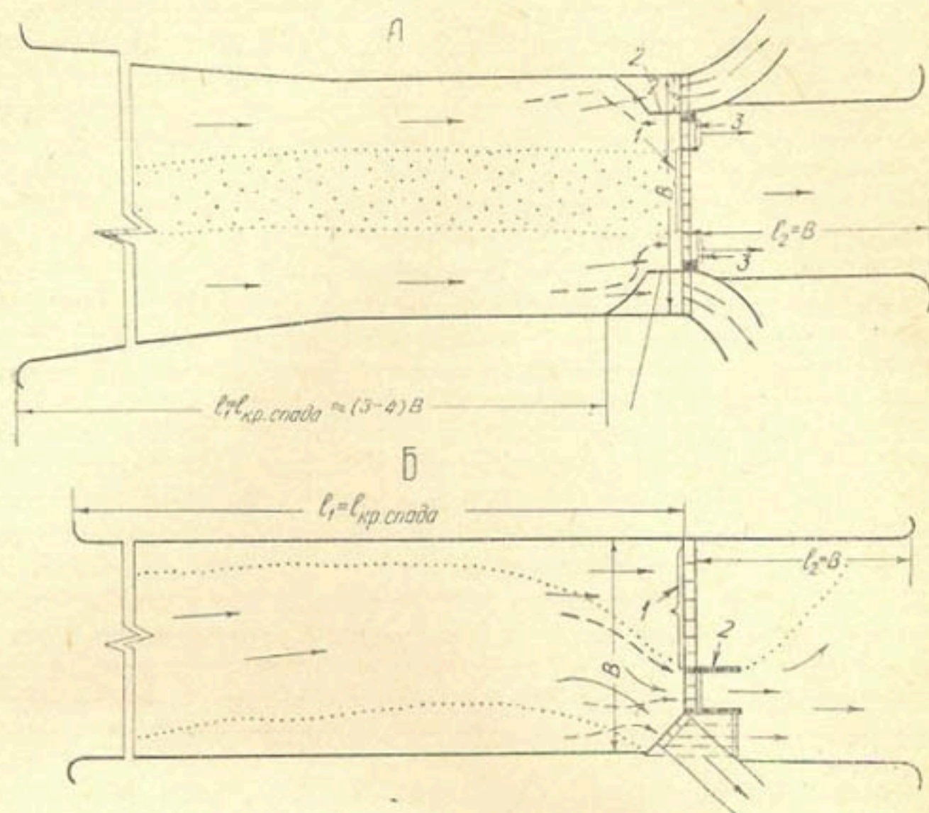
Рис. 4. Рациональные схемы гидроузлов.
