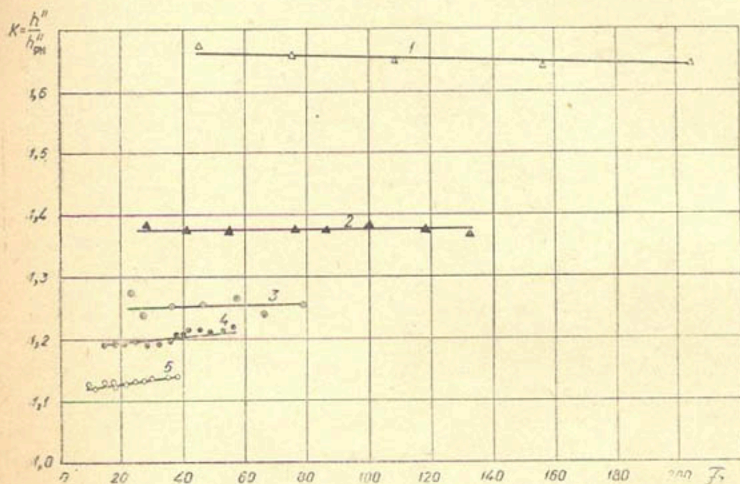
Рис. 3. Зависимость уменьшения сопряженной глубины гидравлического прыжка от числа Фруда.
