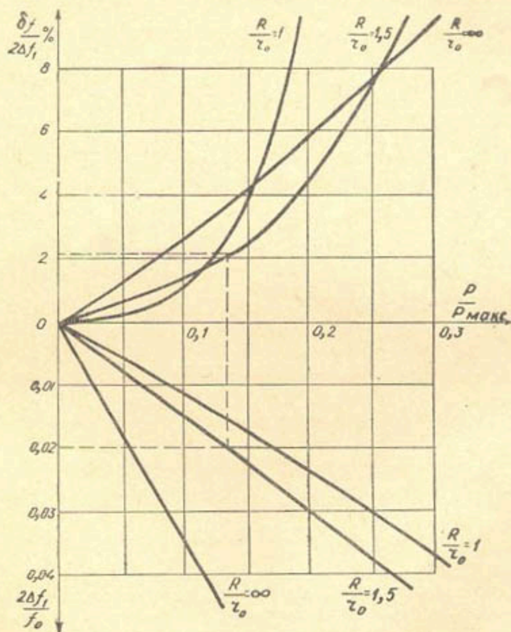
Рис. 3. Кривые отклонения частоты и погрешности в зависимости от измеряемого давления.
