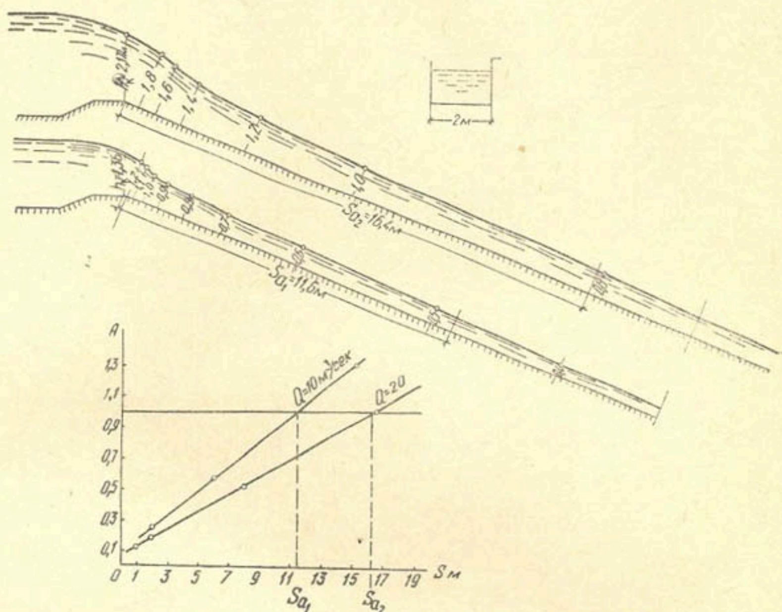
Рис. 2. Пример использования критерия A при гидравлических расчетах ( n=0,016 , i=0,4 ).
