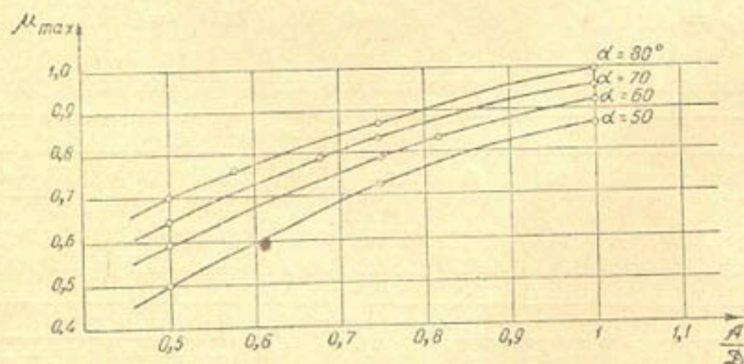
Рис. 3. График изменения максимальных коэффициентов расхода конусных затворов \mu_{\max} = f\left(\alpha^\circ; \frac{A}{D}\right) для \alpha = 50, 60, 70 и 80^\circ .
