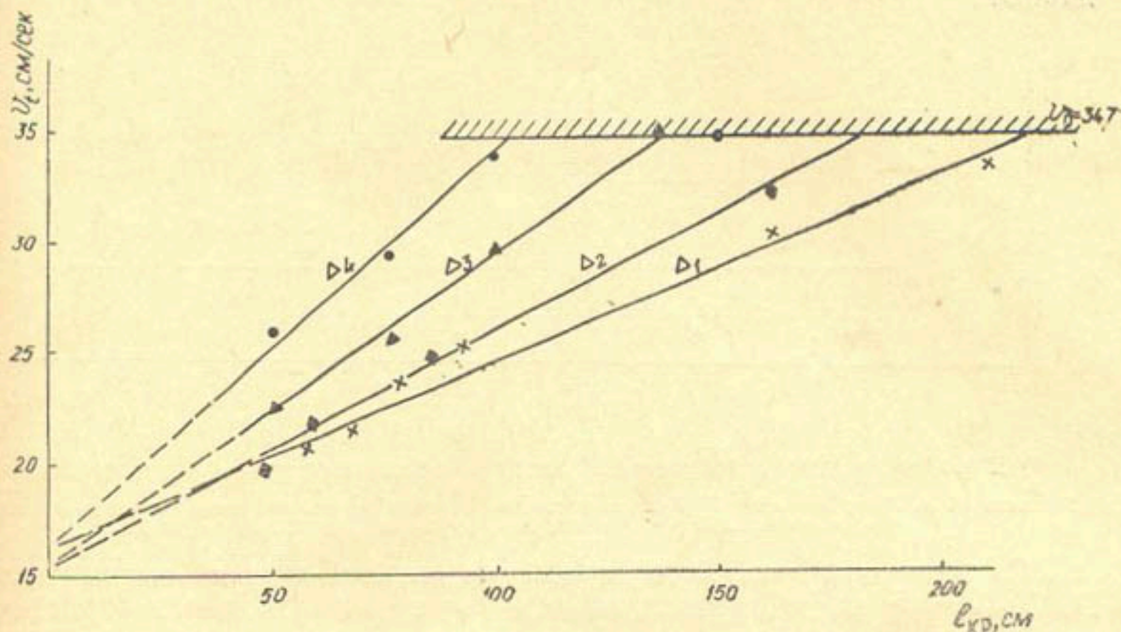
Рис. 3. График зависимости V_t = f(l_{кр}, \Delta_{кр}) . Данные опытов: q = 250 \text{ см}^3/\text{сек} , h_6 = 7,2 \text{ см} , H_{ш} = 12,5 \div 13,5 \text{ см} , a_{ш} = 2,5 \text{ см} ; размываемый материал — песок; шероховатости: \Delta_1 — облицовка из стекла, \Delta_2 — стальной лист, \Delta_3, \Delta_4 — металлические листы с наклейкой песка диаметром 1 \div 2, 3 \div 5 \text{ мм} соответственно.
