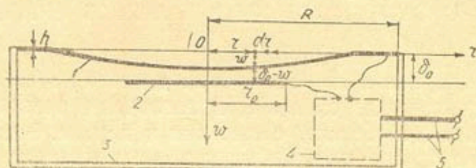
Рис. 1. Схематический разрез емкостного датчика.
