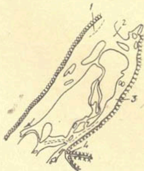
Рис. 1. План участка русла Амударьи у головы канала Ташсака (1947 г.).
