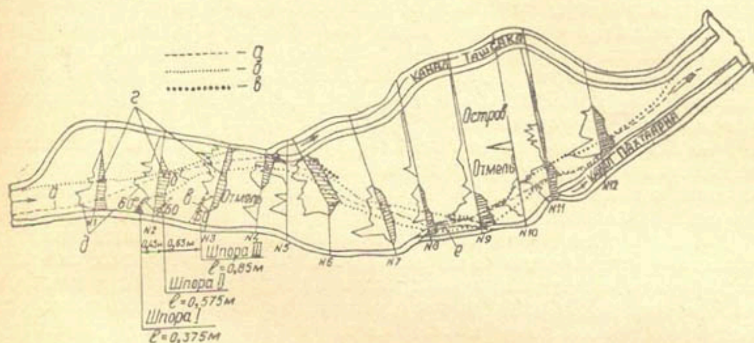
Рис. 5. План модели русла Амударьи (участок — от станции Туямуюн до водозаборного сооружения Пахтаарна) с указанием эпюры скоростей и глубины потока: II-я серия опытов, опыт I; расход на модели равен 6 л/сек, в натуре Q=6000 \text{ м}^3/\text{сек} , количество наносов Q_T = 0,4 \text{ г/л} .
