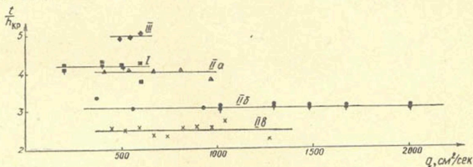
Рис. 4. Зависимость относительной глубины размыва от погонного расхода.
