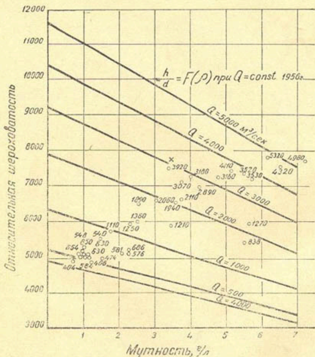
Рис. 2. График изменения относительной шероховатости в зависимости от мутности (без донных наносов) и расхода воды.
