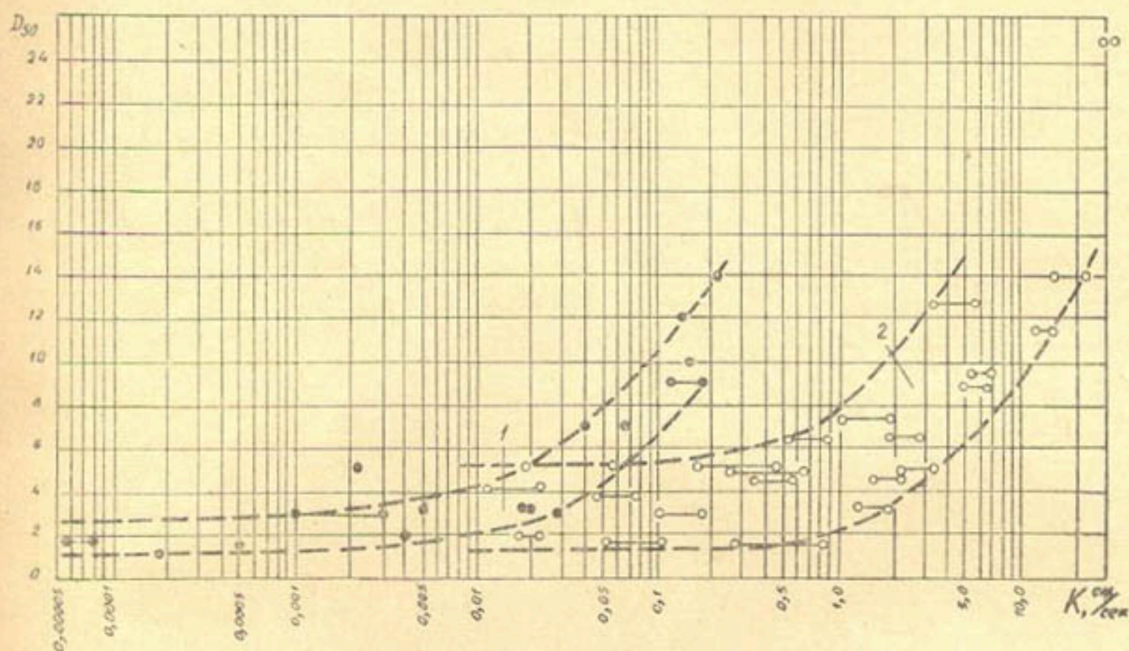
Рис. 3. Значение коэффициента фильтрации пористого бетона в зависимости от гранулометрического состава.
