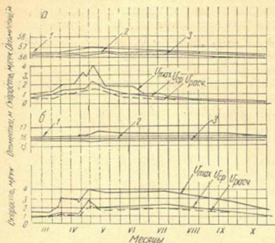
Рис. 1. Изменение средней, максимальной и расчетной скоростей потока и деформация дна с увеличением расходов воды.
