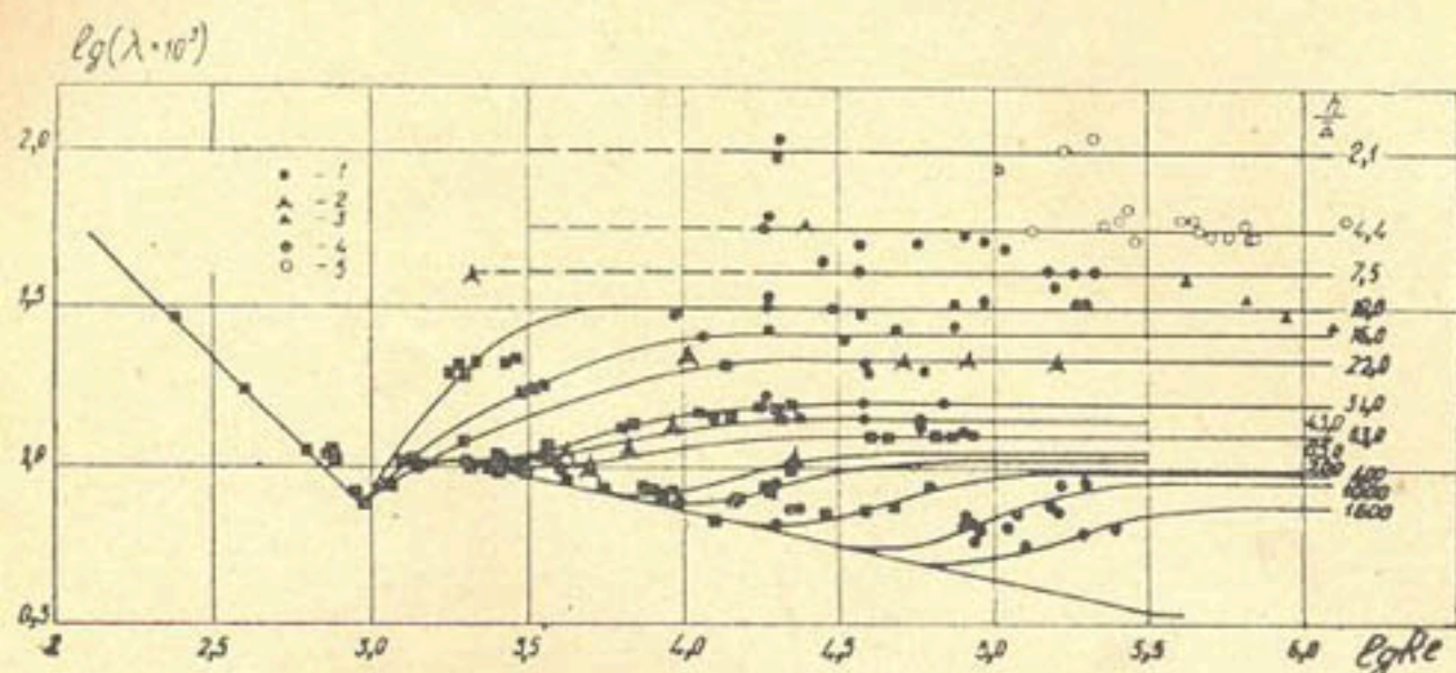
Рис. 3. График зависимости \lambda = f\left(Re, \frac{H}{\Delta}\right) .
