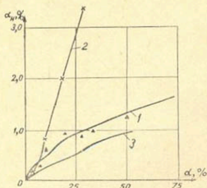
Рис. 3. График зависимости процента попадания донных наносов в водоприемник от коэффициента водозабора.
