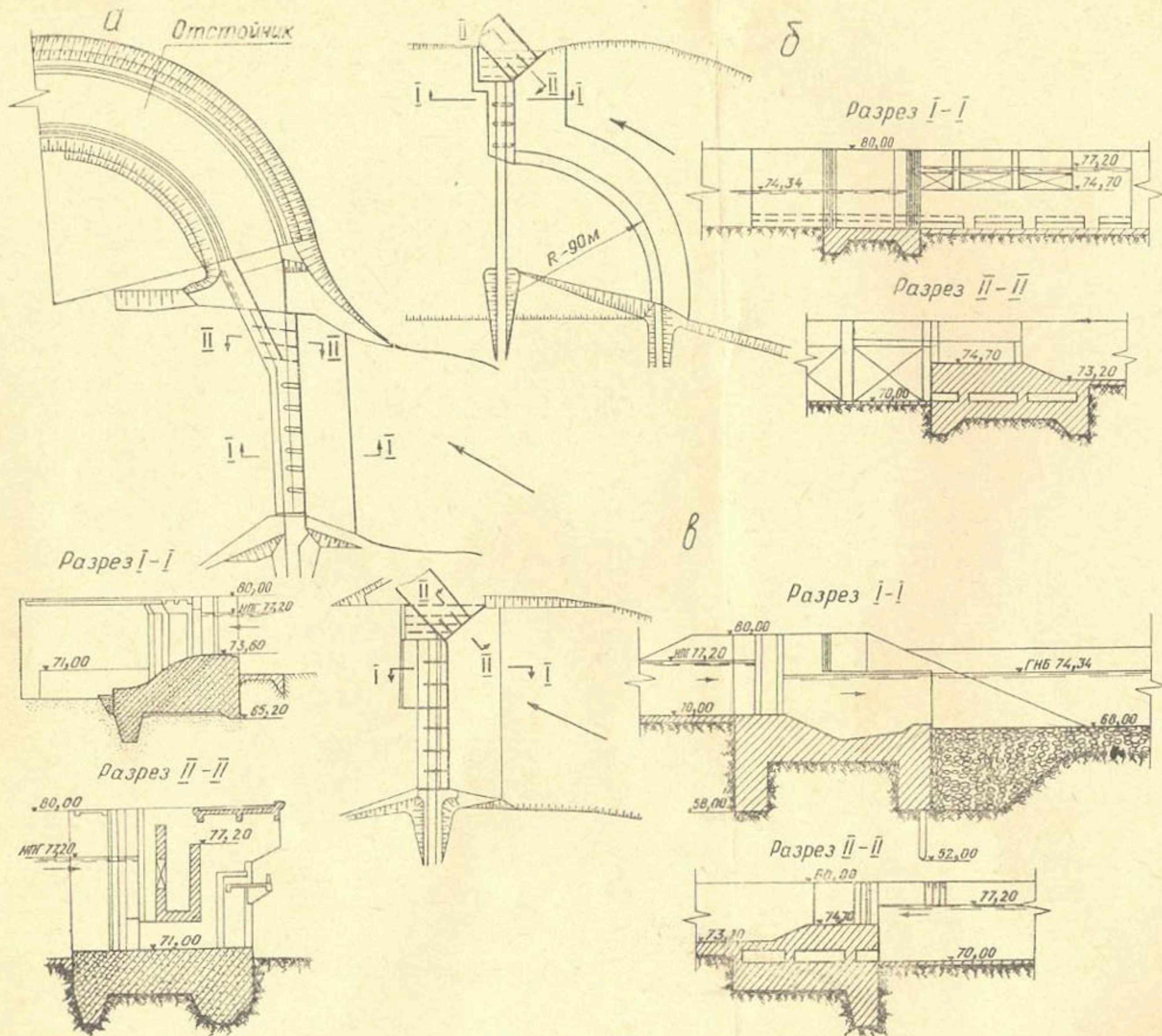
Рис. 1. План и разрезы вариантов компоновки гидроузла.
