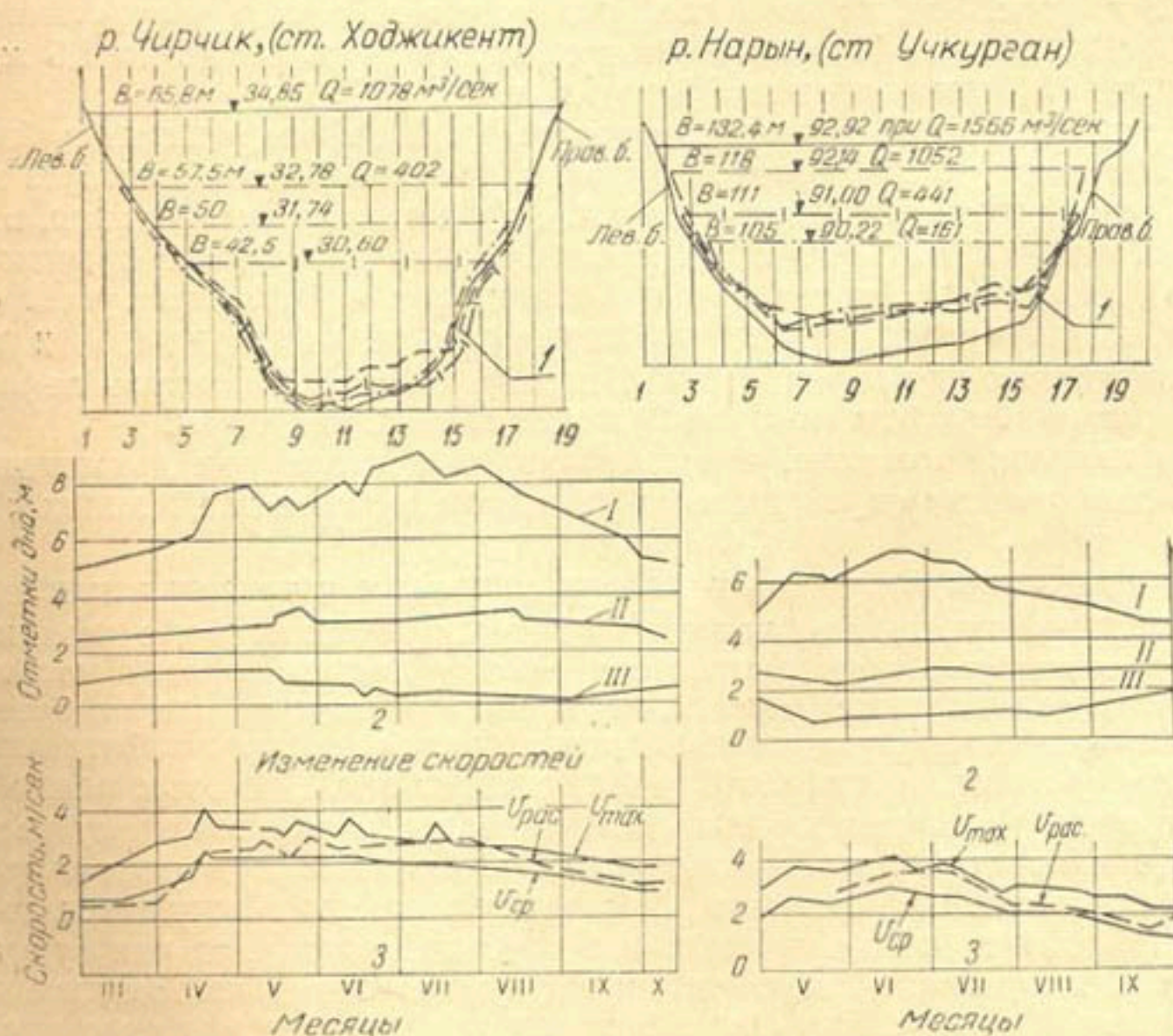
Рис. 2. К характеристике режима рек, 1942 г.
