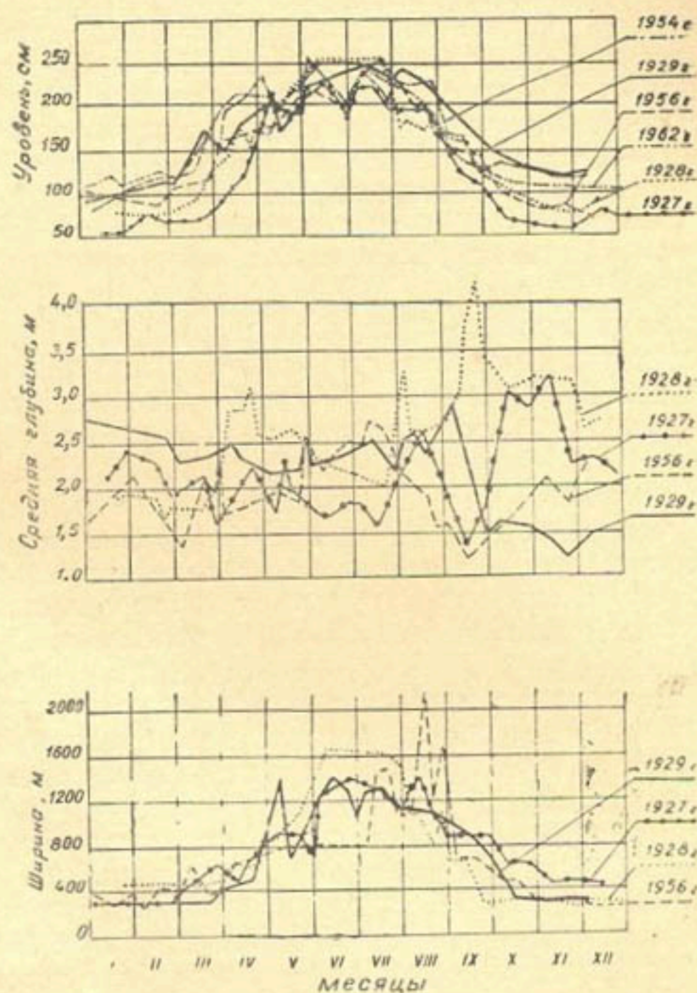
Рис. 1. Графики изменения уровня воды, глубины и ширины потока по годам по створу гидрологической станции Керки на реке Амударье.
