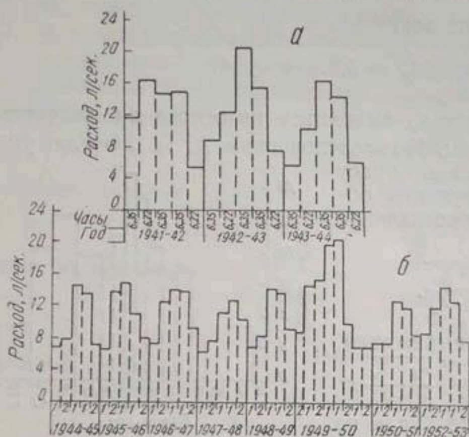
Рис. 5. Модельные гидрографы режима работы Головной ГЭС (а) и Нурекской (б): время пропуска расхода: 1—6 час. 35 мин; 2—6 час. 22 мин.
