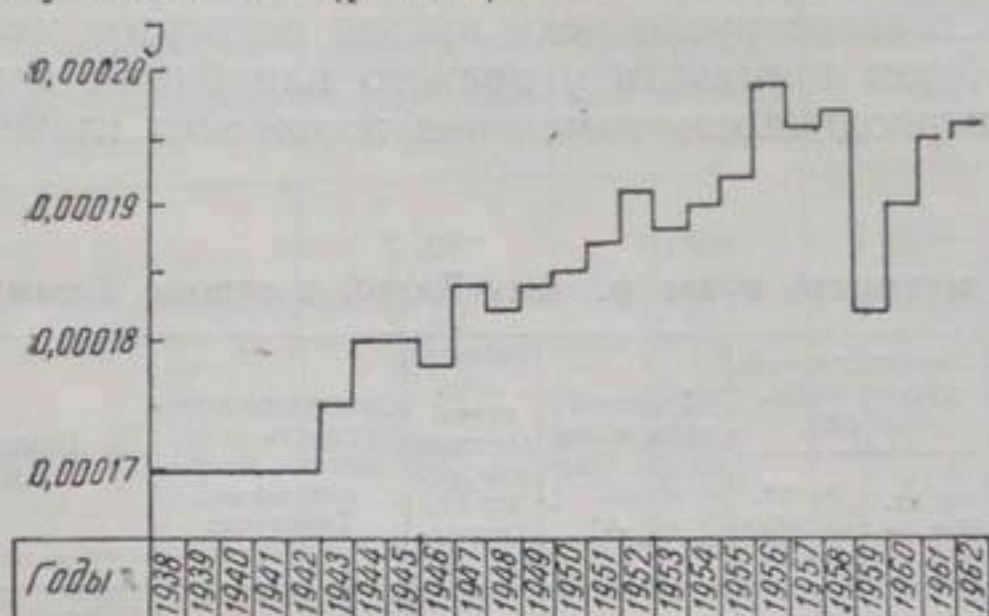
Рис. 5. График изменения среднегодовых уклонов (за 8 мес.) на участке р. Аму-Дарьи между постами Ташсака и Турткуль.
