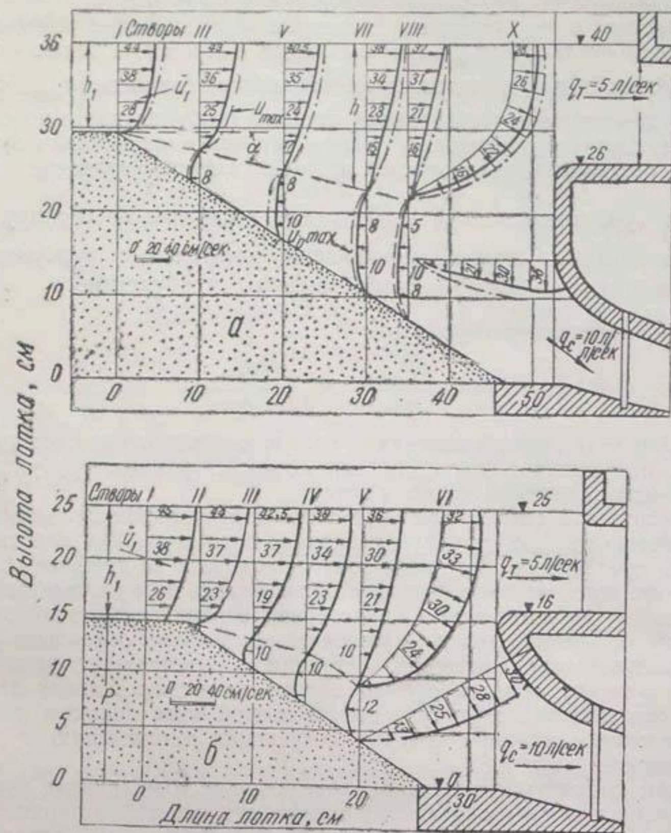
Рис. 1. Поле средних скоростей при q = 15 л/сек на II (а) и III (б) моделях.
