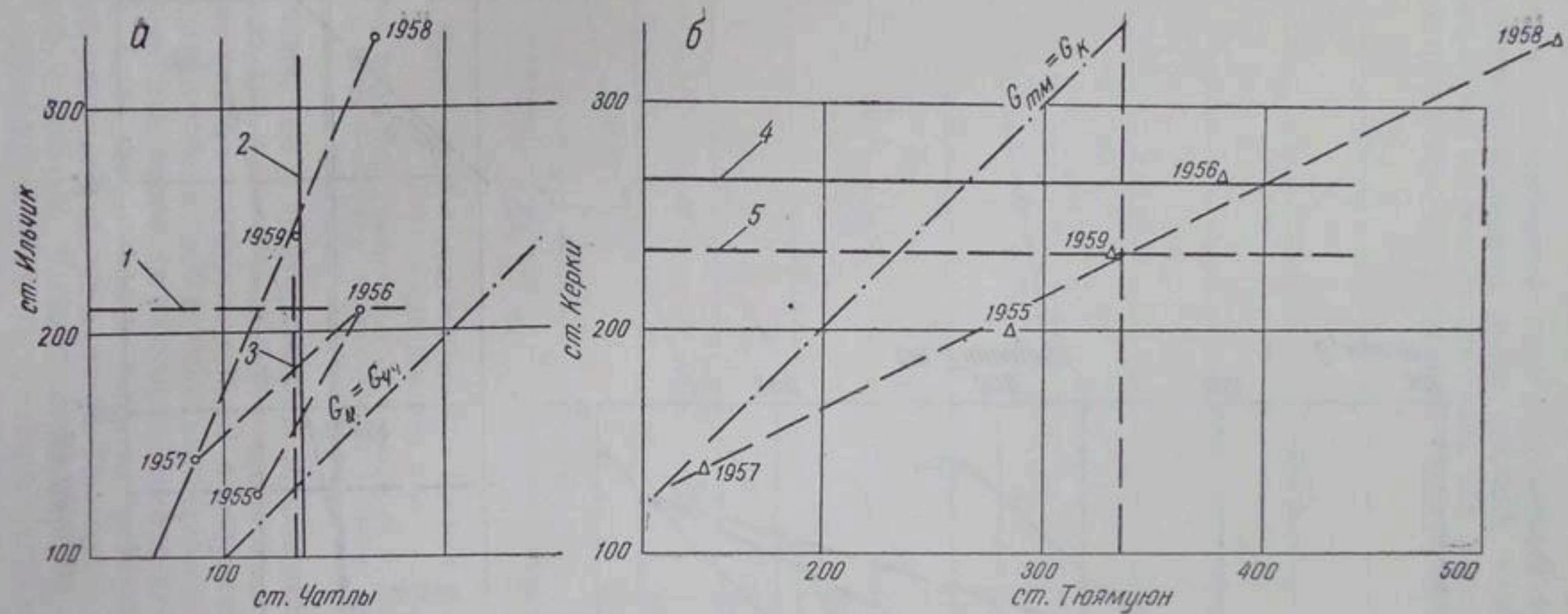
Рис. 3. Связь годового стока взвешенных наносов р. Аму-Дарьи по станциям Ильчик и Чатлы (а), Керки и Тюмуйун (б):
