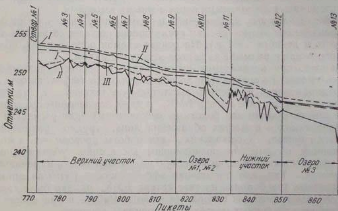
Рис. 1. Продольный профиль горизонтов воды и наинизшего размывтого дна ЦЖК в 1961 г. по 13 створам:
