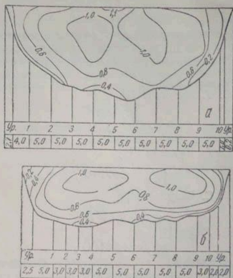
Рис. 2. Изогеты на поперечном профиле каналов (в Хорезме):
