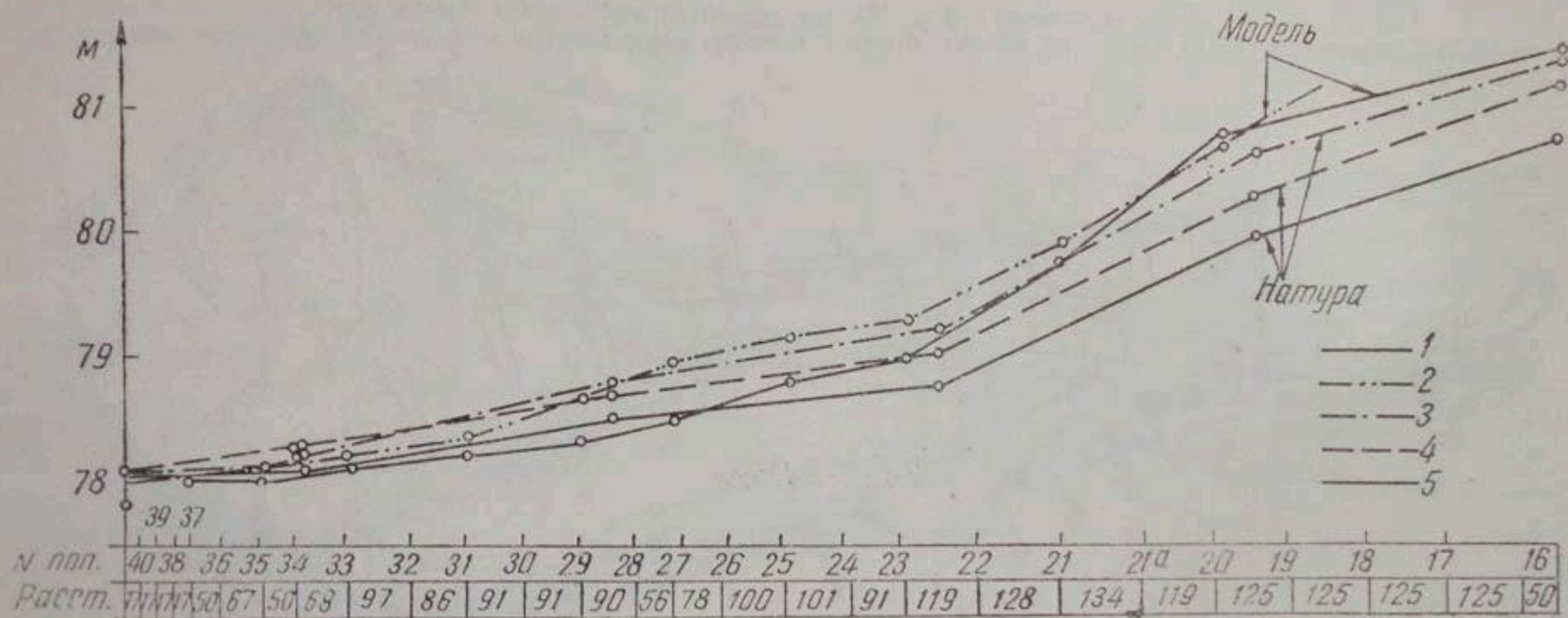
Рис. 7. Совмещенный продольный профиль мгновенных горизонтов воды по верхнему бьефу в натуре и модели: модель: 1— Q=450 \text{ м}^3/\text{сек} ; 2— Q=520 \text{ м}^3/\text{сек} ; натура: 3— Q=530 \text{ м}^3/\text{сек} ; 4— Q=465 \text{ м}^3/\text{сек} ; 5— Q=330 \text{ м}^3/\text{сек} .
