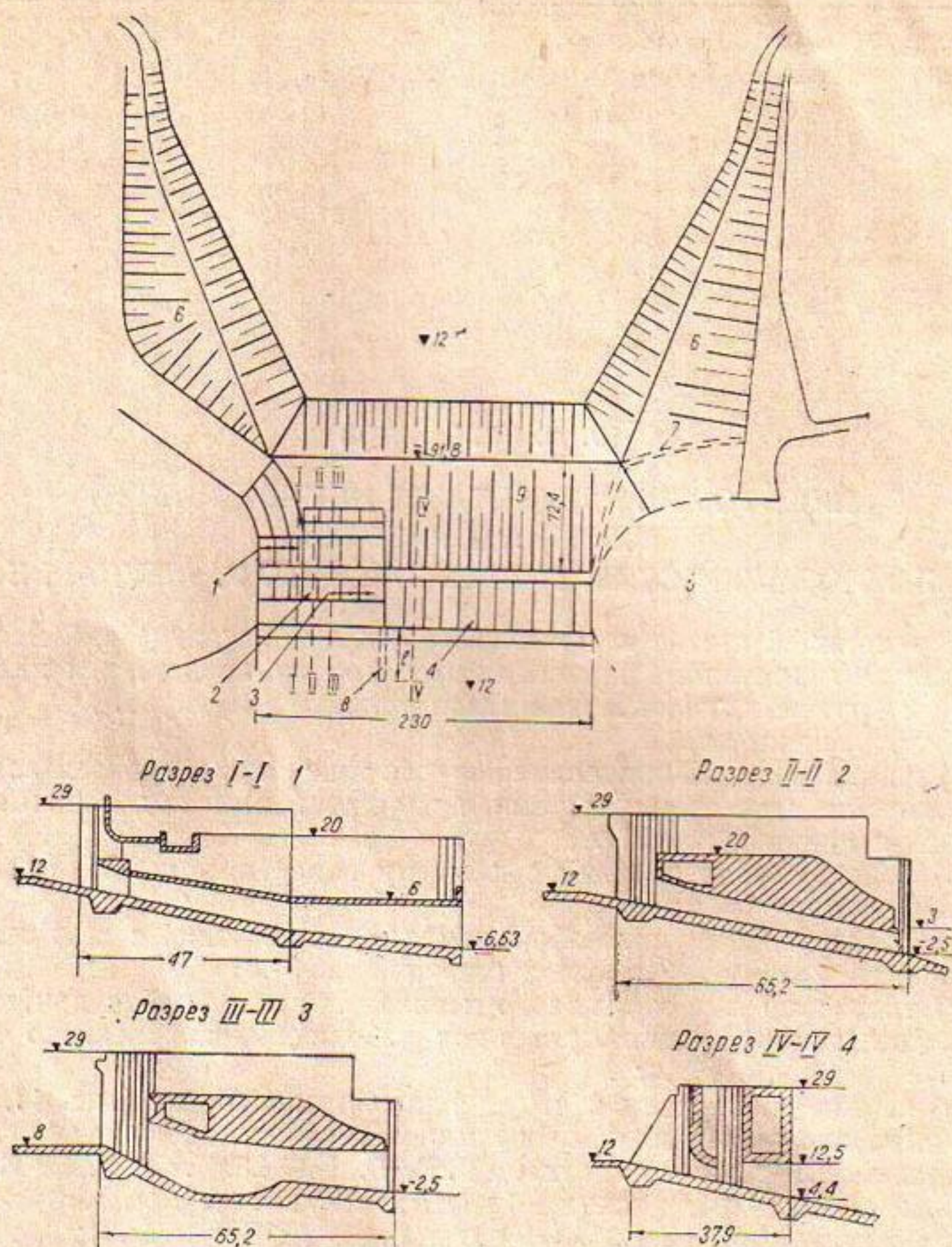
Рис. 1. Схема Тюямунского гидроузла, план и разрезы сооружений: 1—левобережный водозабор; 2—рыбоход и правобережный водозабор; 3—здание ГЭС; 4—водобросная плотина; 5—земляная плотина; 6—правый и левый струенаправляющие пирсы; 7—рекомендуемая сопрягающая стенка; 8—рекомендуемая разделяющая стенка ( l = 1,5 \cdot h бычка); 9—водобой.
