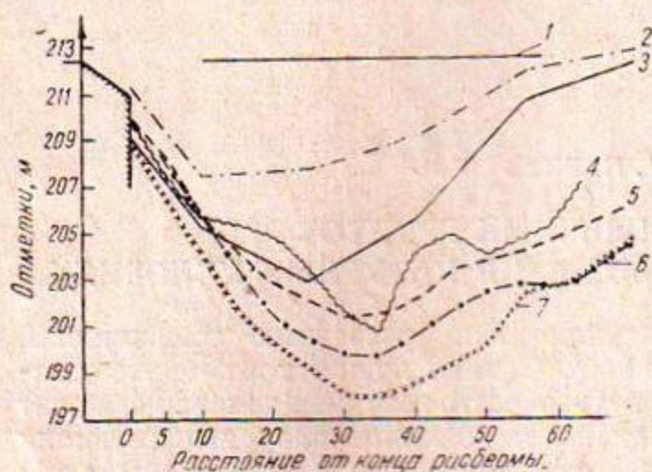
Рис. 1. Профиль размыва по оси пролета № 5: 1 — поверхность дна до размыва; 2 — q = 7,9 \text{ м}^3/\text{сек} (через 4 часа); 3 — q = 12,8 \text{ м}^3/\text{сек} (через 4 часа); 4 — дно в натуре (1946 г.); 5 — q = 19,3 \text{ м}^3/\text{сек} (через 18 \frac{1}{2} час.); 6 — q = 22,5 \text{ м}^3/\text{сек} (через 4 часа); 7 — q = 22,5 \text{ м}^3/\text{сек} (через 17 час.).
