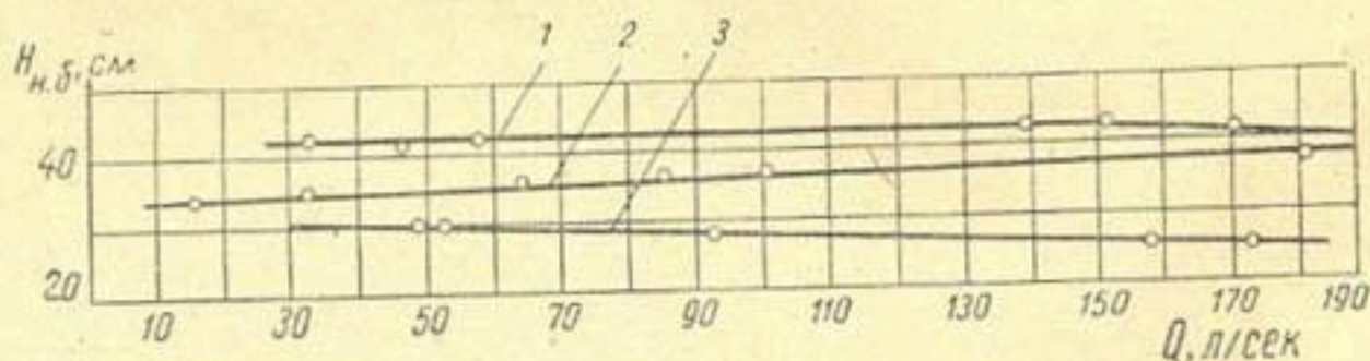
Рис. 5. График поддержания постоянного горизонта в нижнем бьефе для автомата с поплавком в русле (тип „Нейрпик“):
