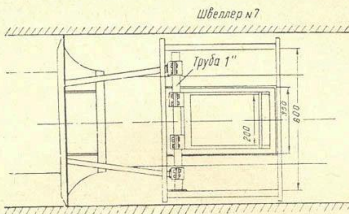
Рис. 2. Схема затвора-автомата нижнего бьефа с поплавком в русле (тип „Нейрпик“). Поплавок, полотнище затвора, корыто изготовить из листового железа \delta=1 мм.
