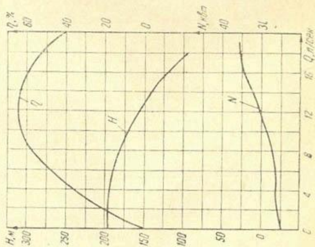
рис. 22. Рабочая характеристика насоса 10ЛПВМ-9×7.
