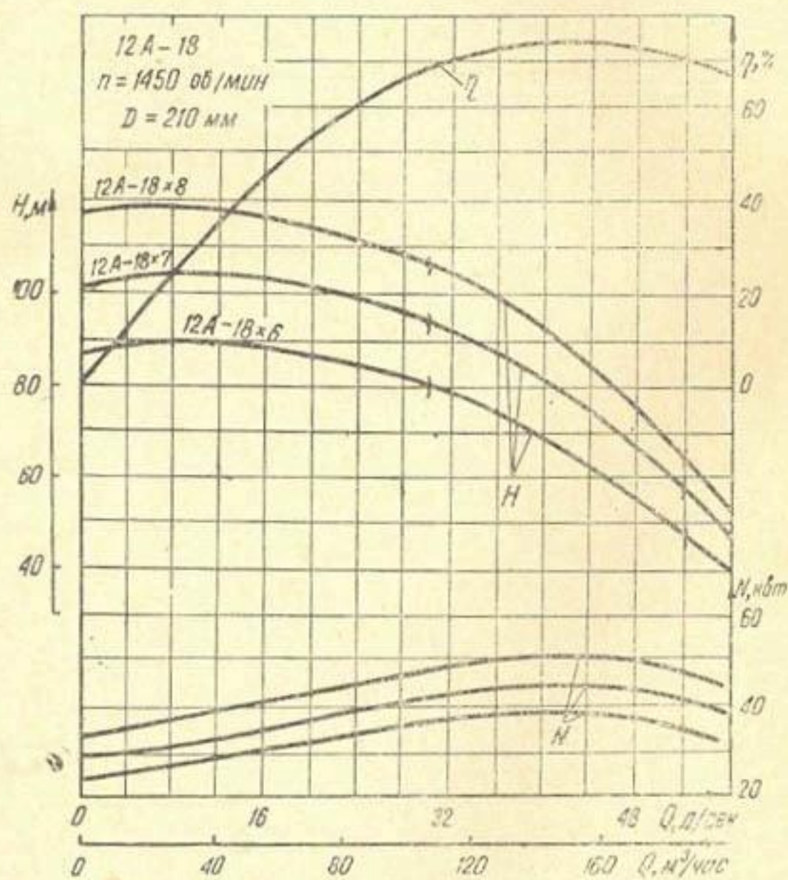
Рис. 31. Рабочая характеристика насосов 12А-18×6, 12А-18×7, 12А-18×8.
