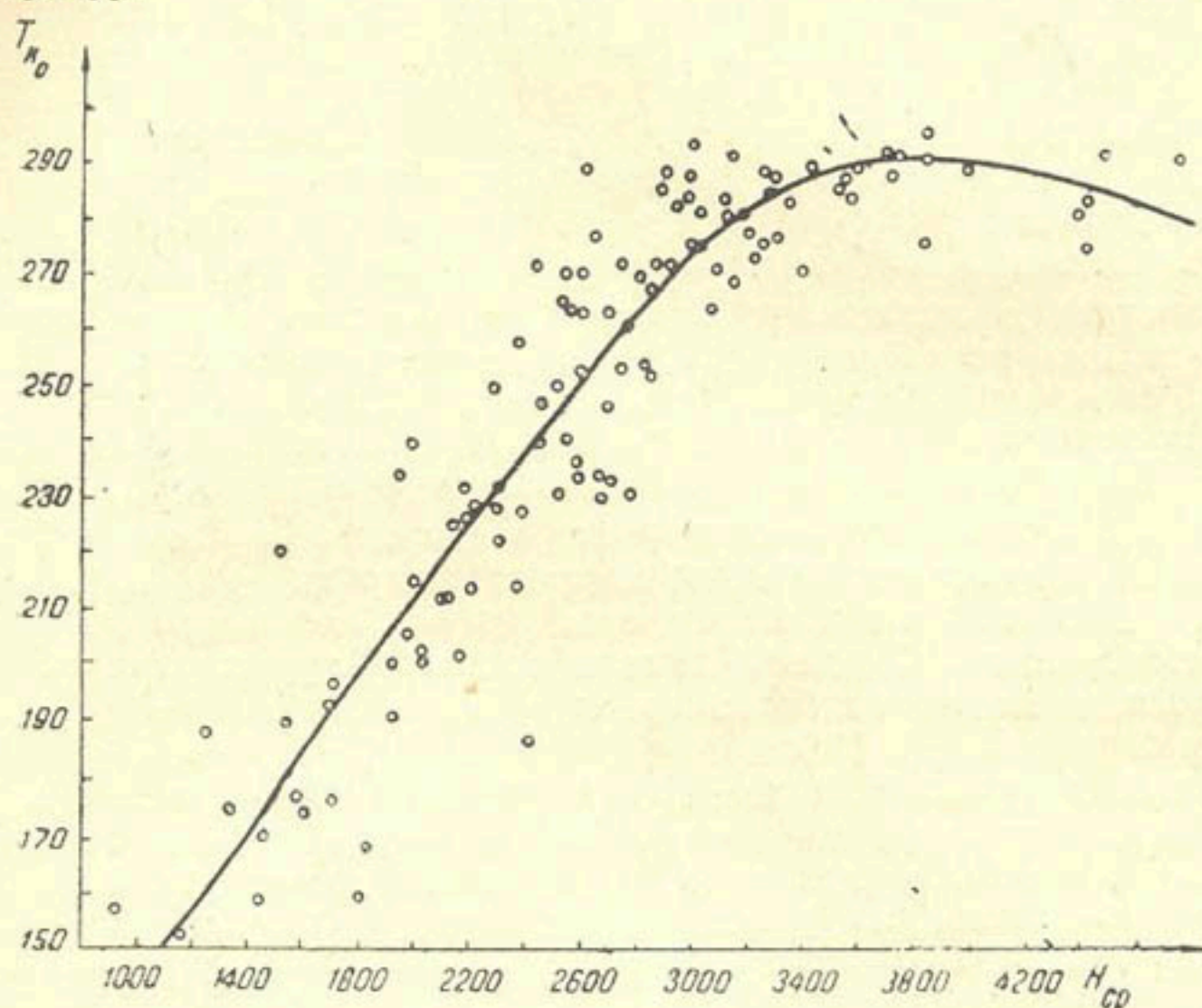
Рис. 2. Зависимость дат конца паводков от H_{cp} .
