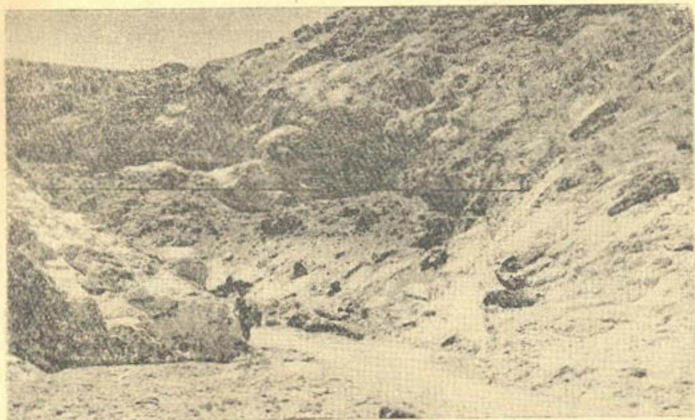
Рис. 2. Метки максимального уровня селевого паводка в ущелье Тойчи 30 апреля 1962 г.
