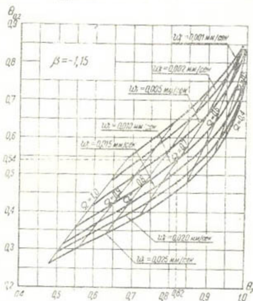
Рис. 3. График для определения параметров w_1 и \Omega по заданному составу наносов при \beta = -1,15 .
