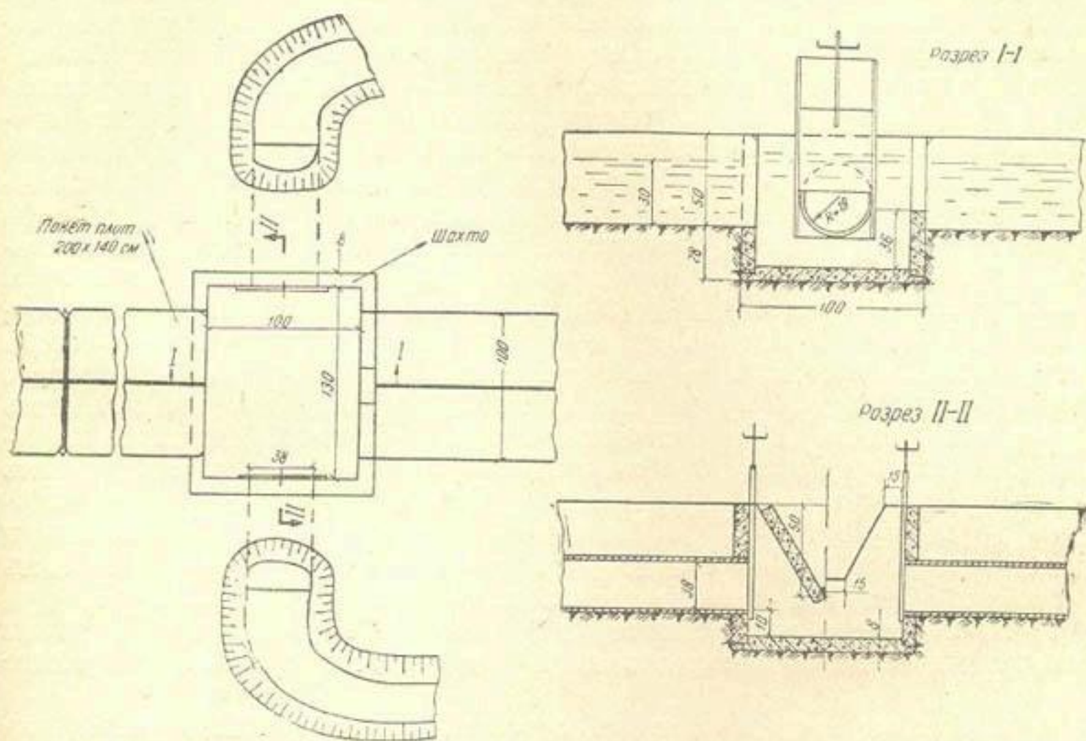
Рис. 5. Схема водовыпуска с Q = 200 л/сек из облицованного канала треугольного сечения; расход материалов: бетон — 0,3 м 3 ; арматура — 2,7 кг; металлоконструкции — 16 кг.
