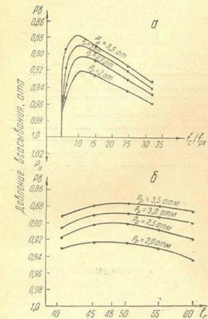
Рис. 3. График зависимости давления всасывания при различных значениях
