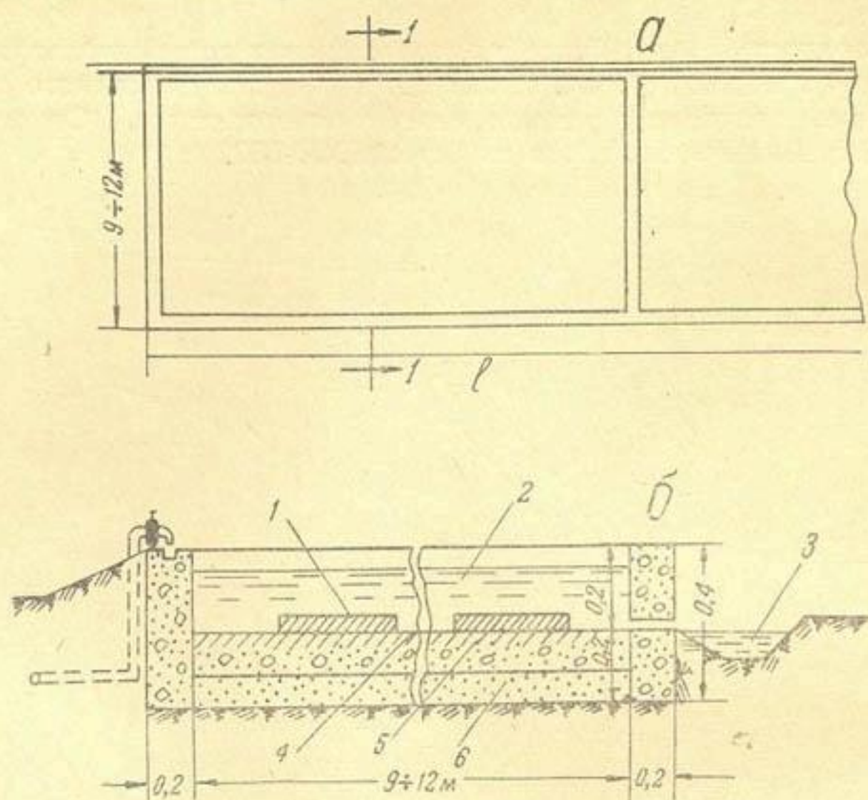
Рис. 4. План (а) и разрез (б) стенда-бассейна:
