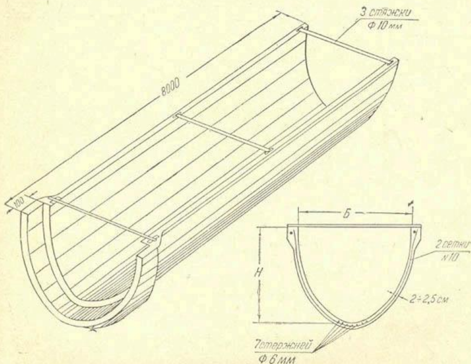
Рис. 1. Армоцементный лоток.
