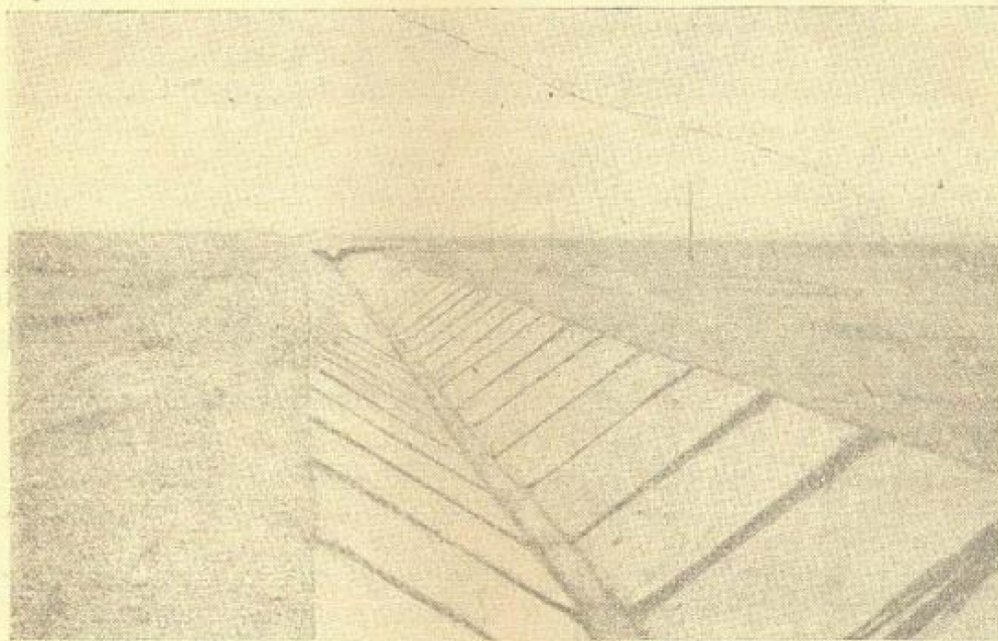
Рис. 1. Сборная облицовка трапецидального канала.
