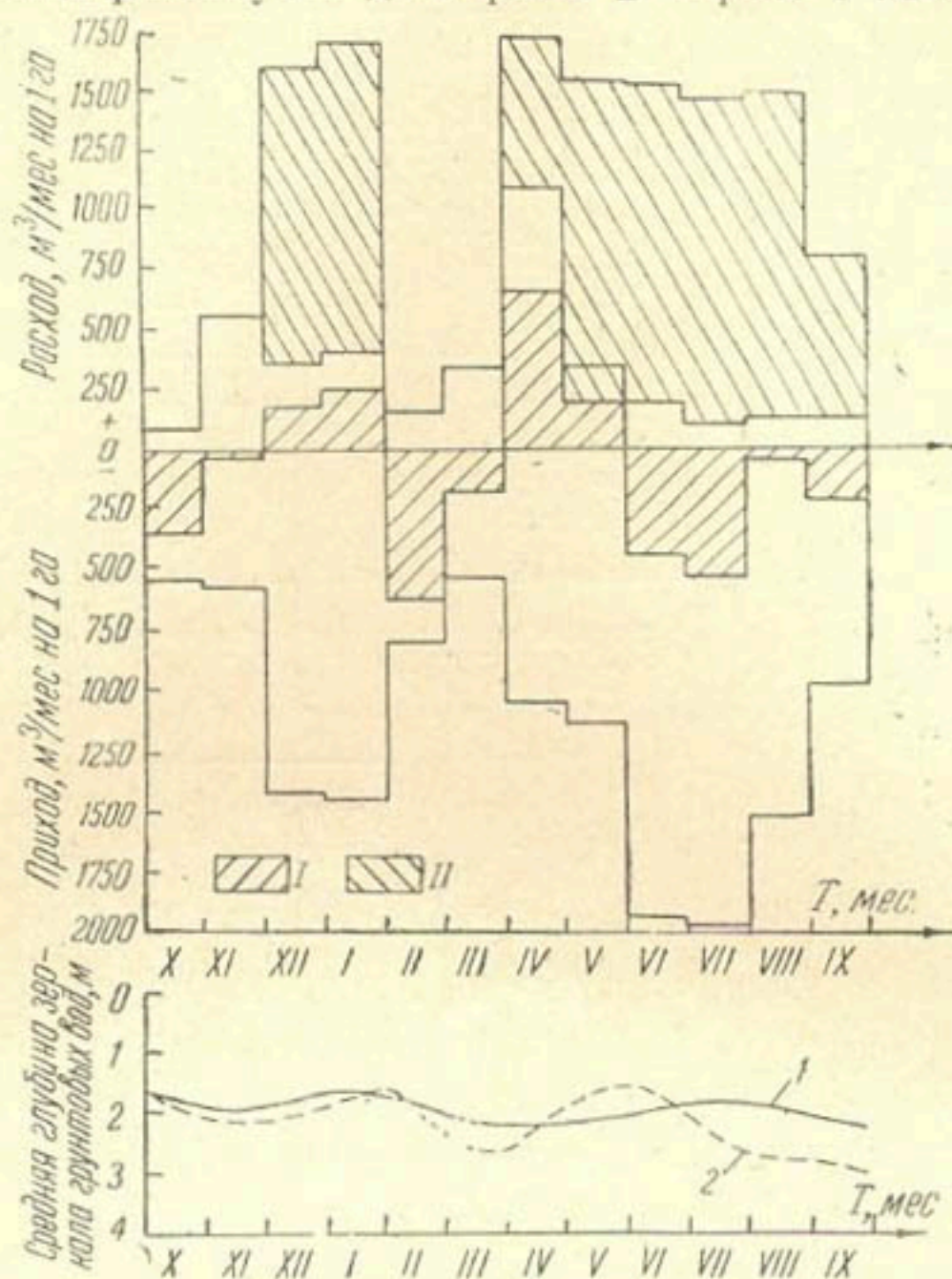
Рис. 2. График прогноза водного баланса и уровня грунтовых вод Шурузякского участка при полном переключении участка на орошение откачиваемых подземных вод ( \omega_{6p} = 2000 \text{ га} при КЗИ—0,9):
