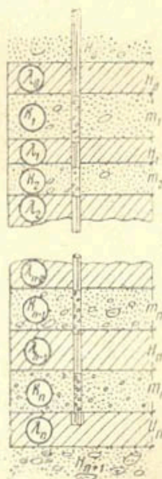
Рис. 1. Схема заложения скважины в n пластах.
