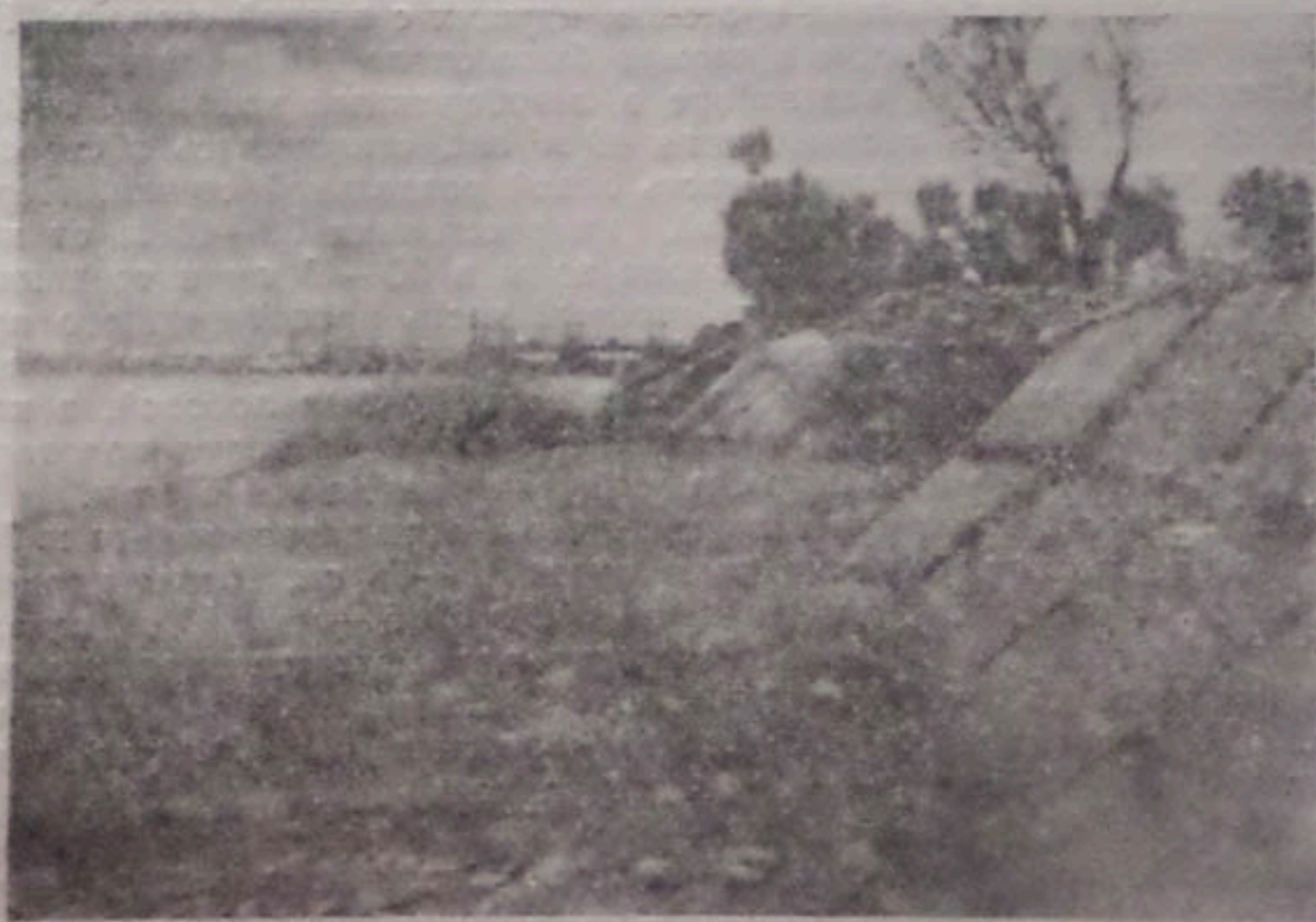
Рис. 23. Разрушение правой струенаправляющей дамбы выше отверстий кольматажного озера.
