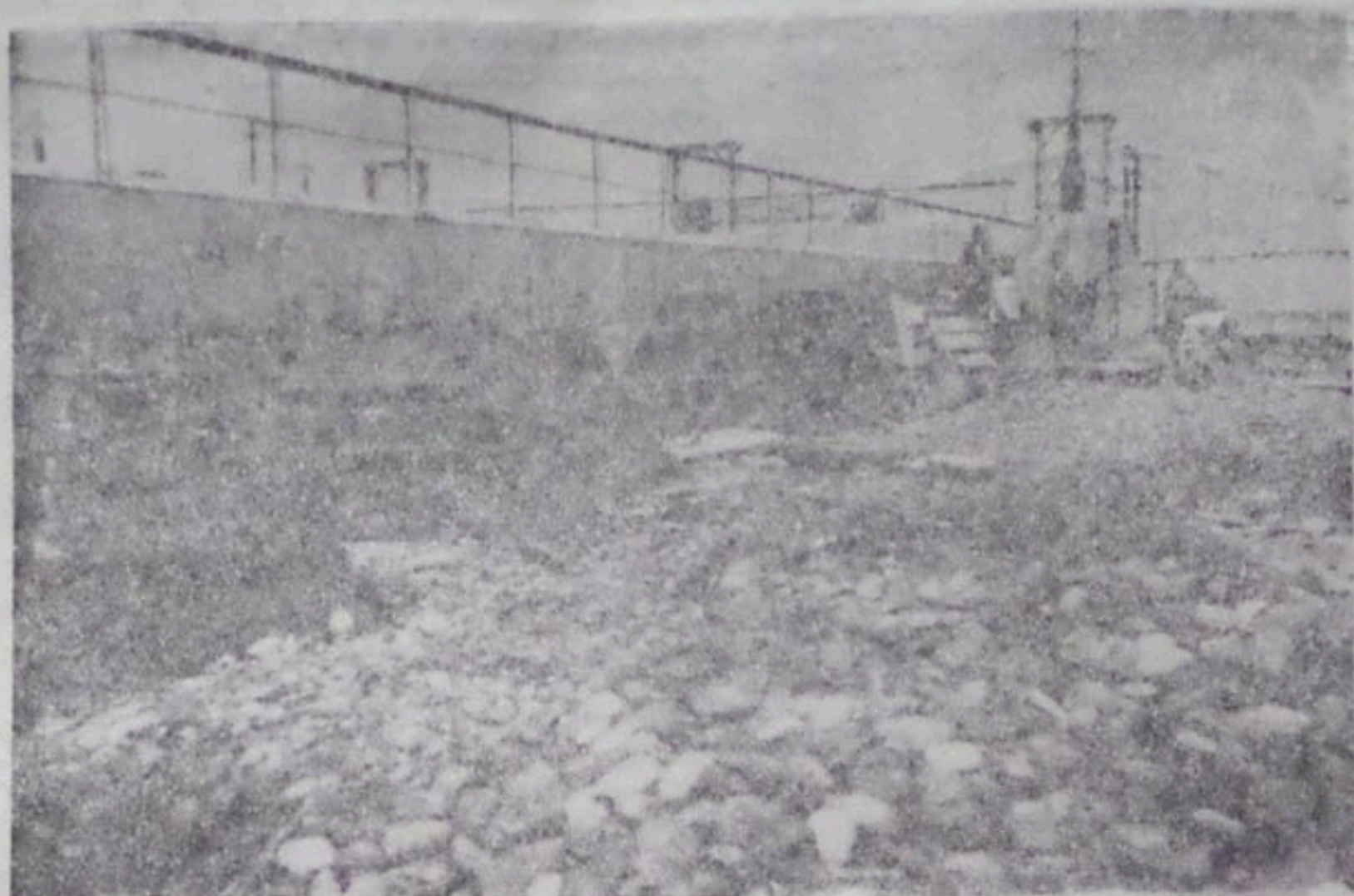
Рис. 19. Бетонные тетраэдры, уложенные в голову отдельных стенок перед паводком 1951 г.
