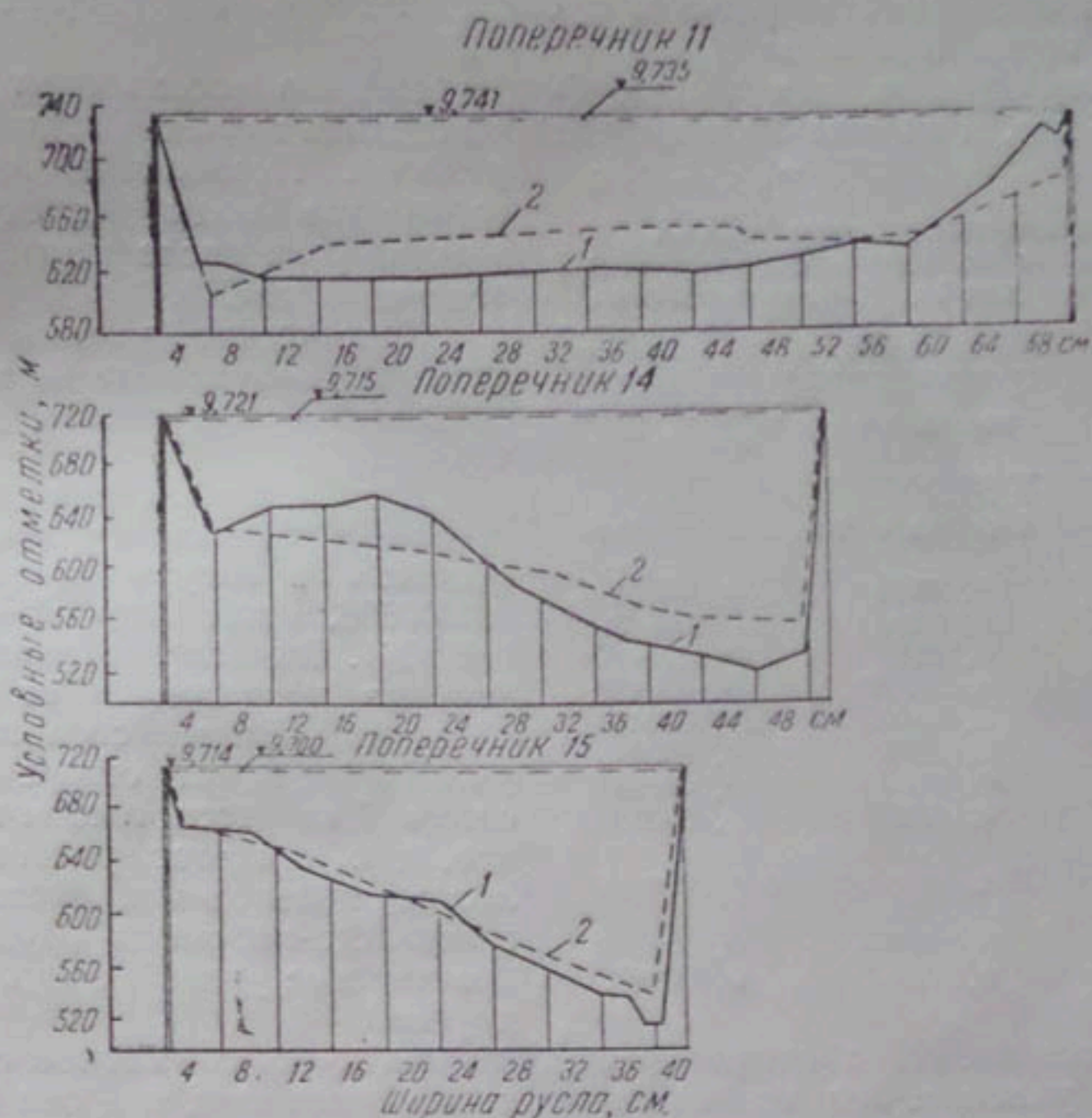
Рис. 4. Совмещенные поперечные профили модели и природы II серии опытов:
