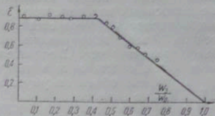
Рис. 3. Изменение степени освещения \varepsilon лабораторного бьефа 2 в зависимости от относительной величины заиления \frac{W_3}{W_0} .
