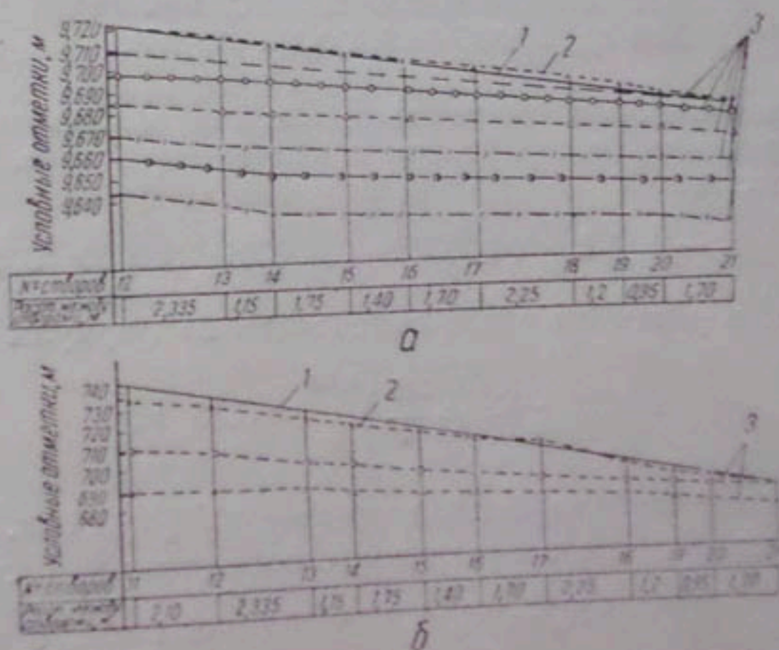
Рис. 5. Продольный профиль горизонта воды I (а) и II (б) серии опытов:
