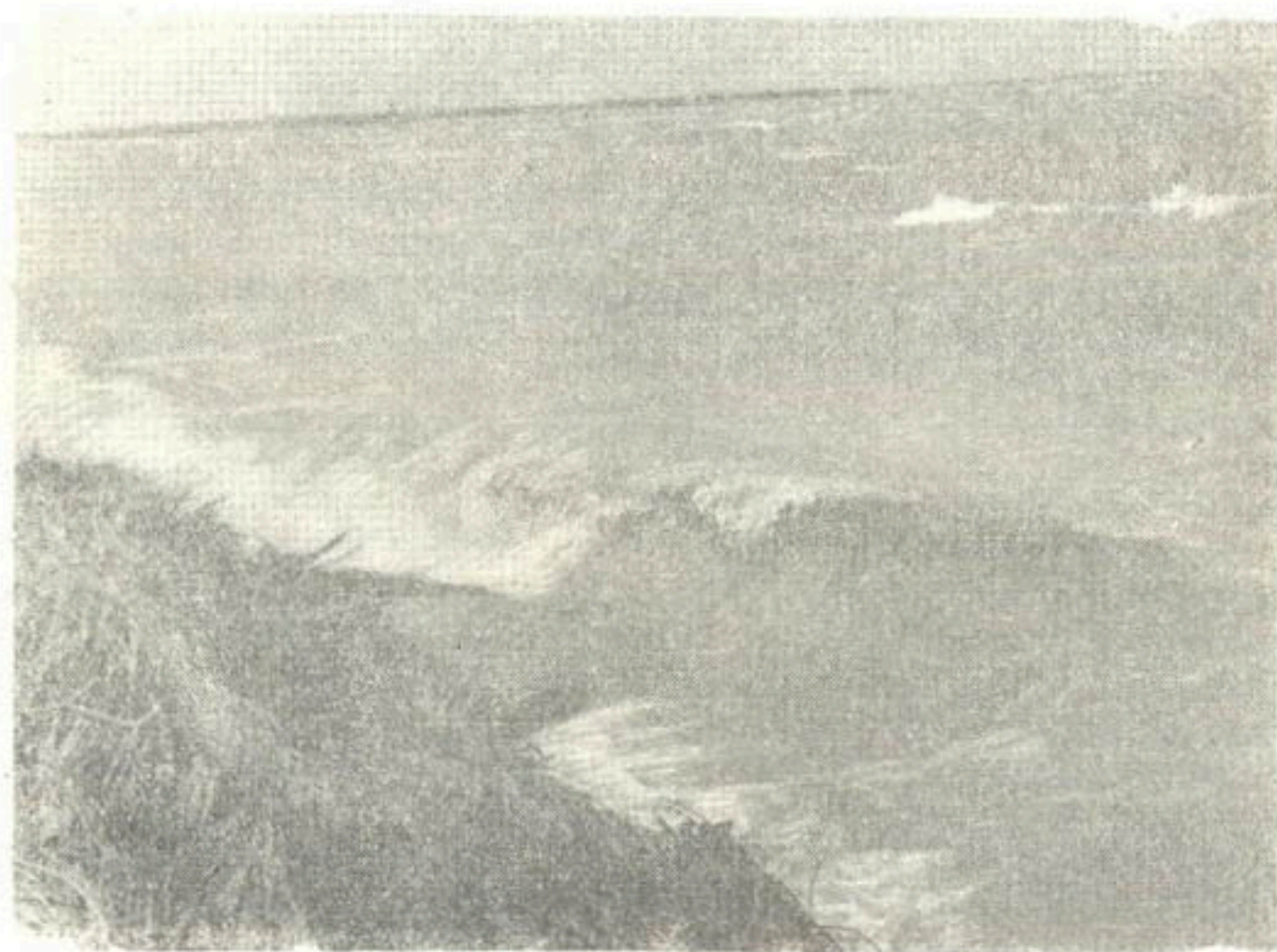
Рис. 7. Тедженское водохранилище; разрушение фашинного крепления ветровой волной.
