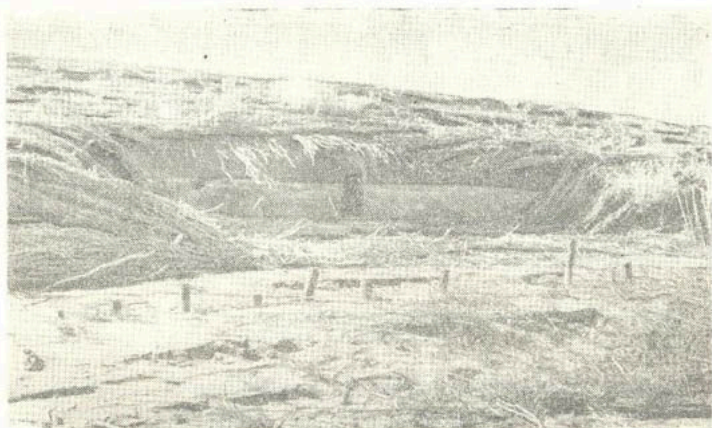
Рис. 8. Тедженское водохранилище; разрушенное фашинное крепление левой дамбы.
