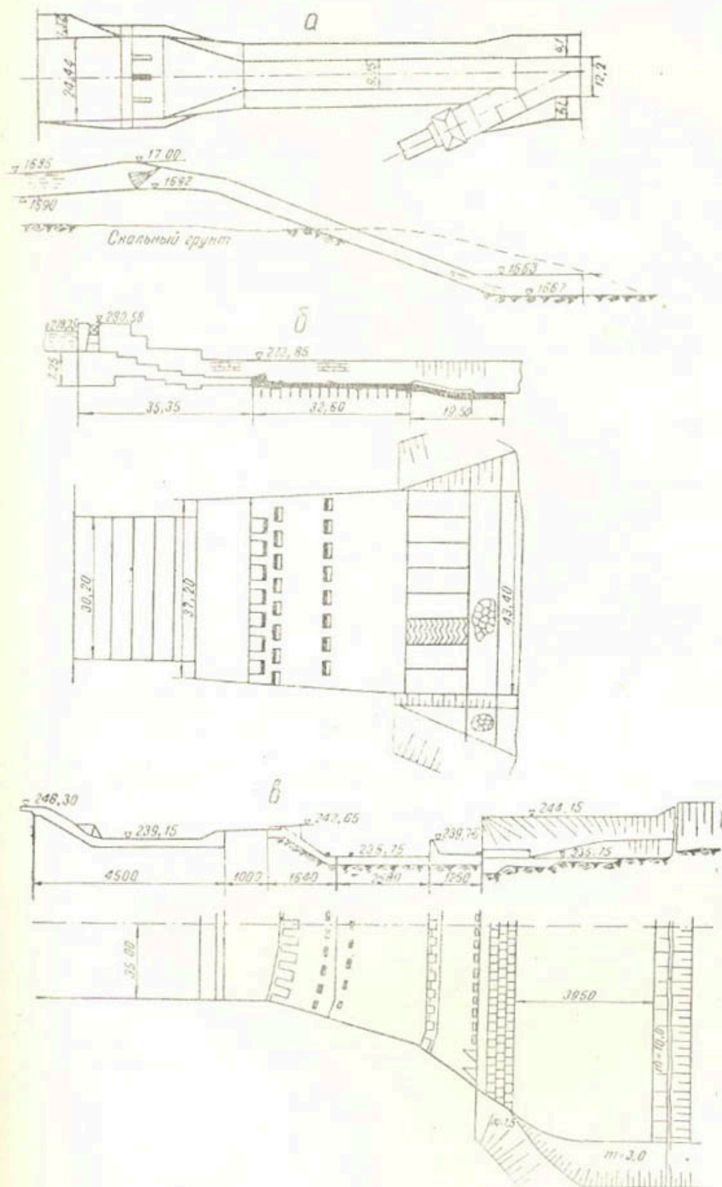
Рис. 10. Схема водовыпуска — водосброса при плотине Эхо в США по проекту 1931 г. на расход Q_{\max} = 405 \text{ м}^3/\text{сек} ( q_{\max} = 45 ), общем перепаде z \approx 31 \text{ м} и уклоне быстрого тока i = 0,25 . Грунт в нижнем бьефе скальный (а). Схема Гиндукушской плотины после реконструкции и ремонта 1953 г. (б). Схема расположения гасителей энергии для реконструкции нижнего бьефа водовыпуска из Тедженского водохранилища (в).
