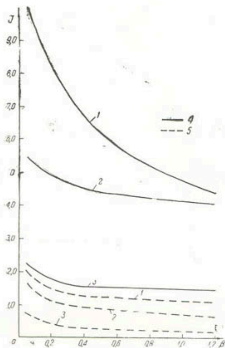
Рис. 17. Значение I_{\max} для водовыпусков с дренажем в виде перехватывающей дрены и тюфяка в концевой части. Условные обозначения те же, что и на рис. 16.
