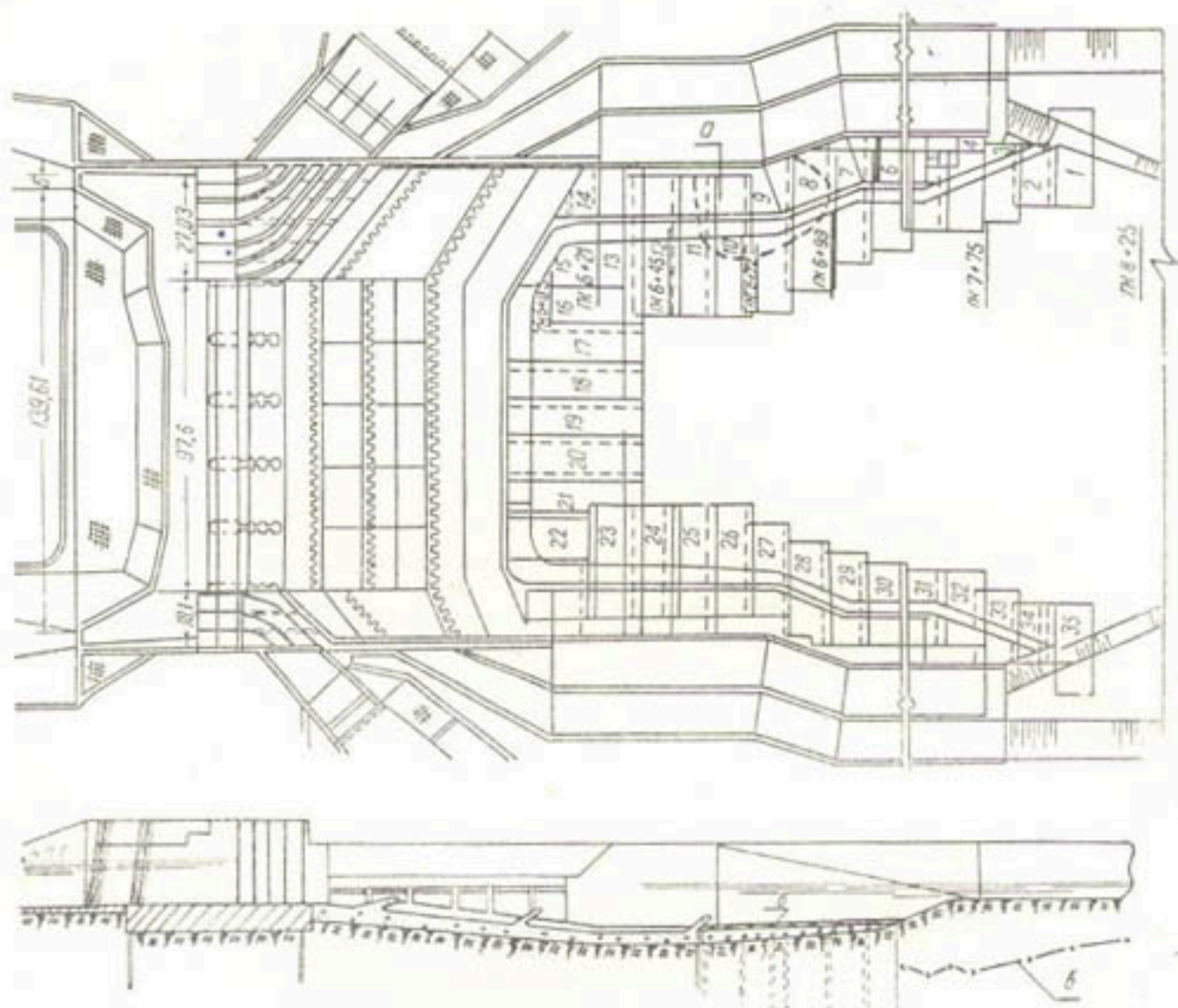
Рис. 1. План и продольный разрез Кызыл-Ординского гидроузла: 1—35—каменно-хворостинные тюфины; а—зона разрушения рибермы в 1957 г.; б—деревянный Уральский пол; в—линия размыва дна.
