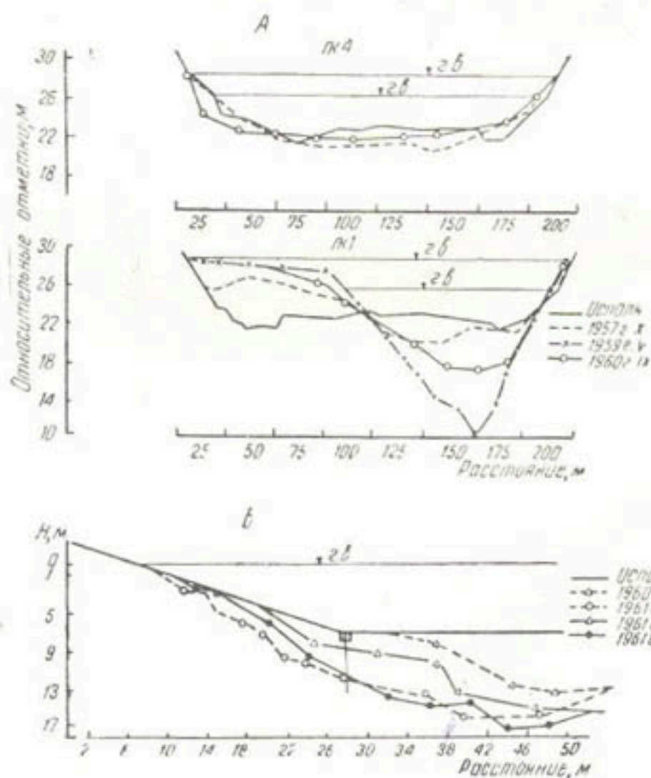
Рис. 5. Поперечные профили подводящего русла ПК 4 (100 м от плотины), ПК 1 (400 м от плотины) (А); размывы у оголовка верхней струенаправляющей дамбы (Б).
