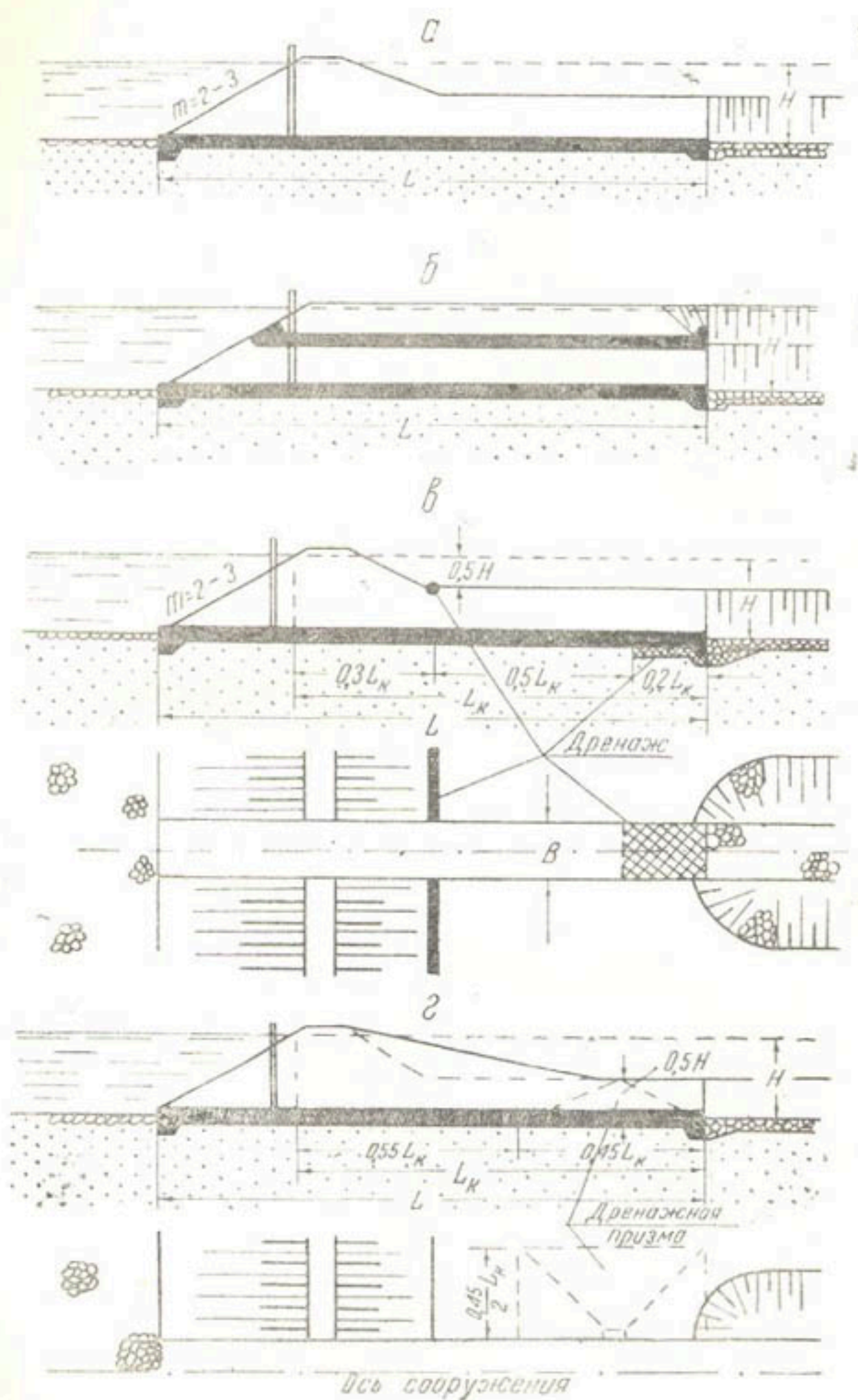
Рис. 8. Схема конструкций исследованных водопусков.
