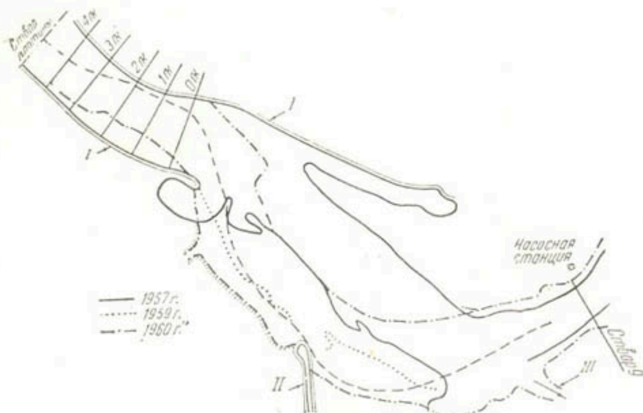
Рис. 4. Деформации подводящего русла: I — низкие струенаправляющие дамбы; II — верхняя струенаправляющая дамба; III — водозабор в обводнительный канал Жигаловья.
