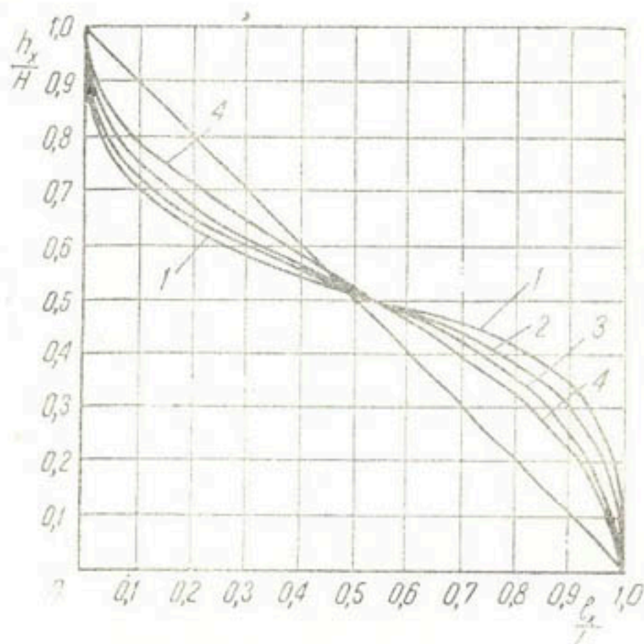
Рис. 3. Зависимость \frac{h_x}{H} = f\left(\frac{x}{L}\right) для перепадов-быстротоков без дренажных устройств: 1— \beta_2=0,20 ; 2— \beta_2=0,40 ; 3— \beta_2=0,60 ; 4—плоское решение.
