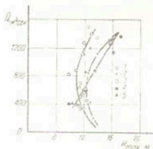
Рис. 10. Изменение глубин наибольшего размыва в нижнем бьефе плотины в зависимости от расхода воды:
