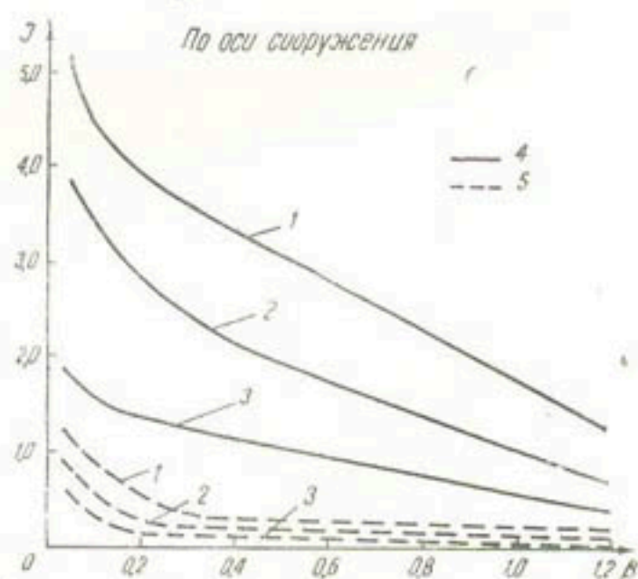
Рис. 16. Значения I_{\max} для водовыпусков с дренажем в виде перехватывающей дренажной трубы в концевой части:
