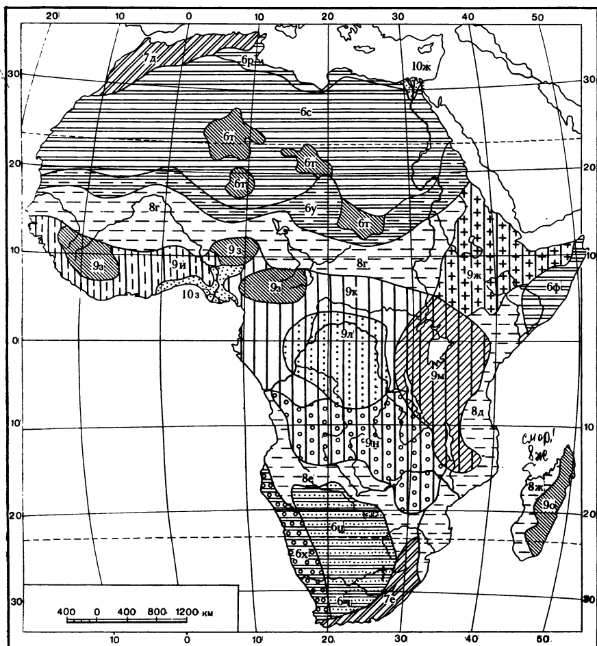
Рис. 39. Схема структуры почвенного покрова Африки. Пояснения см. в тексте и в табл. 7
