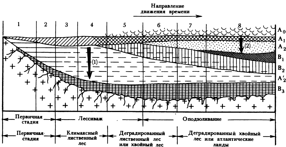
Рис. 12. Эволюция и деградация лесных почв на силикатной водопроницаемой породе (по Ф. Дюшофур, 1970):
