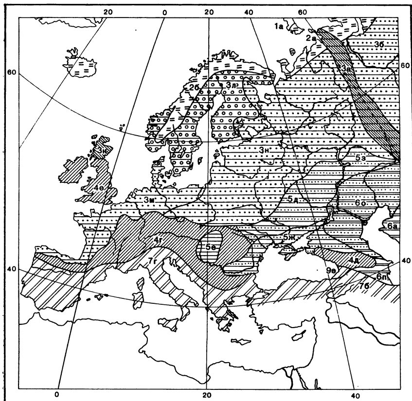
Рис. 30. Схема структуры почвенного покрова Европы (пояснения см. в тексте и в табл. 6; для азиатских регионов 3б, 6а и 7б в табл. 5)
