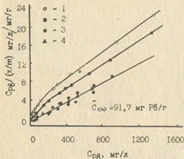
Рис.20. Изотерма адсорбции свинца Са-монтмори́ллонитом в координатах уравнения Лэнгмюра (3.8) при соотношениях твердой и жидкой фаз: 1-1:50, 2-1:100, 3-1:500, 4-1:1000 /II2/.
