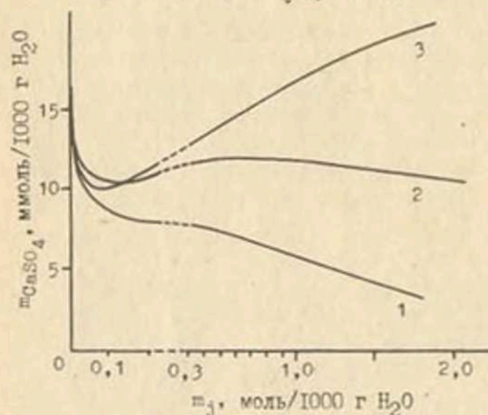
Рис.10. Растворимость гипса в водных растворах \text{CaCl}_2 (1), \text{Na}_2\text{SO}_4 (2) и \text{MgSO}_4 (3) /81/.
