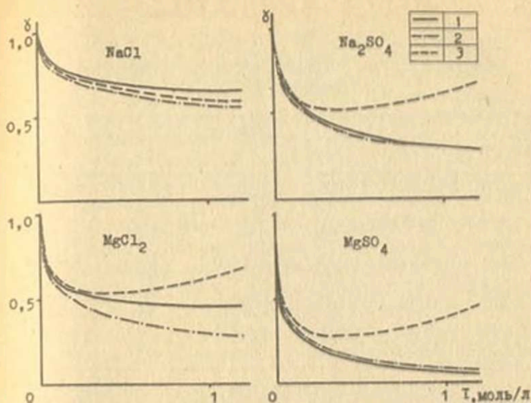
Рис. 3. Зависимость средних ионных коэффициентов активности солей от ионной силы раствора: 1 — экспериментальные данные; 2 — расчет по уравнению Гунтельберга; 3 — расчет по уравнению Дейвиса (2.8).
