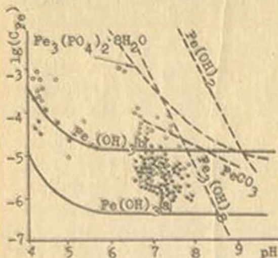
Рис. I7. Диаграмма растворимости присутствующих в почвах соединений железа ((а) — Fe(OH)_3 при pK = 37,5 ; (б) — Fe(OH)_3 при pK = 35,96 ) и концентрации Fe (III) (*) и Fe (II) в некоторых дренажных водах
