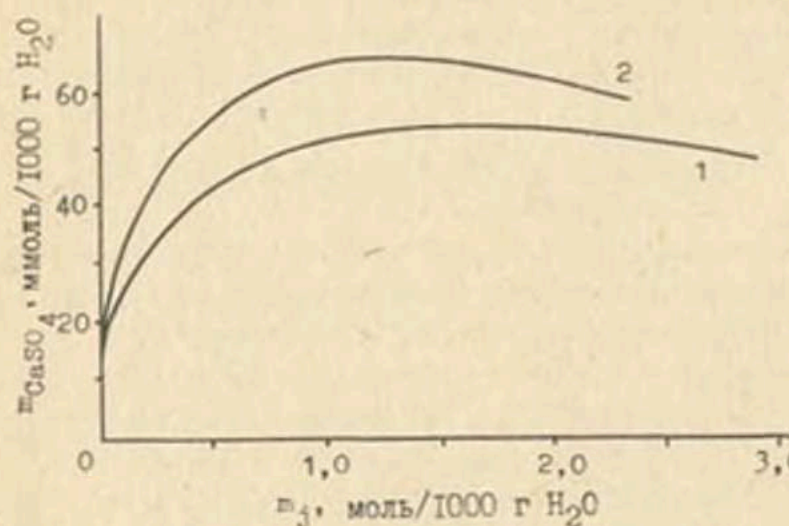
Рис.9. Растворимость гипса в водных растворах \text{NaCl} (1) и \text{MgCl}_2 (2) /81/
