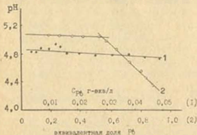
Рис.26. Изменение pH равновесных растворов (2) в зависимости от доли свинца в ШК чернозема выщелоченного (гор.В) по сравнению с значениями pH исходных растворов (1)
