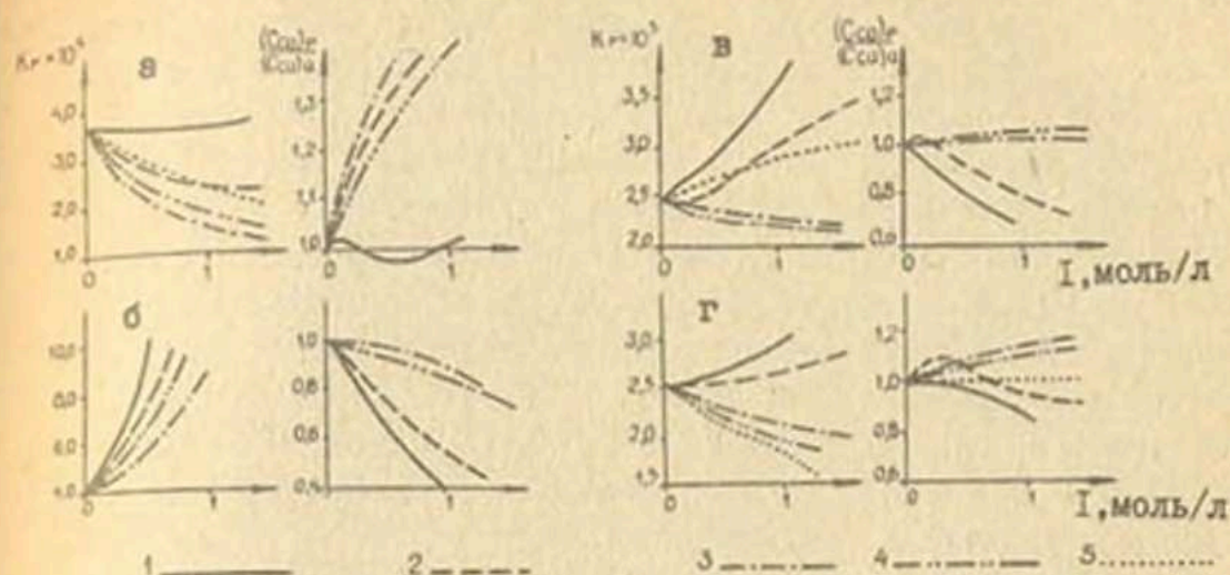
Рис. II. Результаты расчета произведений активности ионов \text{Ca}^{2+} и \text{SO}_4^{2-} ( K_T ) и концентрации кальция в насыщенных по гипсу растворах при 25^\circ / 43/ . Коэффициенты активности ионов вычислены: а) по (2.5) с \alpha^{\circ B} = I ; б) по (2.7) с \alpha^{\circ B} = I , \delta_i = 0, I z_i^2 ; в) при помощи варианта МИП с \delta_{\text{CaSO}_4}^{\circ} = I ; г) при помощи варианта МИП с \lg \delta_{\text{CaSO}_4}^{\circ} = -0,3 I_{\text{эф}} . Солевые системы: 1 - \text{Na}_2\text{SO}_4 - \text{CaSO}_4 - \text{H}_2\text{O} ; 2 - \text{MgSO}_4 - \text{CaSO}_4 - \text{H}_2\text{O} ; 3 - \text{NaCl} - \text{CaSO}_4 - \text{H}_2\text{O} ; 4 - \text{MgCl}_2 - \text{CaSO}_4 - \text{H}_2\text{O} ; 5 - \text{CaCl}_2 - \text{CaSO}_4 - \text{H}_2\text{O}
