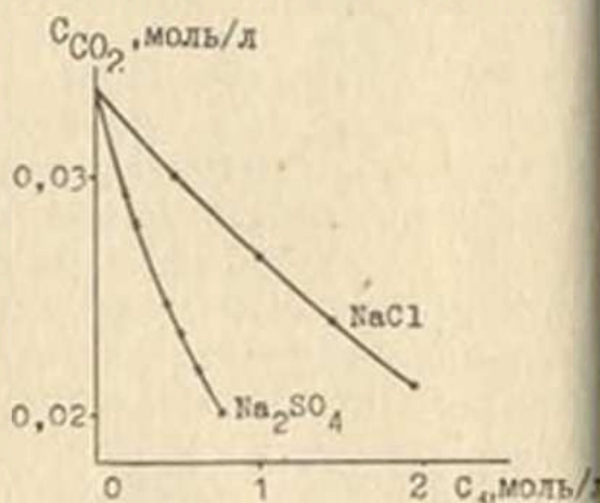
Рис.7. Растворимость \text{CO}_2 в водных растворах солей ( P_{\text{CO}_2} = 1 атм, t = 25^\circ ).
