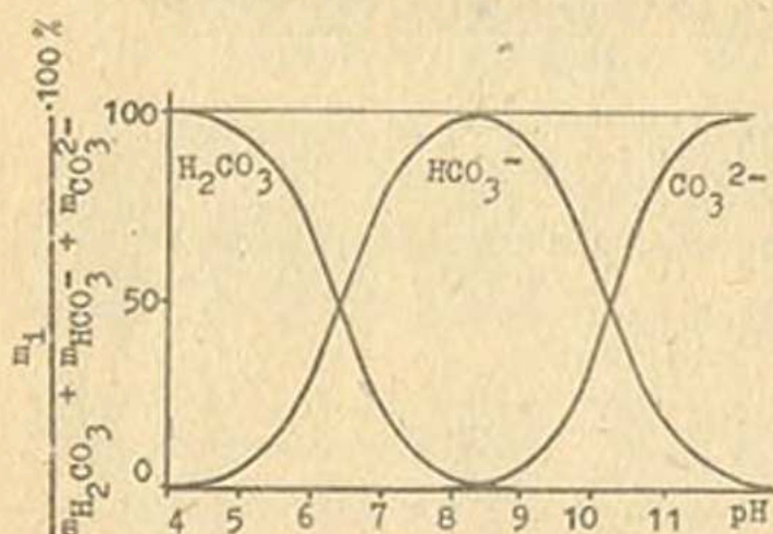
Рис. 8. Соотношение между концентрациями H_2CO_3 , HCO_3^- и CO_3^{2-} в воде при различных pH ( 25^\circ ).
