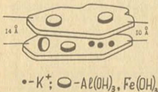
Рис. 18. Сорбция гидроксидов Fe и Al вермикулитом
