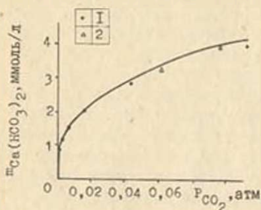
Рис. 13. Зависимость растворимости кальцита в воде при 25^\circ от парциального давления CO_2 в газовой фазе. Точки — экспериментальные данные /81/, кривая — расчет по (2.20) с вычислением коэффициентов активности ионов по (2.5) с \alpha^{\circ} = 1
