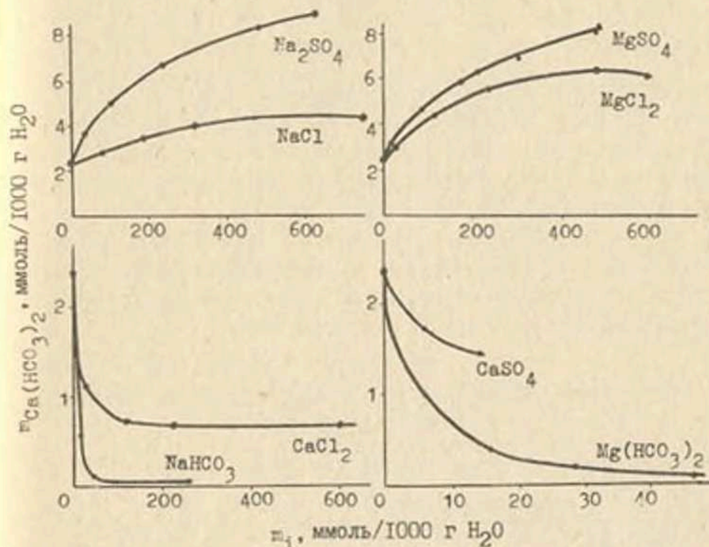
Рис. 14. Растворимость кальцита в водных растворах солей при 25^{\circ} и парциальном давлении \text{CO}_2 0,02 атм /62/.
