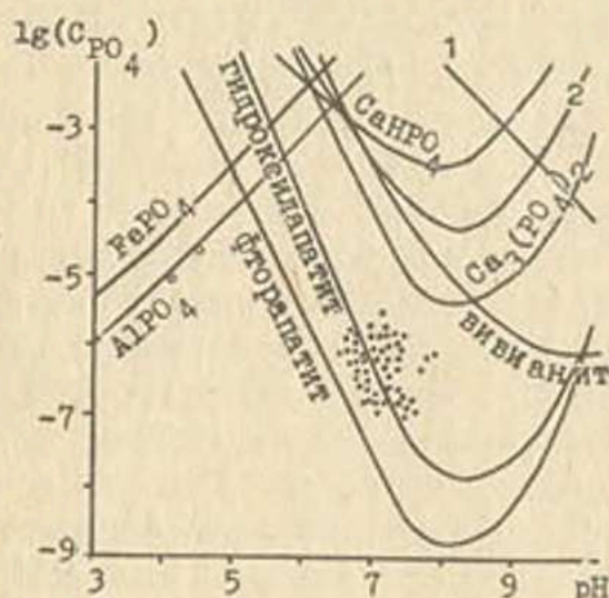
Рис. 15. Диаграмма растворимости присутствующих в почвах соединений фосфора (1 — кривая растворимости Mg_3(PO_4)_2 \cdot 22H_2O ; 2 — кривая растворимости Ca_4H(PO_4)_3 \cdot 2,5H_2O ) и концентрации фосфатов в некоторых дренажных водах (•) и промывных водах монолита (○)
