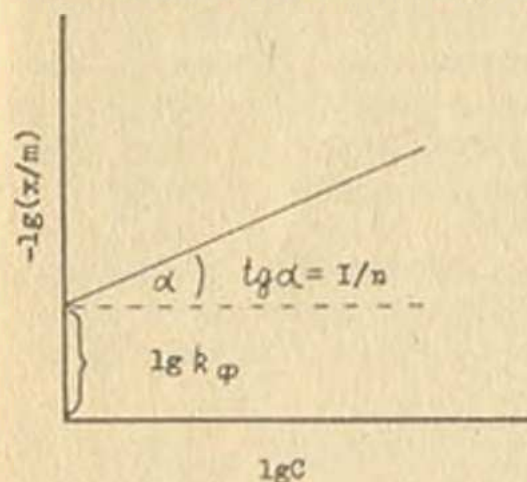
Рис. 19. Изотерма адсорбции Фрейндлиха в координатах уравнения (3.1)
