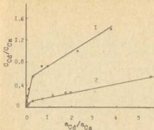
Рис.23. Изотермы ионного обмена \text{Ca}^{2+} - \text{Cd}^{2+} на Са-формах серой лесной почвы в координатах уравнения ЗДМ: 1 - гор. А (0-19 см), 2 - гор. В (19-31 см)
