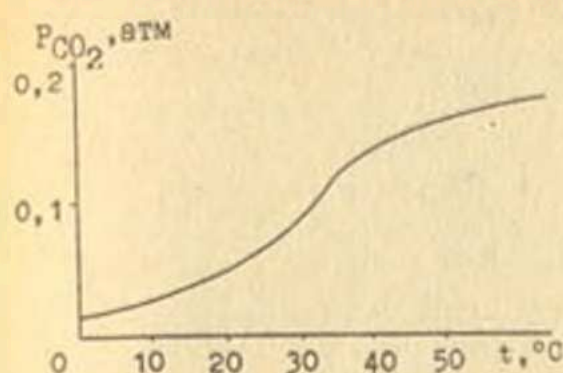
Рис. 4. Зависимость парциального давления \text{CO}_2 в почве от температуры /104/.
