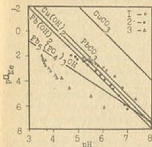
Рис. 27. Активности ионов \text{Cu}^{2+} и \text{Pb}^{2+} в равновесных суспензиях почв и кривые растворимости соединений этих элементов: 1 - лугово-черноземная карбонатная почва (Cu), 2 - чернозем типичный (Pb), 3 - серая лесная почва (Pb)
