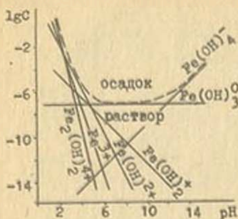
Рис. I6. Активность гидроко-м-п-лексов Fe (III) и его об-щая концентрация (---) в растворе
