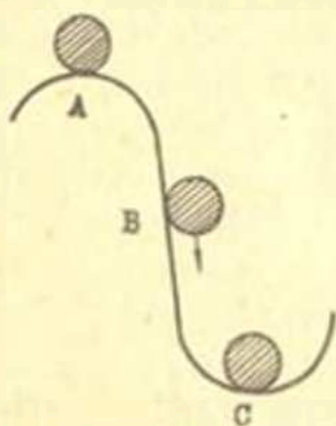
Рис. 2. Модель, иллюстрирующая равновесие в механической системе.
