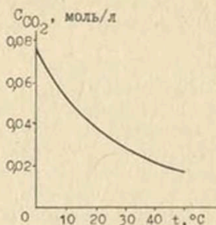
Рис.6. Зависимость растворимости \text{CO}_2 в воде от температуры при P_{\text{CO}_2} = 1 атм.
