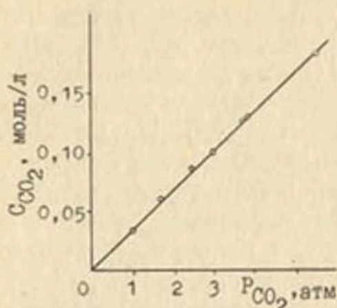
Рис.5. Зависимость растворимости \text{CO}_2 в воде от его парциального давления в газовой фазе при 25^\circ . Точки — экспериментальные данные; прямая — расчет по уравнению (2.II).
