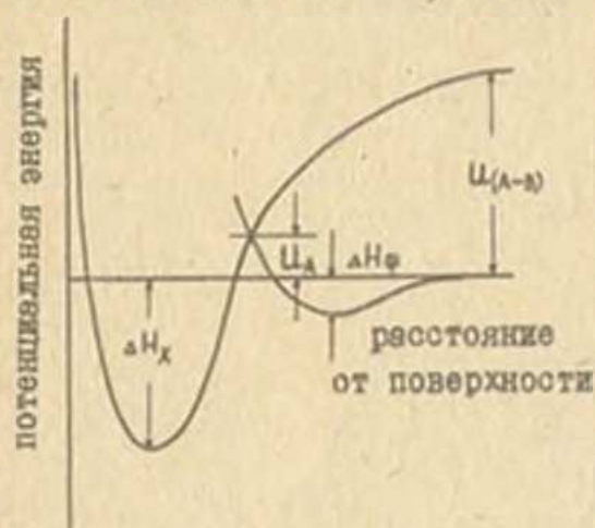
Рис. 22. Профиль потенциальной энергии адсорбции: H_A — энтальпия физической адсорбции, H_X — энтальпия хемосорбции, u_A — энергия активации хемосорбции, u_{A-B} — энергия возбужденной молекулы
