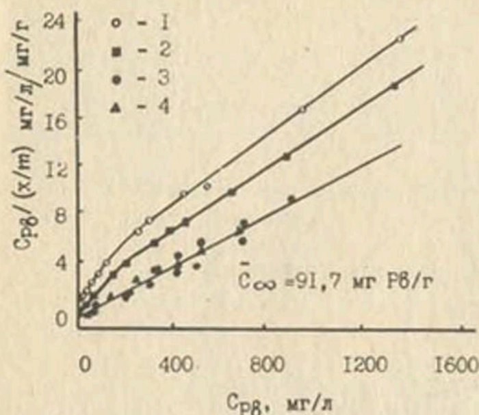
Рис.20. Изотерма адсорбции свинца Са-монтморионитом в координатах уравнения Лэнгмюра (3.8) при соотношениях твердой и жидкой фаз: 1-1:50, 2-1:100, 3-1:500, 4-1:1000 /II2/
