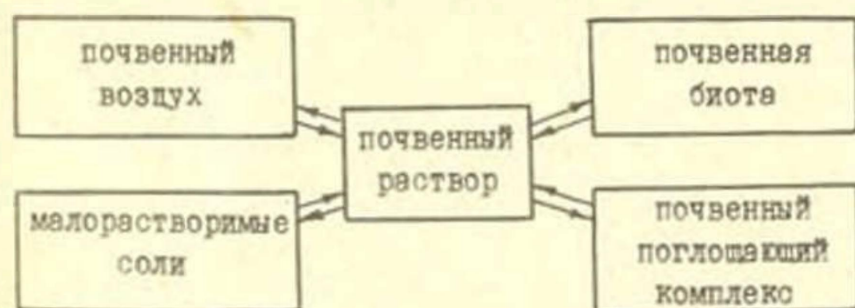
Рис. I. Блок-схема взаимодействия составляющих почвы
