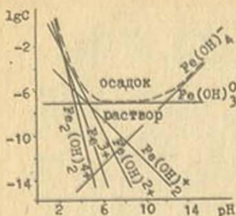
Рис.16. Активность гидроко-м-п-лексов Fe (III) и его об-щая концентрация (---) в растворе
