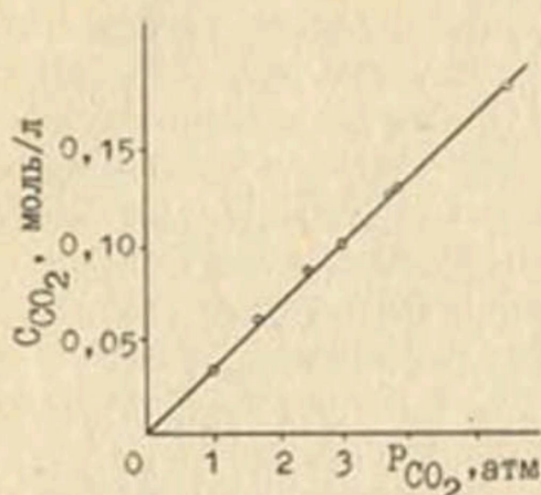
Рис. 5. Зависимость растворимости \text{CO}_2 в воде от его парциального давления в газовой фазе при 25^\circ . Точки — экспериментальные данные; прямая — расчет по уравнению (2.11).
