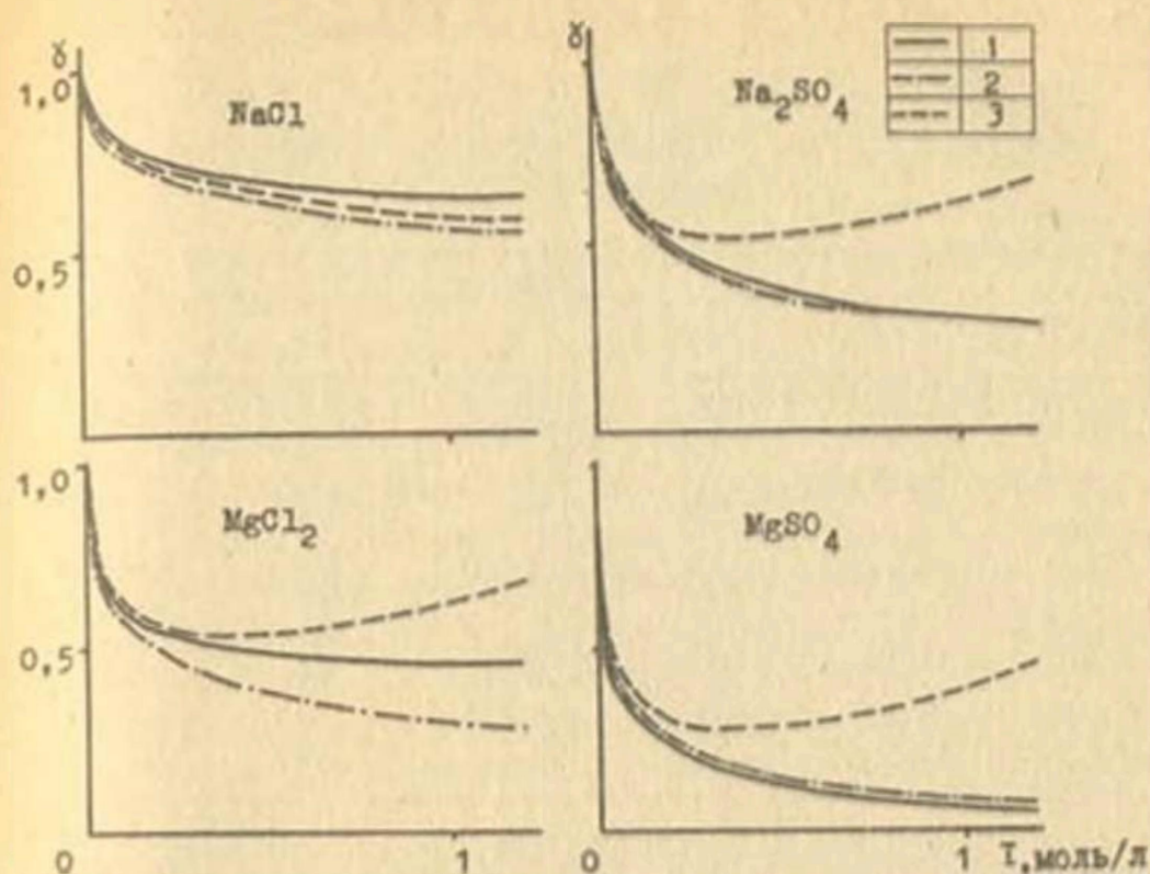
Рис. 3. Зависимость средних ионных коэффициентов активности солей от ионной силы раствора: 1 — экспериментальные данные; 2 — расчет по уравнению Гиттельберга; 3 — расчет по уравнению Дейвиса (2.8).
