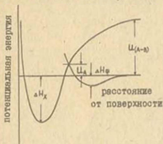
Рис. 22. Профиль потенциальной энергии адсорбции: \Delta H_A — энтальпия физической адсорбции, \Delta H_X — энтальпия хемосорбции, U_A — энергия активации хемосорбции, U_{A-B} — энергия возбужденной молекулы
