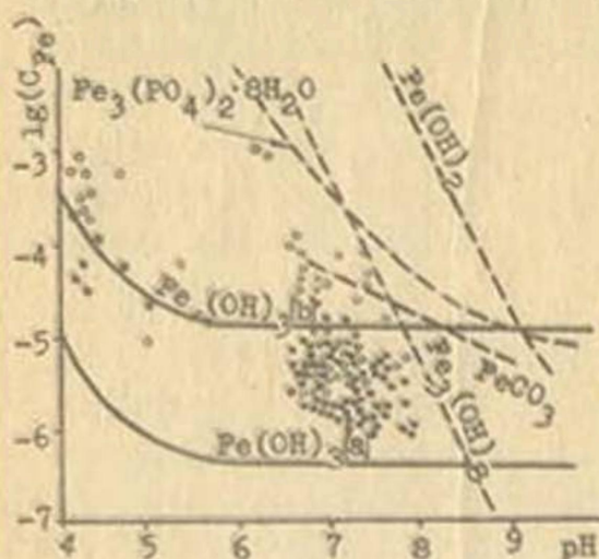
Рис.17. Диаграмма растворимости присутствующих в почвах соединений железа ((а) — Fe(OH)_3 при pK = 37,5 ; (б) — Fe(OH)_3 при pK = 35,96 ) и концентрации Fe (III) (*) и Fe (II) в некоторых дренажных водах
