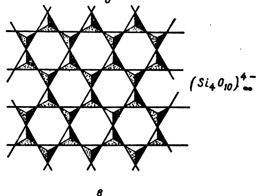
Рис. 1.2. Кремнекислородные радикалы:
