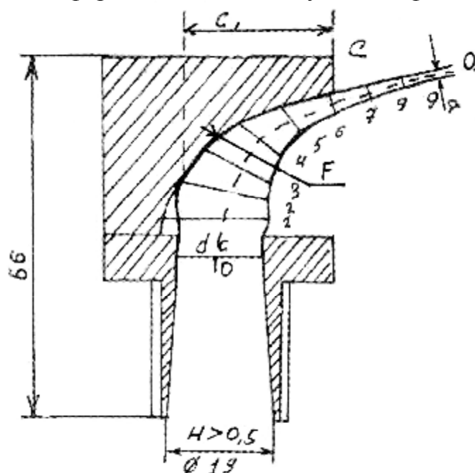
Рис. 7. Форма потока воды по секторному насадку
