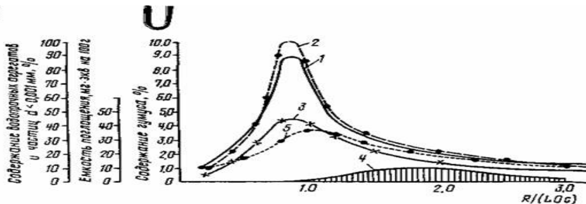
Рис. 22. Зависимость основных свойств почвы от гидротермического режима (по И. П. Айдарову):
