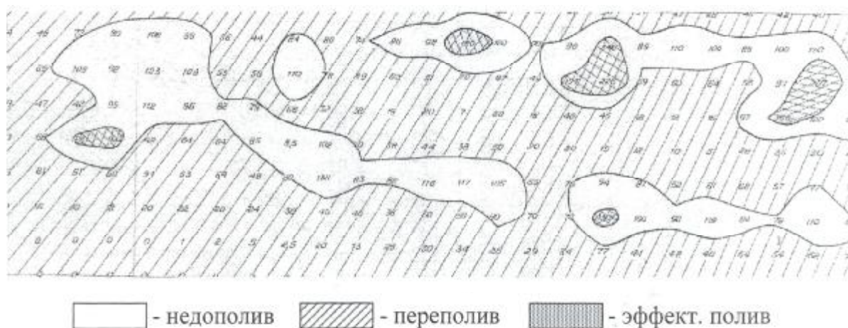
Рис. 17. Карта распределения искусственного дождя дождевальной машины ДКФ-1ПК – при рабочей высоте консоли 2 м
