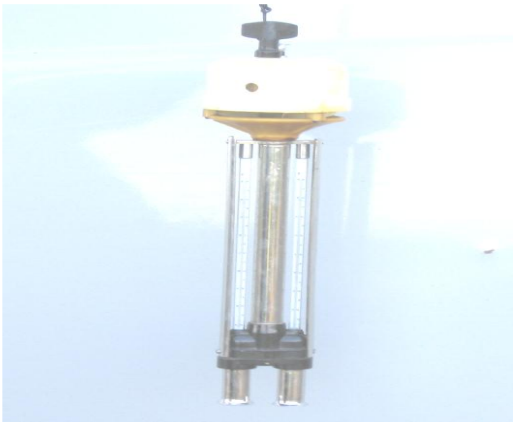
Рис. 16. Психрометр
