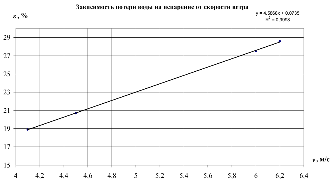
Рис. 19. Зависимость потерь воды на испарение от скорости ветра
