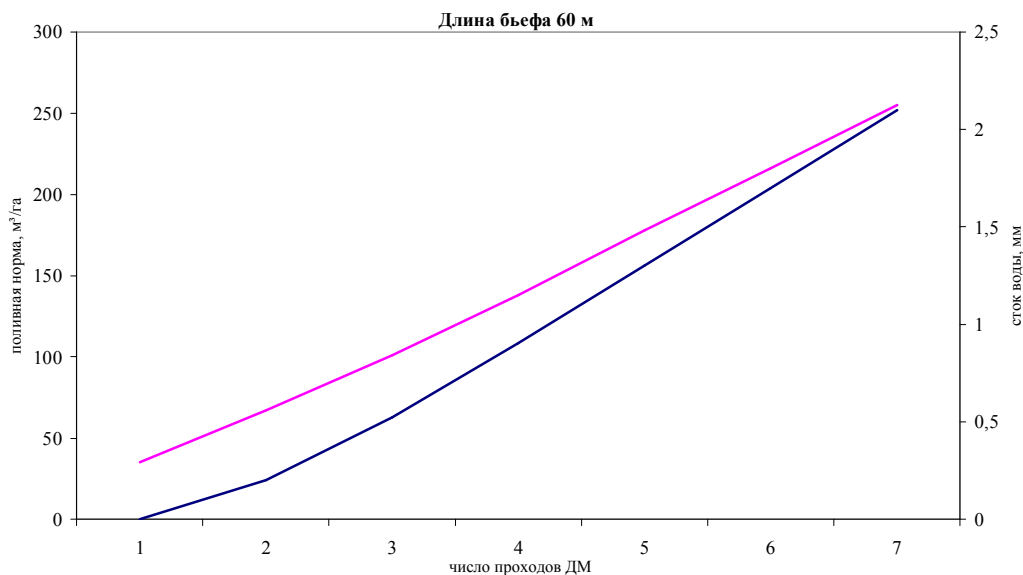
Рис. 20. Зависимость выдачи поливной нормы при длине бьефа 60 м
