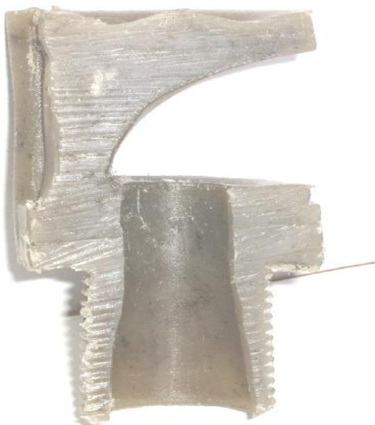
Рис. 6. Секторный насадок в разрезе
