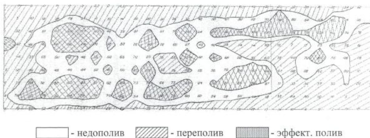
Рис. 18. Карта распределения искусственного дождя дождевальной машины ДКФ-1ПК – с понижением консоли на 0,5 м
