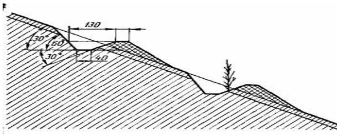
Рис. 23. Схема траншейных террас
