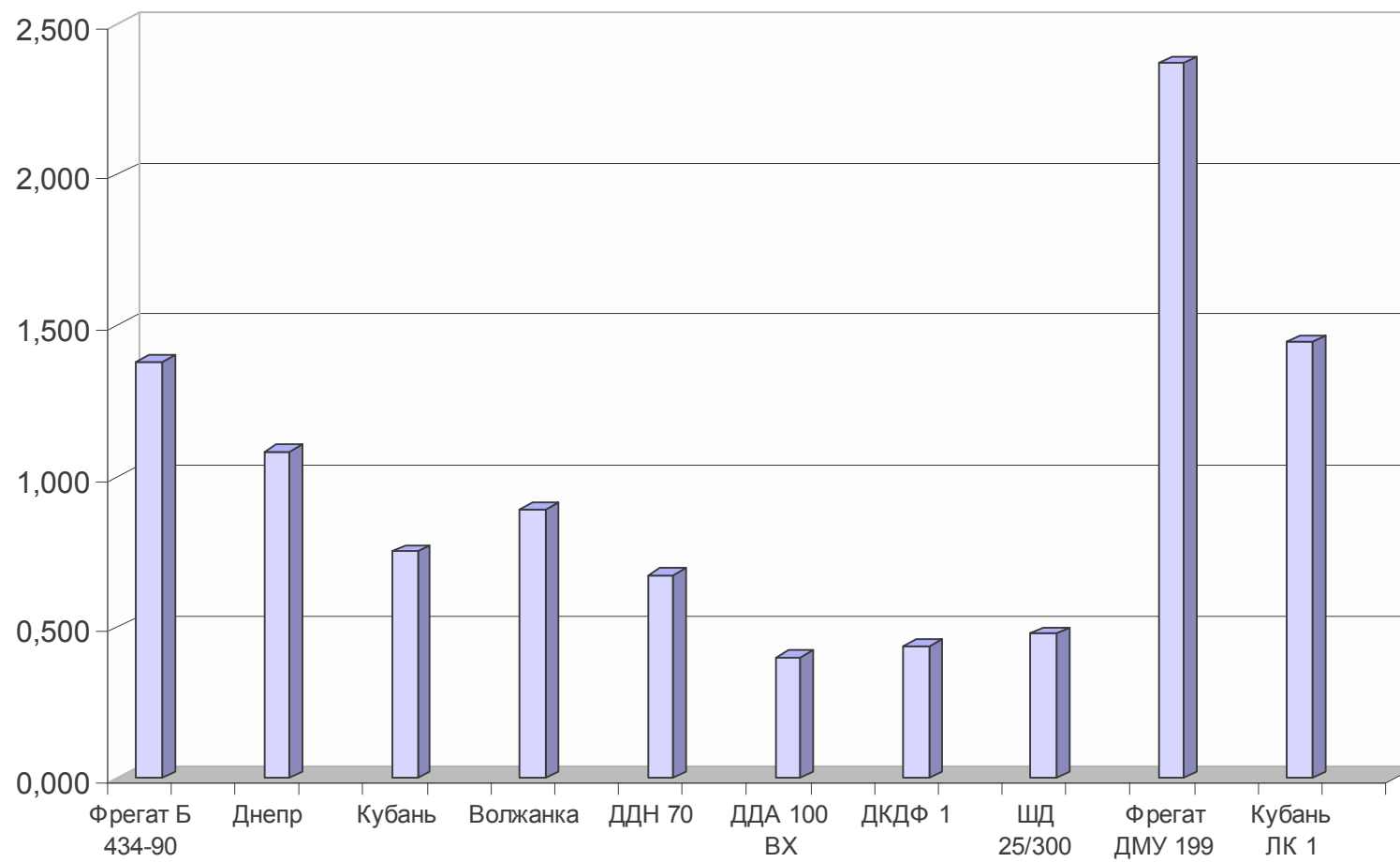
Рис. 1. График относительных показателей серийных дождевальных машин
