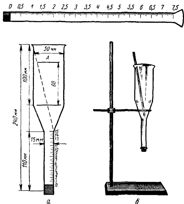
Рис. 14. Воронка М. М. Филатова для механического анализа почвы (размеры в мм)
