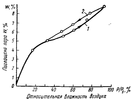
Рис. 54. Типичная изотерма адсорбции и десорбции водяных паров почвами:
