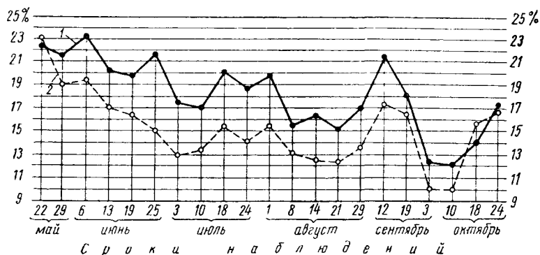
Рис. 72. Влажность дерново-подзолистой суглинистой почвы на раннем паре в % сухой почвы. Собакино опытное Московской области. Вершина склона, 1924:
