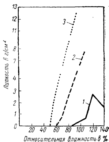
Рис. 73. Липкость дерново-подзолистой суглинистой пылевато-песчаной почвы в зависимости от оструктуренности, распыленности и влажности в г/см², Ап, стерня ржи:
