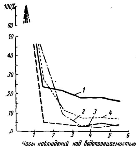
Рис. 71. Водопроницаемость и водопрочность агрегатов дерново-подзолистой суглинистой почвы из гор. А 1 в %. Московская обл., колхоз «Красноармеец». Метод определения Фадеева — Вильямса:
