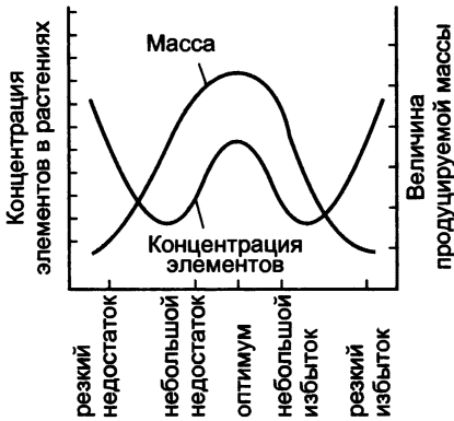
Рис. 9. Изменение продуцируемой массы в зависимости от концентрации элементов в растениях (Ринькис, 1972)
