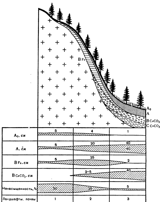
Рис. 24. Почвенно-геохимическое сопряжение в поясе еловых лесов Центрального Тянь-Шаня (По Глазовой, 1968):
