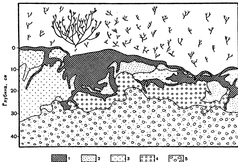
Рис. 56. Крйотурбация в арктикотундровых почвах. Гренландия (по Уголини, 1966):
