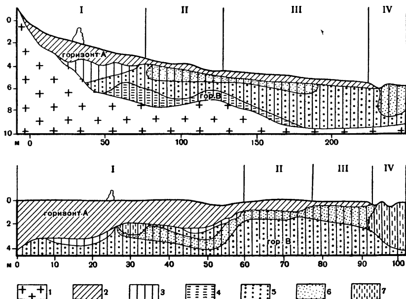
Рис. 62. Почвенно-геохимическая катена в бассейне оз. Чад (по Бокье, 1970).
