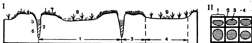
Рис. 30. Микрорельеф хорошо развитого крупнопolygonального болотно-го ландшафта Яно-Инди́гирской низменности:
