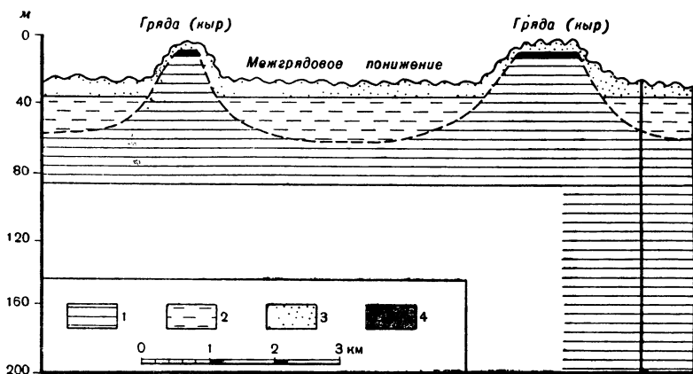
Рис. 52. Условия залегания ископаемых почв на останках (кырах) плиоценовой аллювиальной равнины (Юго-Восточные Каракумы): 1 — заунгузская свита, 2 — древний аллювий Пра-Амударьи; 3 — золотые пески; 4 — ископаемая почва
