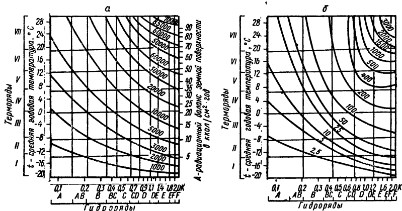
Рис. 2. Затраты энергии в почвообразовании (ккал/см 2 ·год): а — суммарные затраты энергии в биогеоценозе на почвообразование; б — запасы энергии, накапливаемые в годичном приросте растительной массы, надземной и корневой (по В. Р. Волобуеву, 1963)
