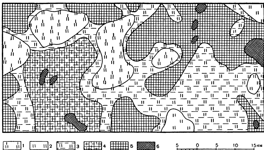
Рис. 51. План лугово-степного комплекса с суффозионным микрорельефом в Прикаспии (по Е. Н. Ивановой и др.):
