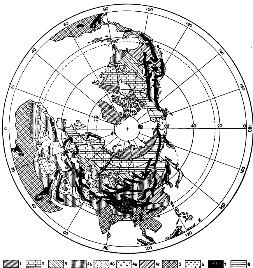
Рис. 1. Почвенные зоны Северного полушария (схема) (В. В. Докучаев, 1899): 1 — бореальная (арктическая); 2 — лесная; 3 — черноземных степей; 4 — азральная (а — каменистая, б — песчаная, в — солончаковая, г — лёссовая); 5 — латеритные почвы; 6 — аллювий; 7 — горные цепи; 8 — облесенные территории
