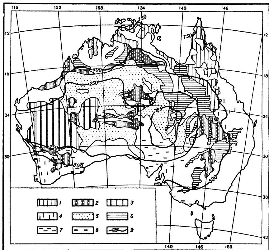
Рис. 64. Ландшафтно-геохимические реликты Австралии. Реликты древних элювиальных и суперкальвальных влажнотропических ландшафтов. Области распространения древней каолинит-гематитовой (латеритной) коры выветривания:
