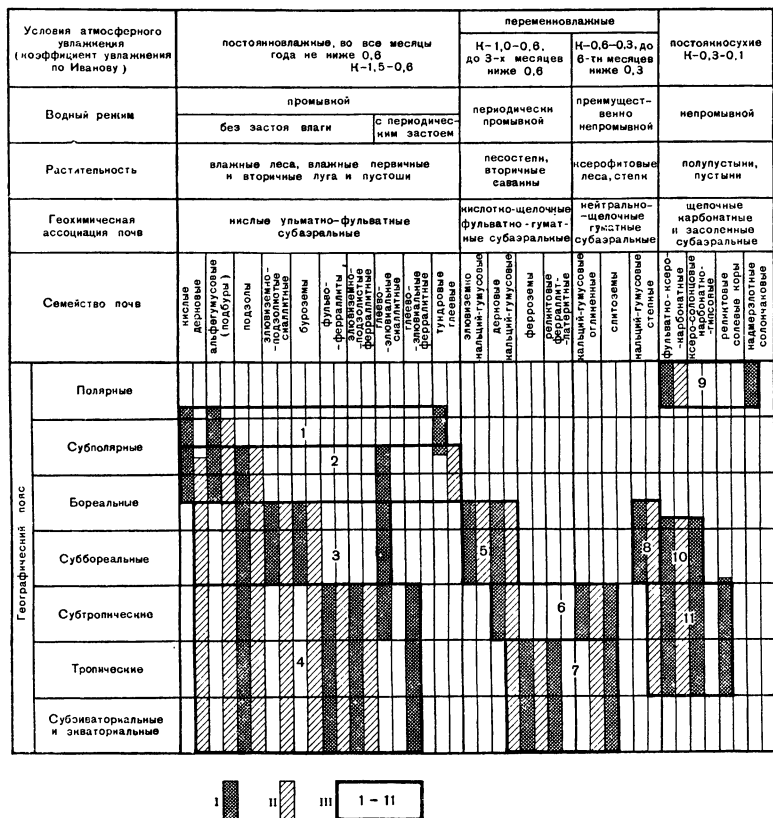
Распространение геохимических ассоциаций и семейств субэвразальных почв по географическим поясам и зонам увлажнения (на равнинах)
