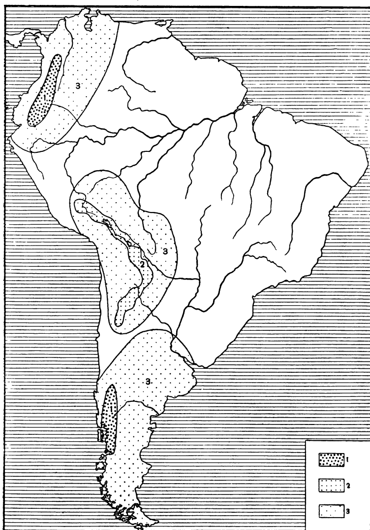
Рис. 59. Распространение вулканических пеплов в Южной Америке: 1 — ландшафты с выветрелым вулканическим пеплом; 2 — ландшафты с невыветрелым пеплом; 3 — ландшафты со слабыми пеплопадами
