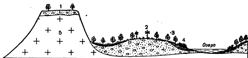
Рис. 33. Распределение почв по элементам мезорельефа в предтундровых редколесьях Северной Лапландии (по М. А. Глазовской, 1964):
