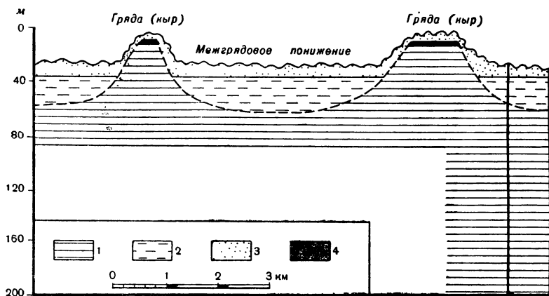
Рис. 52. Условия залегания ископаемых почв на останцах (кырах) плиоценовой аллювиальной равнины (Юго-Восточные Каракумы): 1 — заунгузская свита, 2 — древний аллювий Пра-Амударьи; 3 — золотые пески; 4 — ископаемая почва
