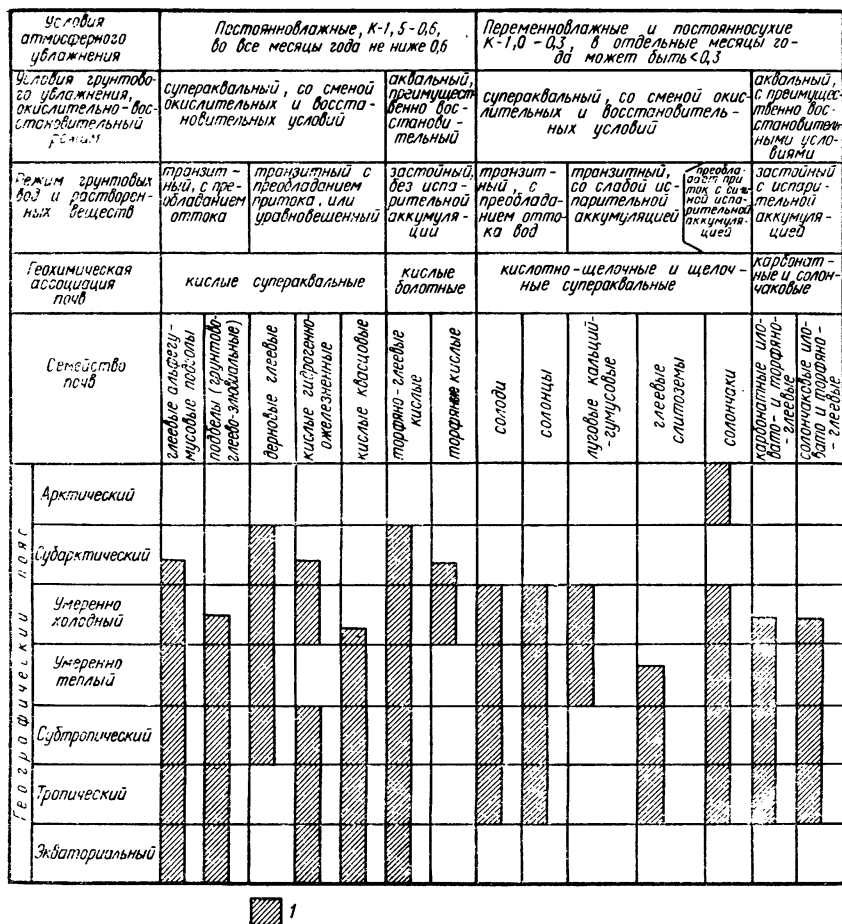
Рис. 8. Распространение геохимических ассоциаций супераквальных почв по географическим поясам и зонам увлажнения. 1 — ареалы семейств почв
