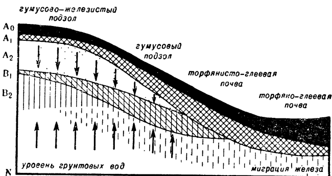
Рис. 37. Почвенная катена на склоне песчаного холма при близком стоянии грунтовых вод в ландах в Гасконии (по Дюшофуру, 1948)
