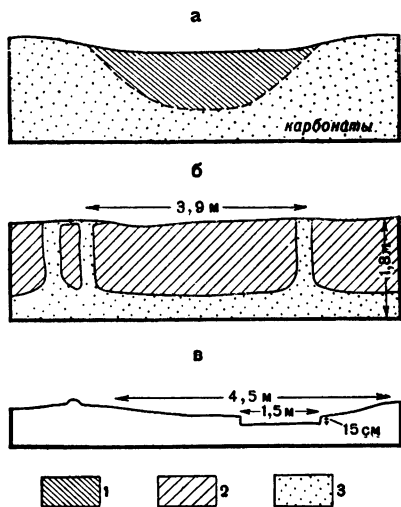
Рис. 66. Разрезы через комплексы «гильгаи»:
