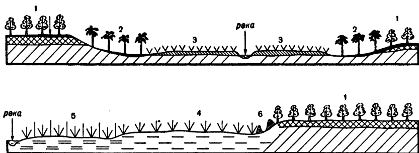
Рис. 63. Схема распределения почв и растительности по рельефу в Замбии (по М. Коул, 1963):
