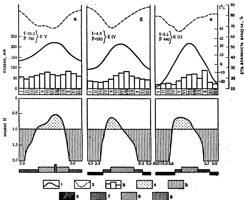
Рис. 36. Гидротермические условия в районах распространения: а — бурых лесных почв Западной и Восточной Европы; б — дерново-подзолистых почв Восточной Европы; в — Западной Сибири (по В. Р. Волобуеву, 1963); 1 — среднемесячная температура; 2 — отн. влажность воздуха; 3 — среднемесячная сумма осадков; 4 — K < 1 ; 5 — K > 1 ; 6 — температура воздуха ниже 0^{\circ}\text{C} ; 7 — от 0^{\circ}\text{C} до 10^{\circ}\text{C} ; 8 — от 10 до 20^{\circ}\text{C} ; 9 — от 20 до 30^{\circ}\text{C}
