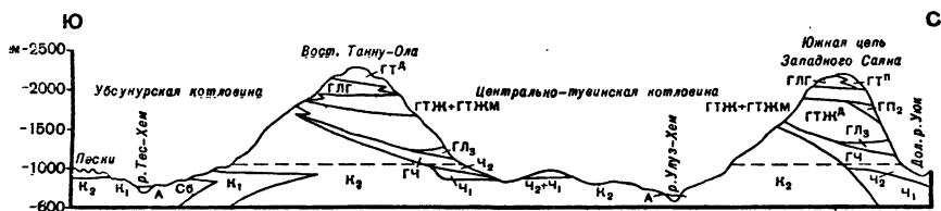
Рис. 49. Структура почвенного покрова в связи с рельефом по основным природным частям Тувы (по В. А. Носику):
