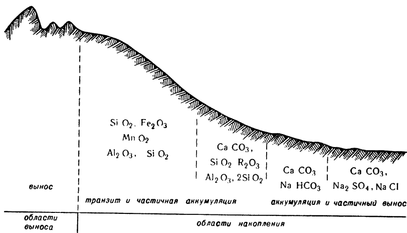
Рис. 48. Схема распространения продуктов выветривания и почвообразования в Маньчжурии и Монголии (по В. А. Ковде, 1959)
