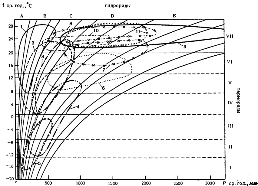
Рис. 11. Климатические ареалы основных почвенных типов мира в гидротермической системе координат (по В. Р. Волобуеву, 1963):
