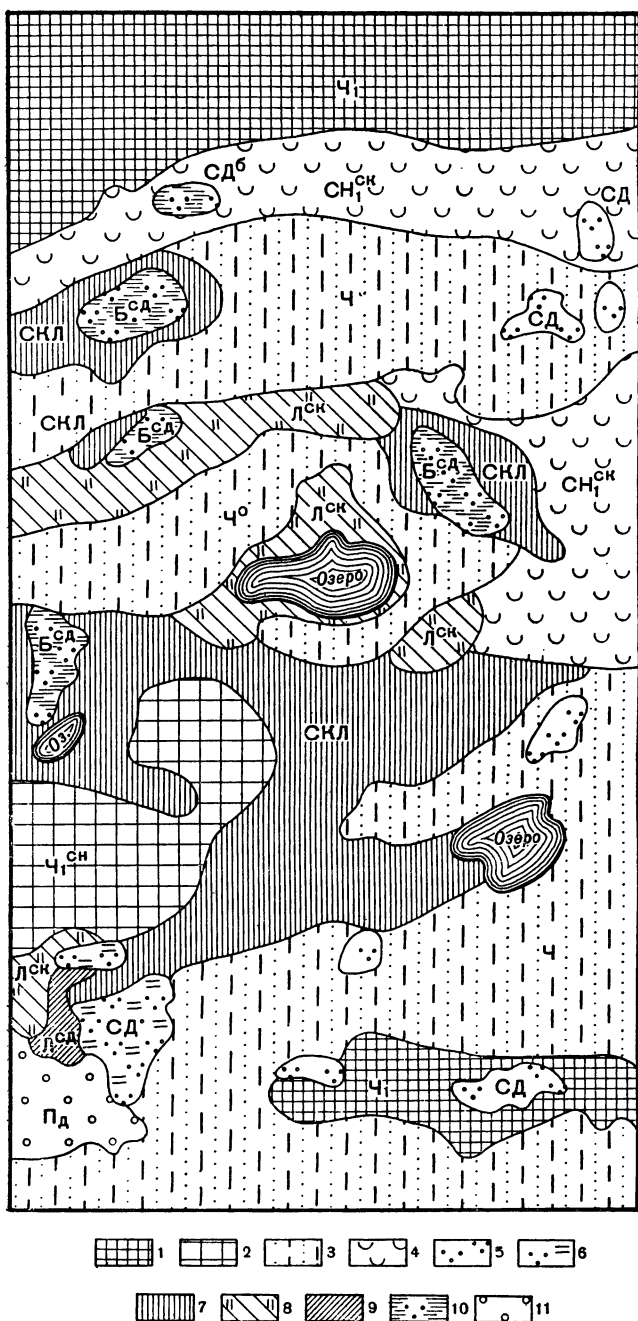
Рис. 50. Сочетания и комплексы почв в черноземной зоне Алтайского края («Почвы Алтайского края», 1959):
