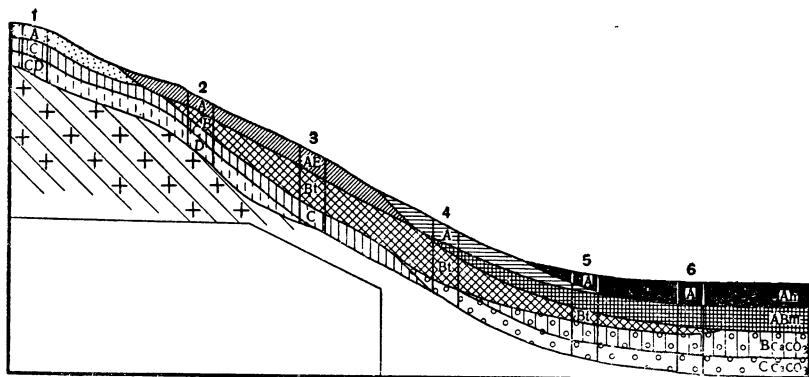
Рис. 42. Распределение почв по рельефу Гранитного массива в Болгарии (по В. Койнову и др., 1969):
