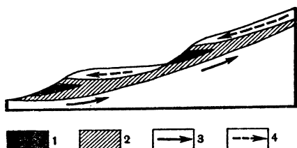
Рис. 60. Схема процесса денудации лесных почв на склонах после порубки лесов (Оберу и Миньену):
