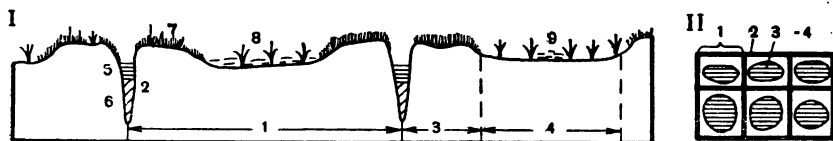
Рис. 30. Микрорельеф хорошо развитого крупнопolygonального болотно-го ландшафта Яно-Инди́гирской низменности:
