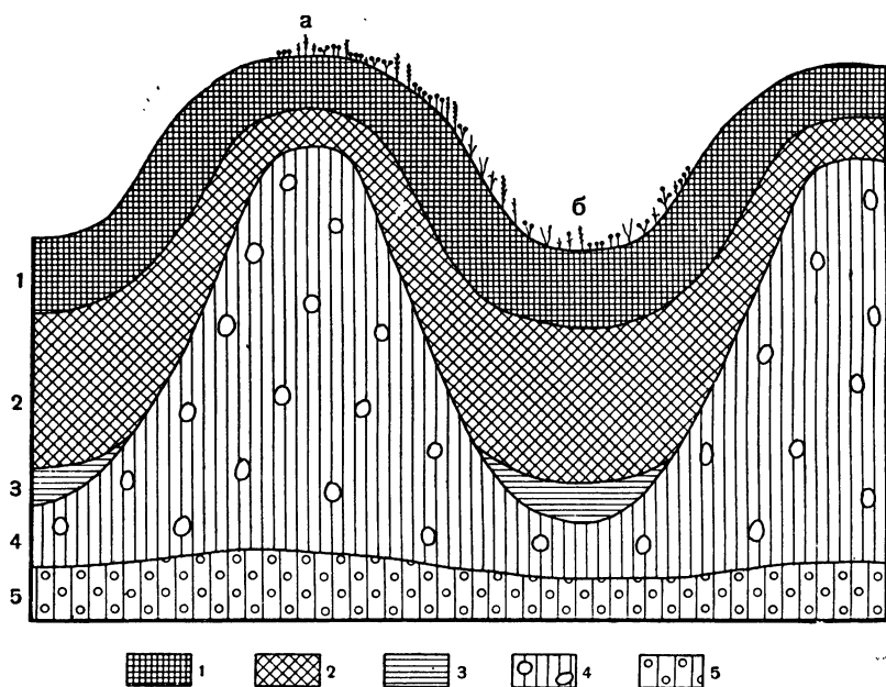
Рис. 32. Схема почвенного комплекса в ложине на п-ове Пьятина (по Е. Н. Наумову, 1965):
