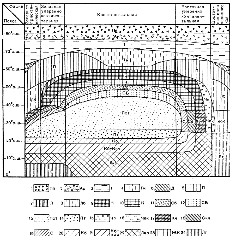
Рис. 12. Схема горизонтальных почвенных зон северного полушария на «идеальном континенте».
