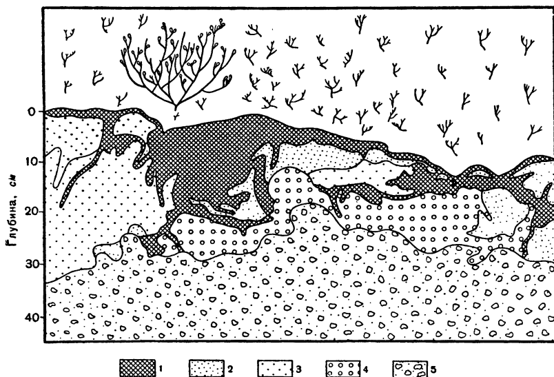
Рис. 56. Криотурбация в арктикотундровых почвах. Гренландия (по Уголини, 1966):
