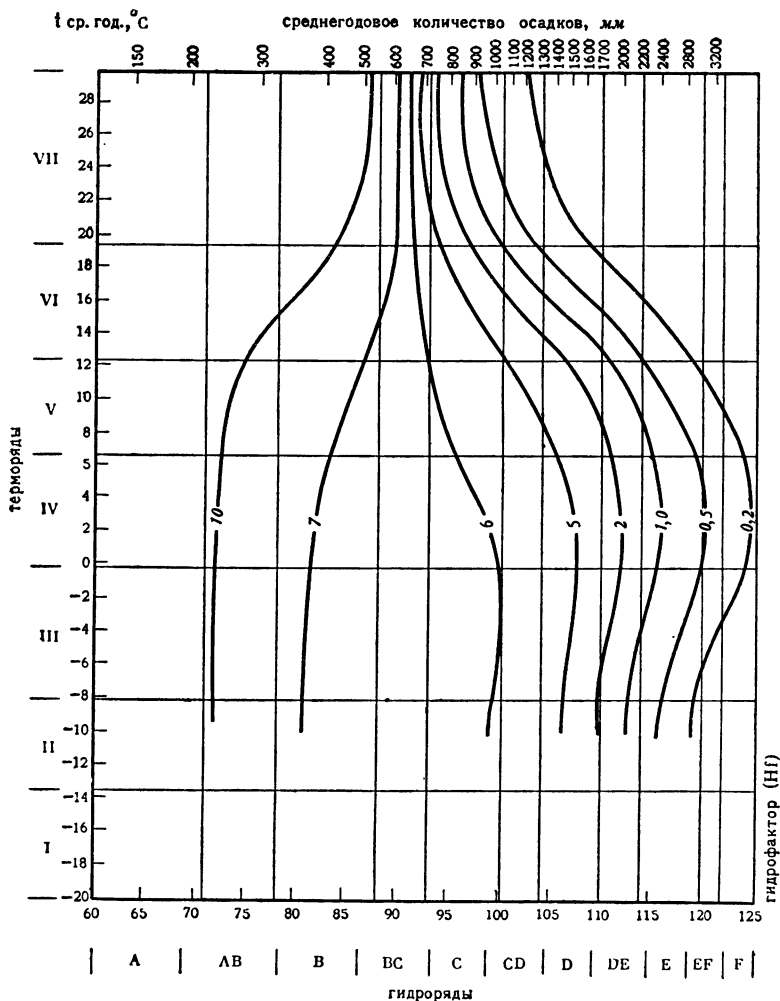
Рис. 6. Содержание карбонатов (% CO 2 ) в верхнем метровом слое почв в связи с гидротермическими условиями (по В. Р. Волобуеву, 1963)
