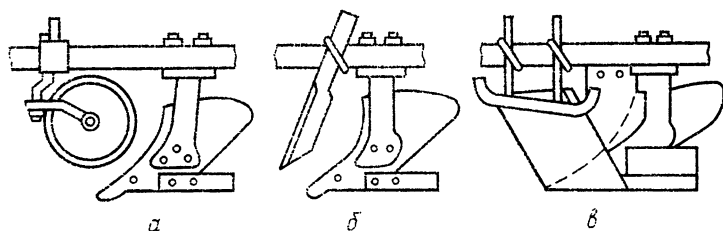
Рис. 13. Ножи плугов.
