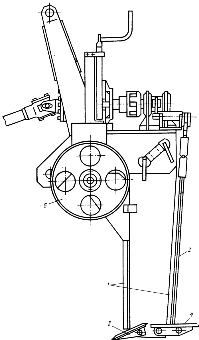
Рис. 32. Виброрыхлитель.
