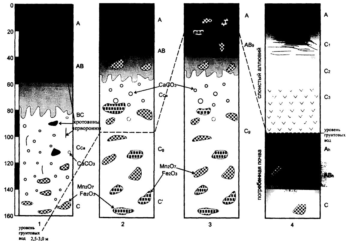
Рис. 18. Строение гидроморфных почв:
