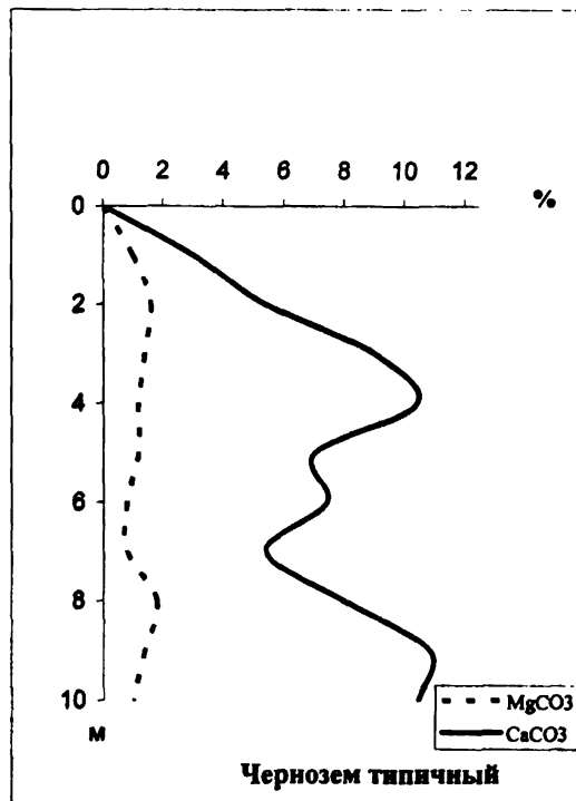
Рис. 12. Карбонатный профиль черноземов Предкавказья в 10-метровом слое (Валяков, Токосов)
