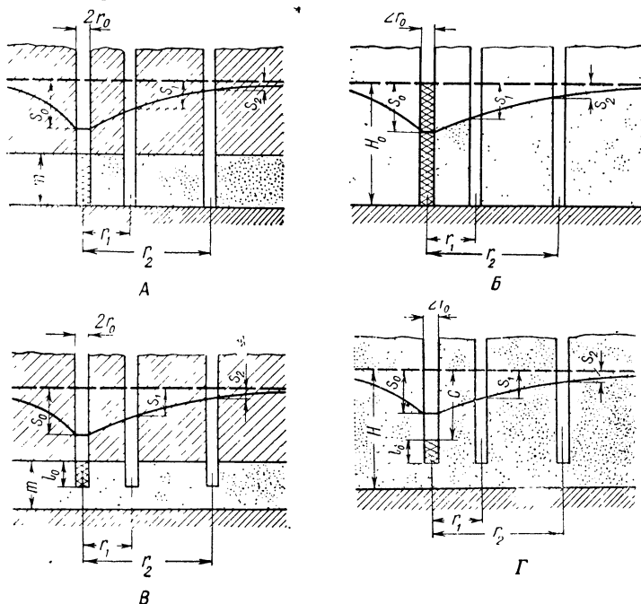
Рис. 24. Схема определения коэффициента фильтрации грунта методом откачек.
