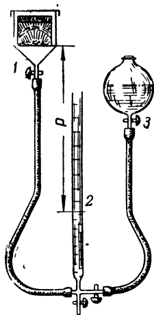
Рис 10 Капилляриметр Фишера
