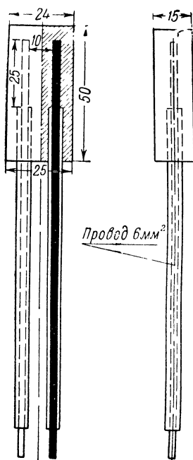
Рис. 5. Схема гипсового блока.
