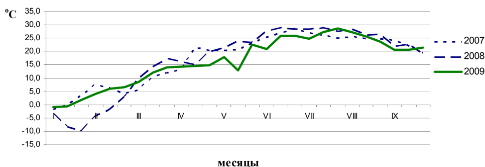
График 5.2 Температура воздуха
